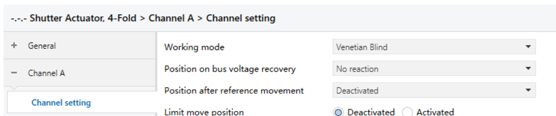
Fig.5.3 parameter window "Channel X"
