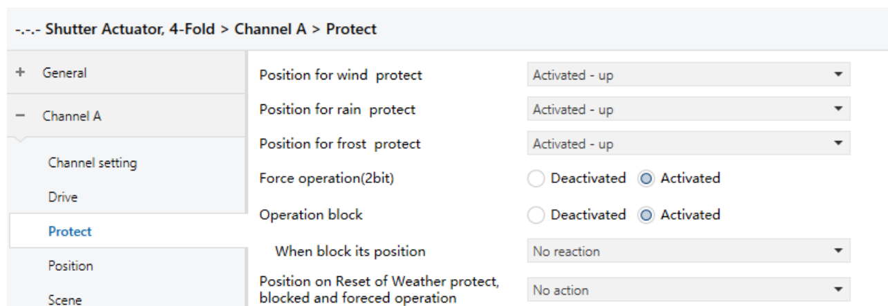
Fig.5.5 parameter window "Protect"
