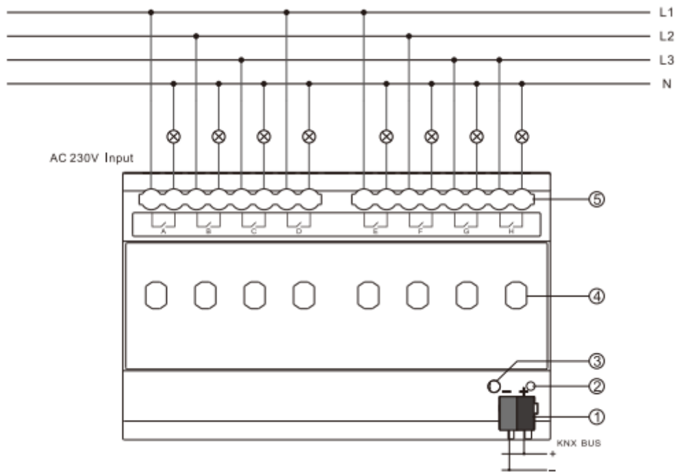
Fig.3.2(2)ARCD-08/16.S
