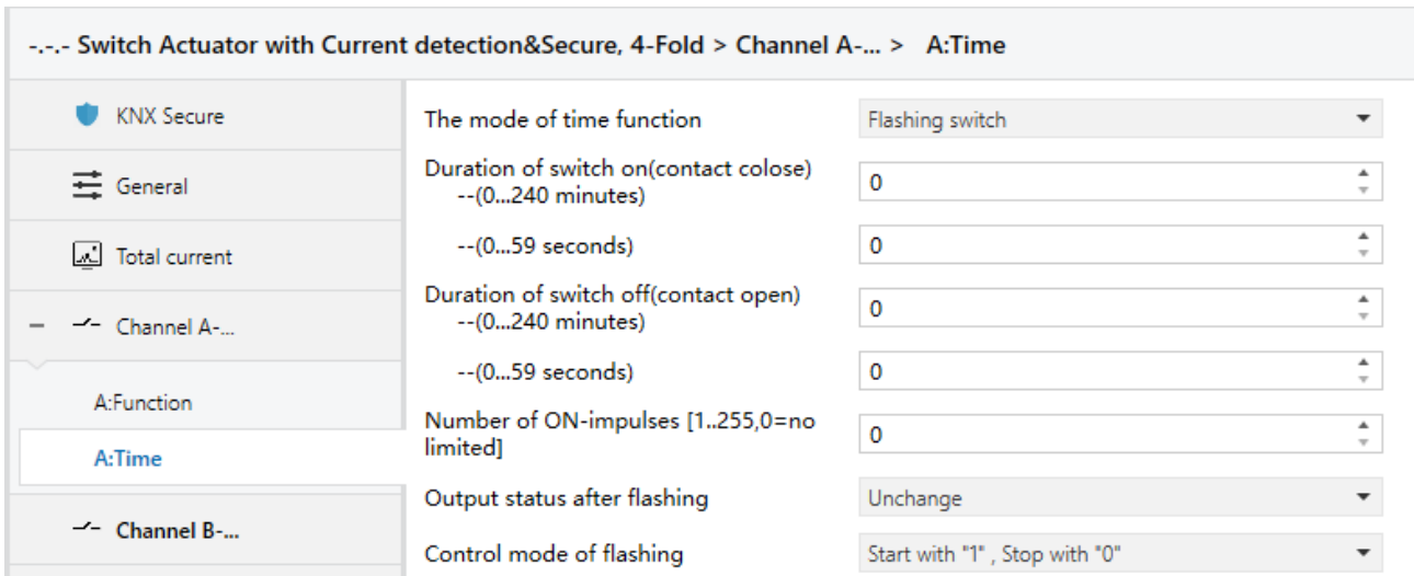
Fig. 4.4.1.2 Parameter window "X: Time"-Flashing switch
