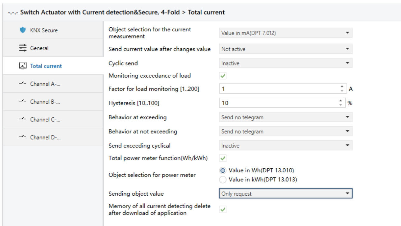
Fig. 4.3.1 Parameter window “Total current”
