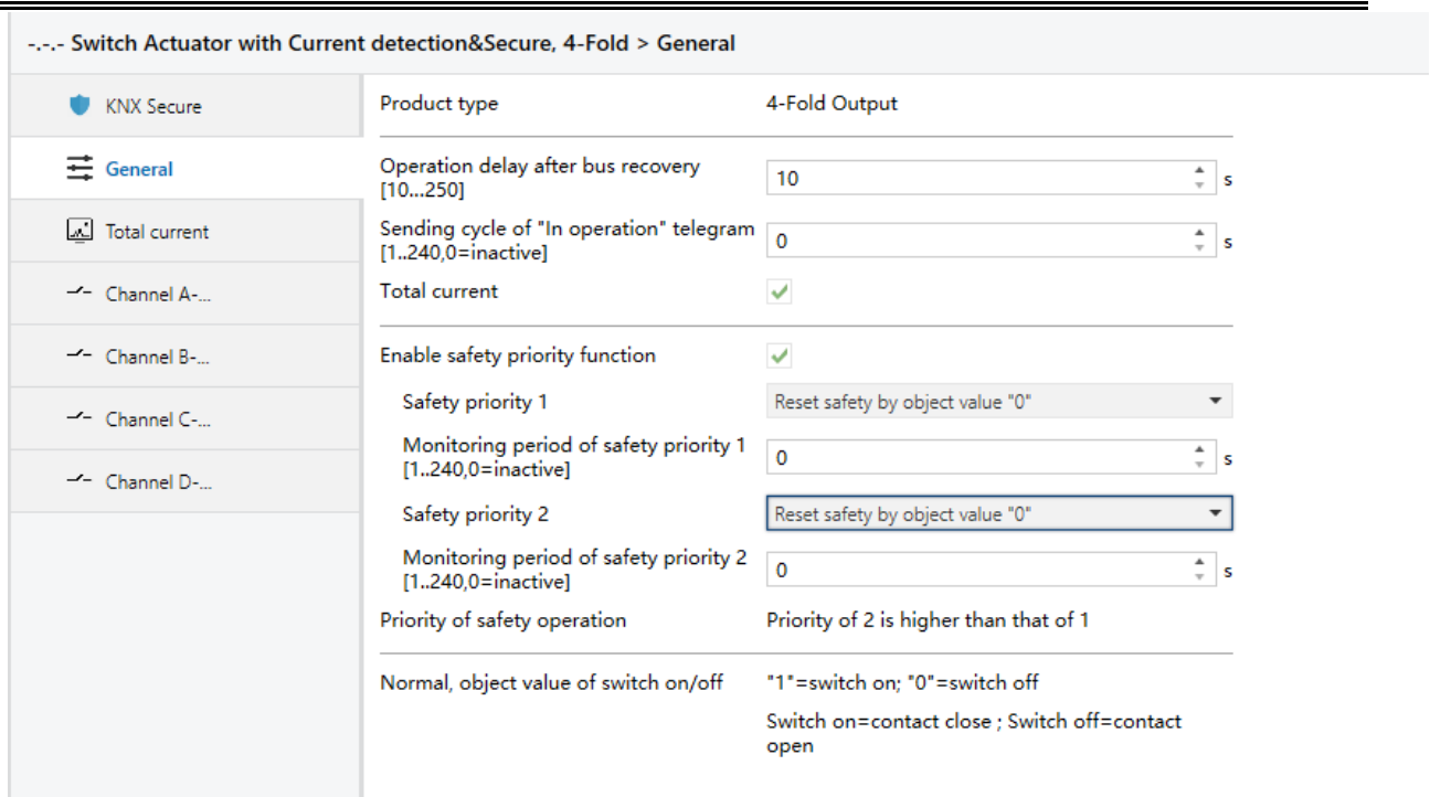
Fig. 4.3 Parameter window "General"
