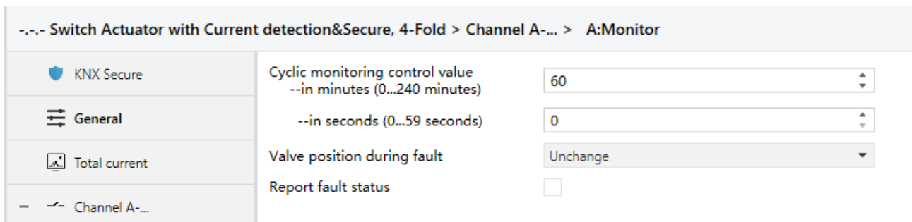
Fig. 4.5.1 Parameter window "X: Monitor"
