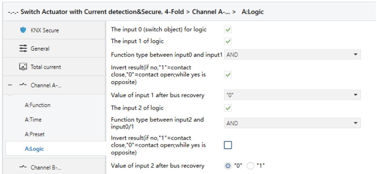
Fig. 4.4.3 Parameter window “X: Logic”
