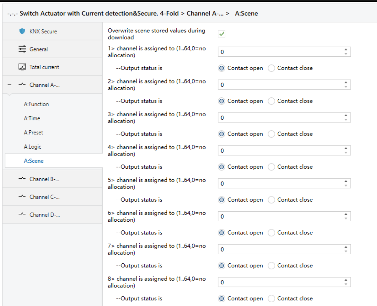
Fig. 4.4.4 Parameter window "X: Scene"
