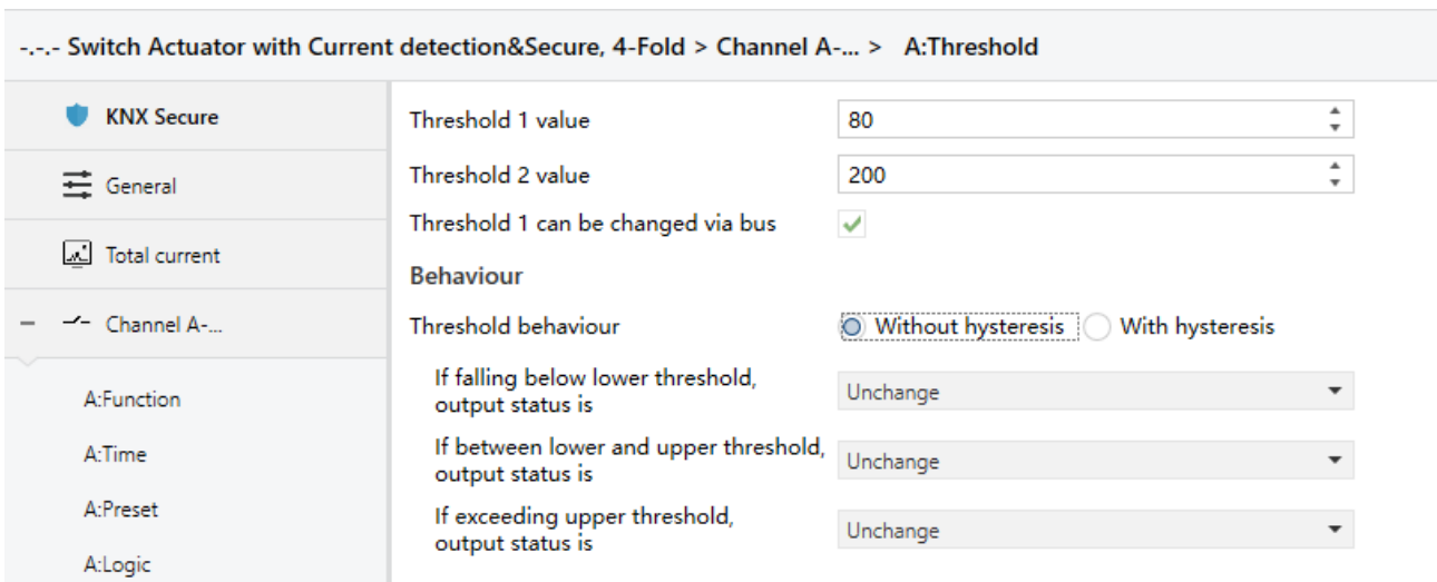
Fig. 4.4.5 Parameter window "X: Threshold"
