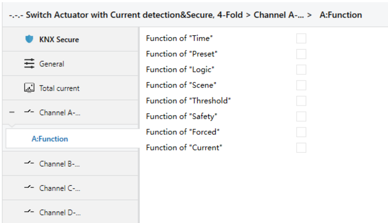
Fig. 4.4(3) Starting parameter window “X: Function”
