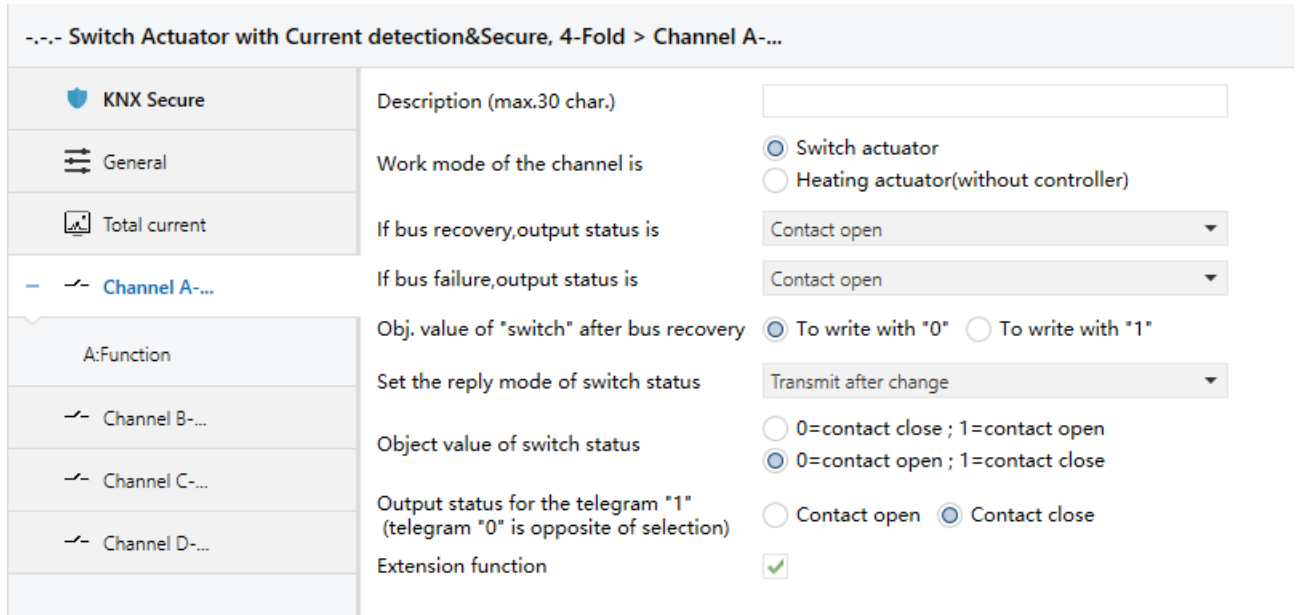
Fig. 4.4(2) Starting parameter window “X: Function”
