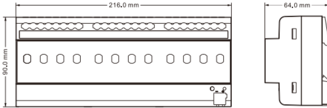
Fig.3.1(3)ARCD-12/16.S
