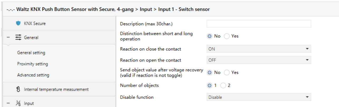
Fig.5.4.2(1) Parameter setting of switch sensor
