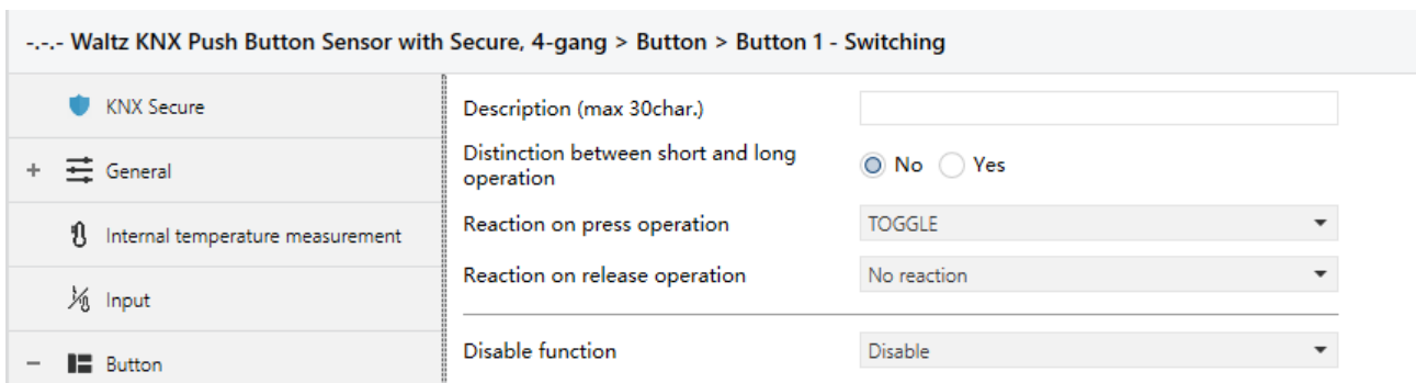
Fig.5.5.1 Parameter setting of switch function
