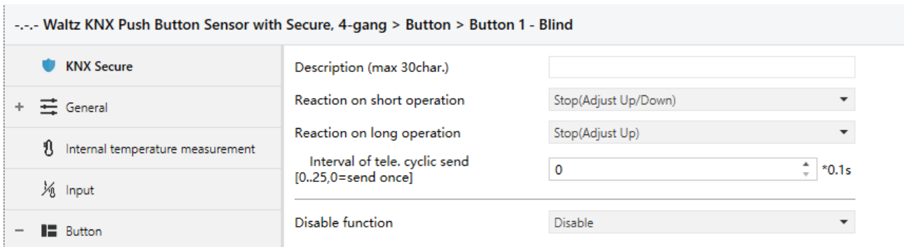
Fig.5.5.8 Parameter setting of blind function
