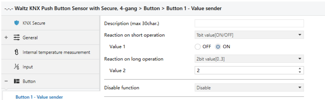
Fig.5.5.6 Parameter setting of value sender
