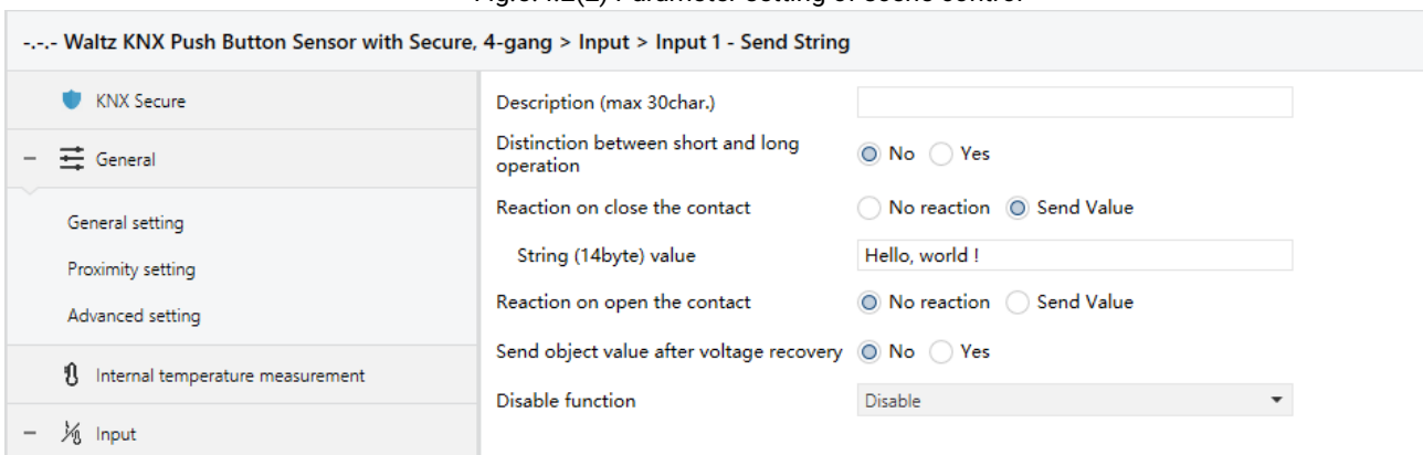
Fig.5.4.2(3) Parameter setting of sending string
