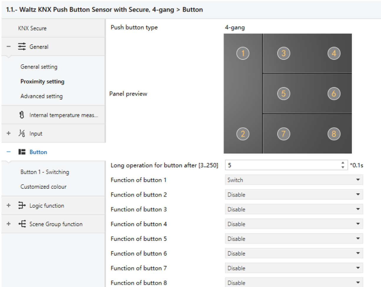
Fig.5.5“Button” parameter window
