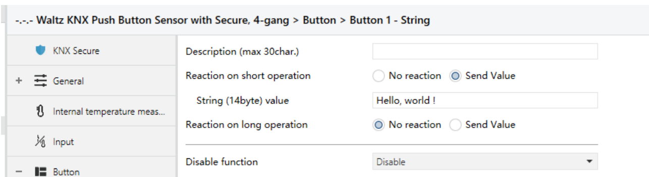
Fig.5.5.13 Parameter setting of string function
