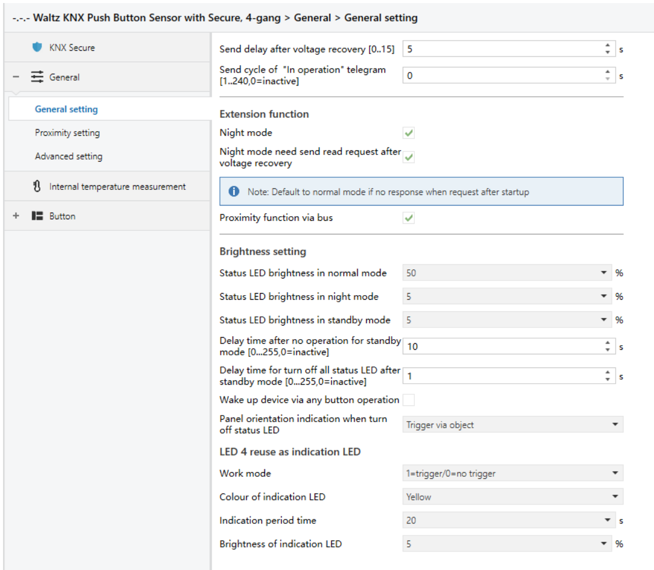
Fig.5.1.1 “General setting” parameter window
