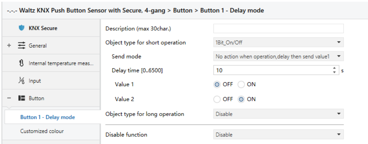
Fig.5.5.11 Parameter setting of delay mode function
