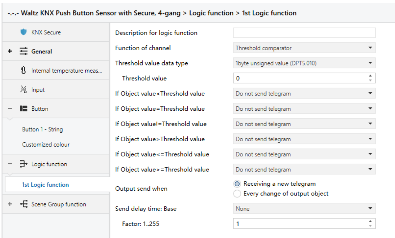
Fig.5.6.3 "Threshold comparator" parameter window
