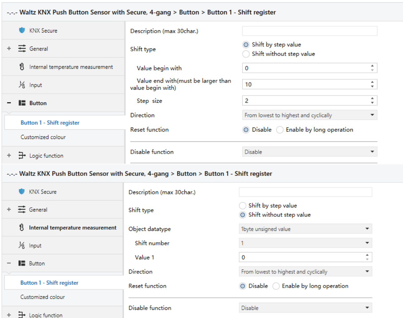
Fig.5.5.9 Parameter setting of shift register function
