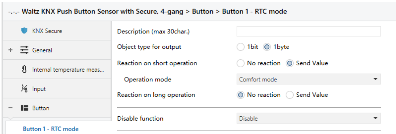
Fig.5.5.12 Parameter setting of RTC mode function
