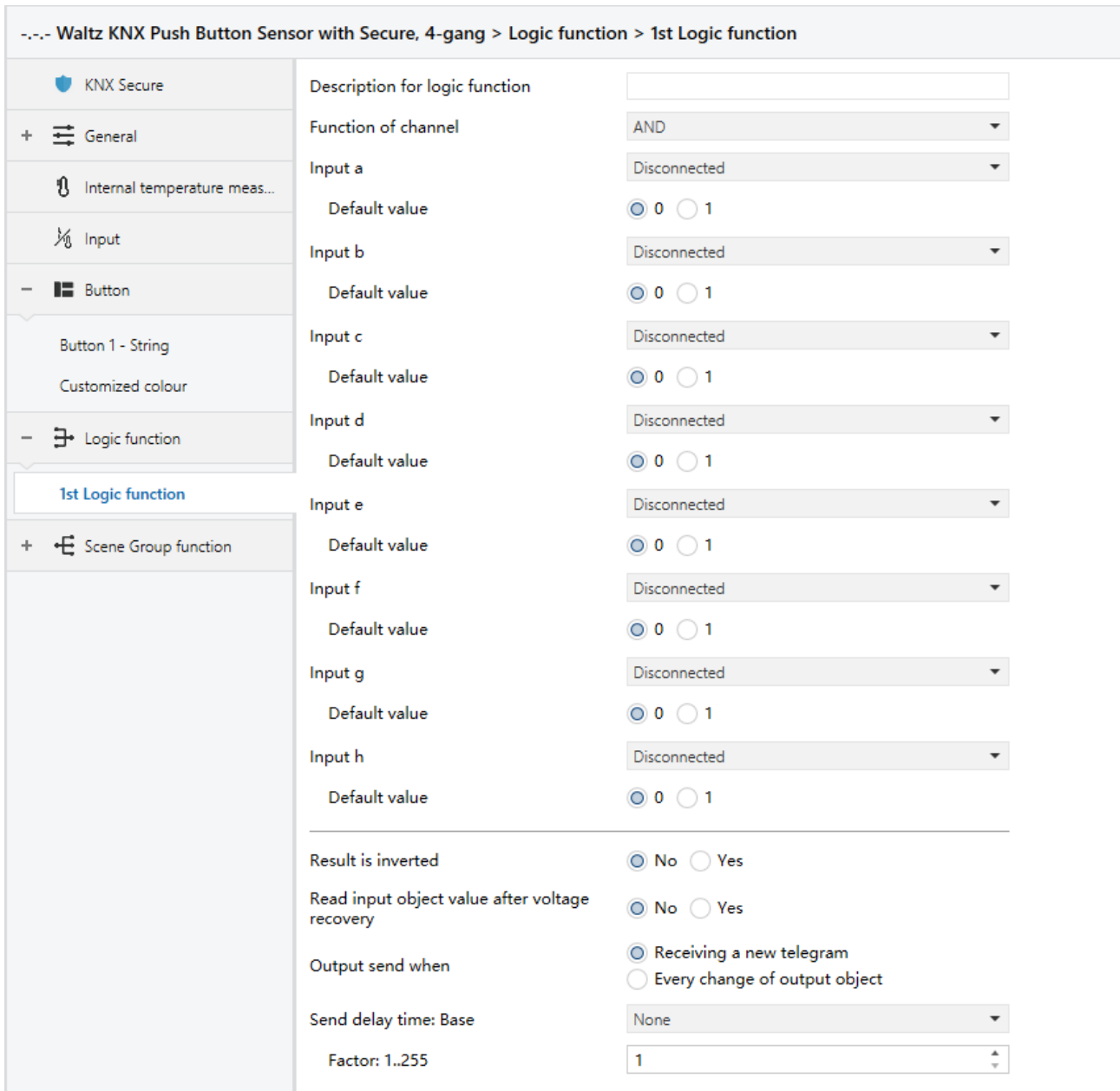
Fig.5.6.1 “AND/OR/XOR” parameter window
