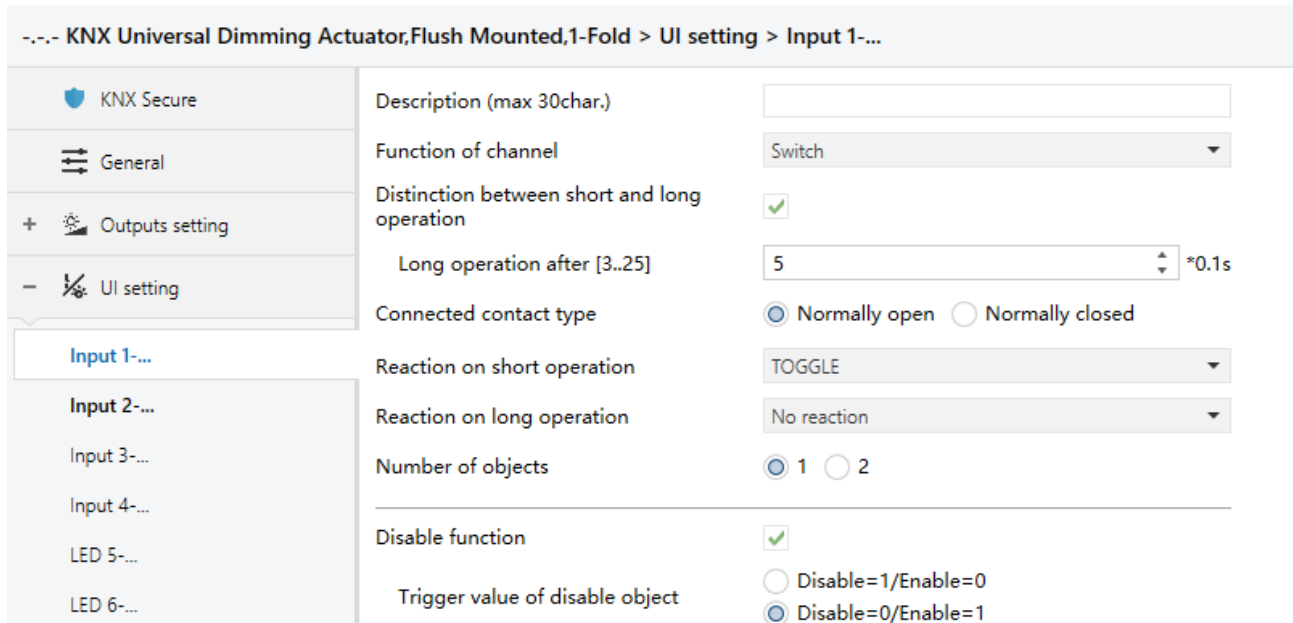
Fig.5.4.1.1 "Input x-Switch" parameter window
