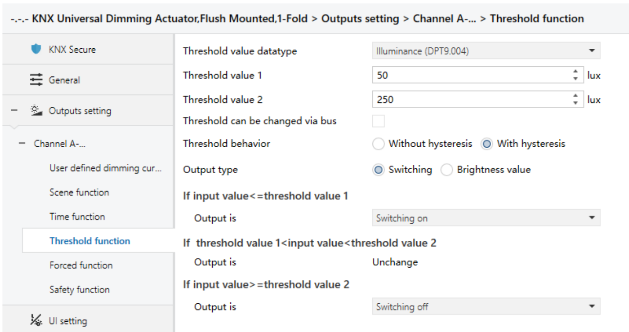
Fig.5.3.3.3 "Threshold function" parameter window
