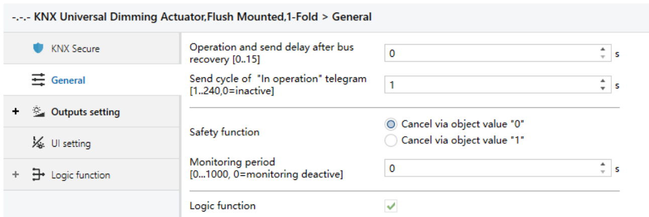
Fig.5.2 "General setting" parameter window
