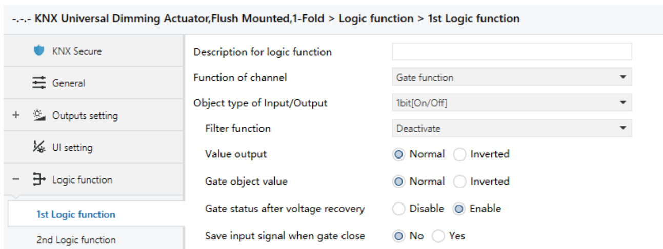
Fig.5.5.5 "Gate function" parameter window
