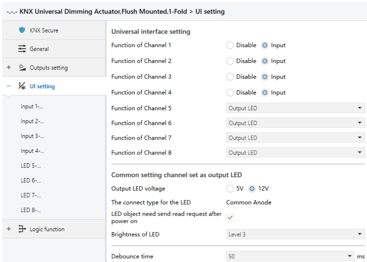
Fig.5.4 "UI setting" parameter window
