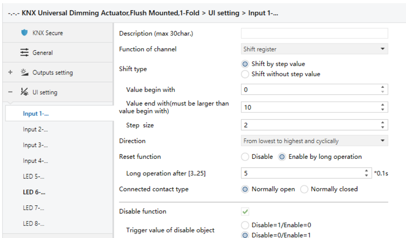
Fig.5.4.1.6 "Input x- Shift register" parameter window
