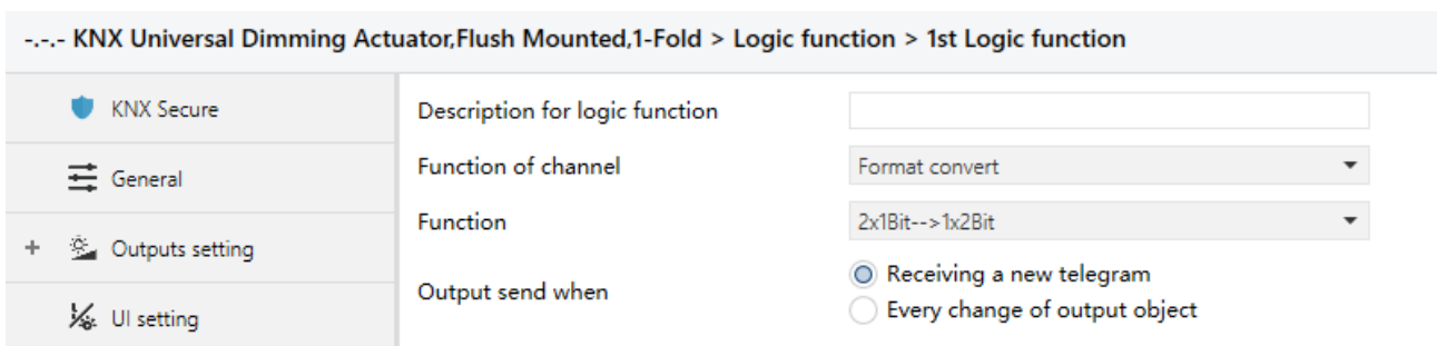
Fig.5.5.4 "Format convert" parameter window
