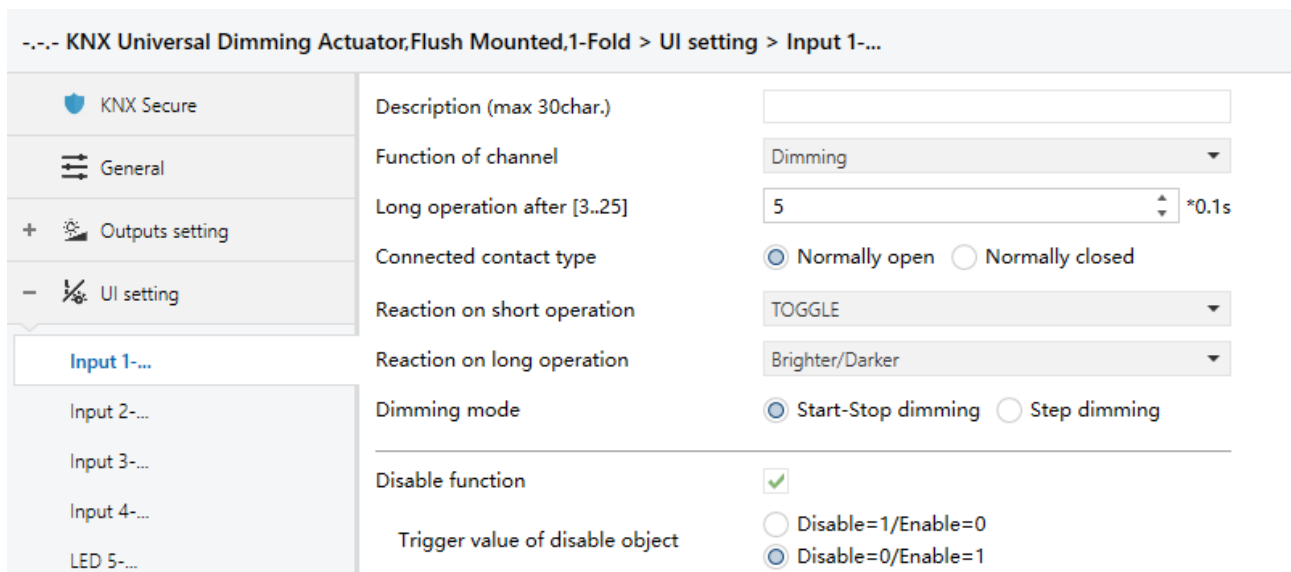
Fig.5.4.1.2 "Input x- Dimming"parameter window
