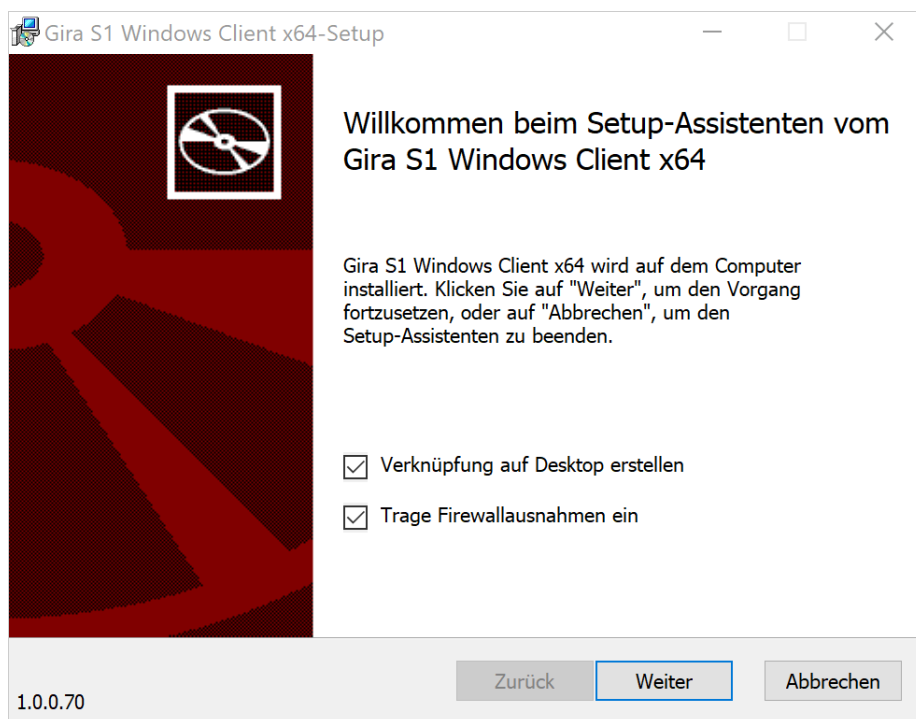
Bild 15: Installations-Dialog
