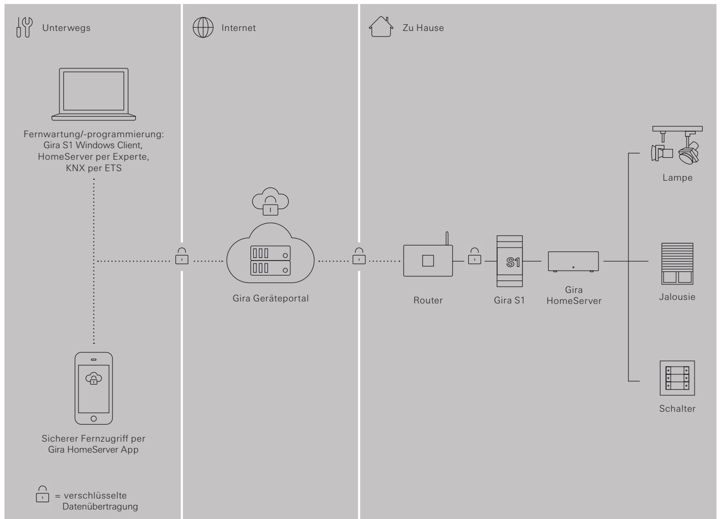
Bild 3: Sichere Konfiguration des Gira HomeServers mit dem Gira S1.
