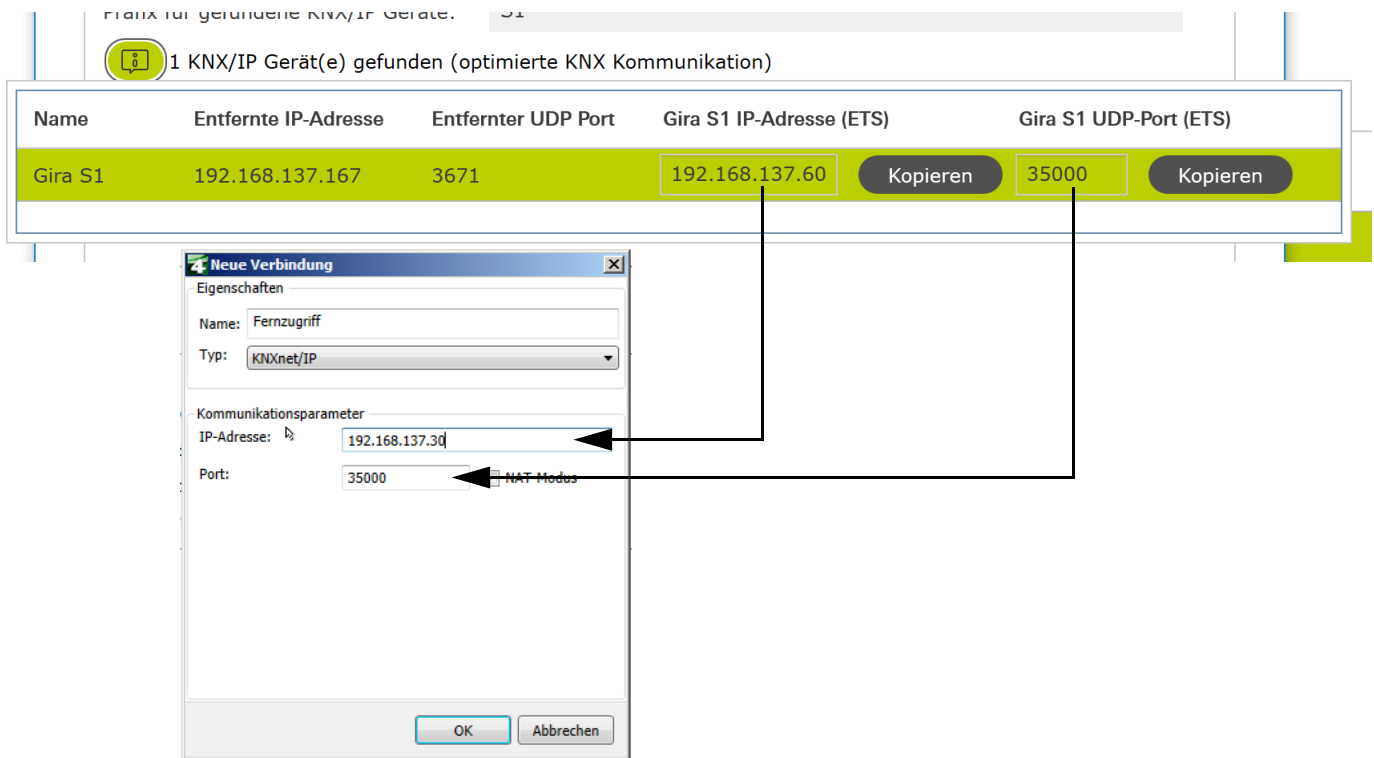
Bild 20: Manuelle KNX/IP Interfacekonfiguration für ETS kleiner ETS4.2.
