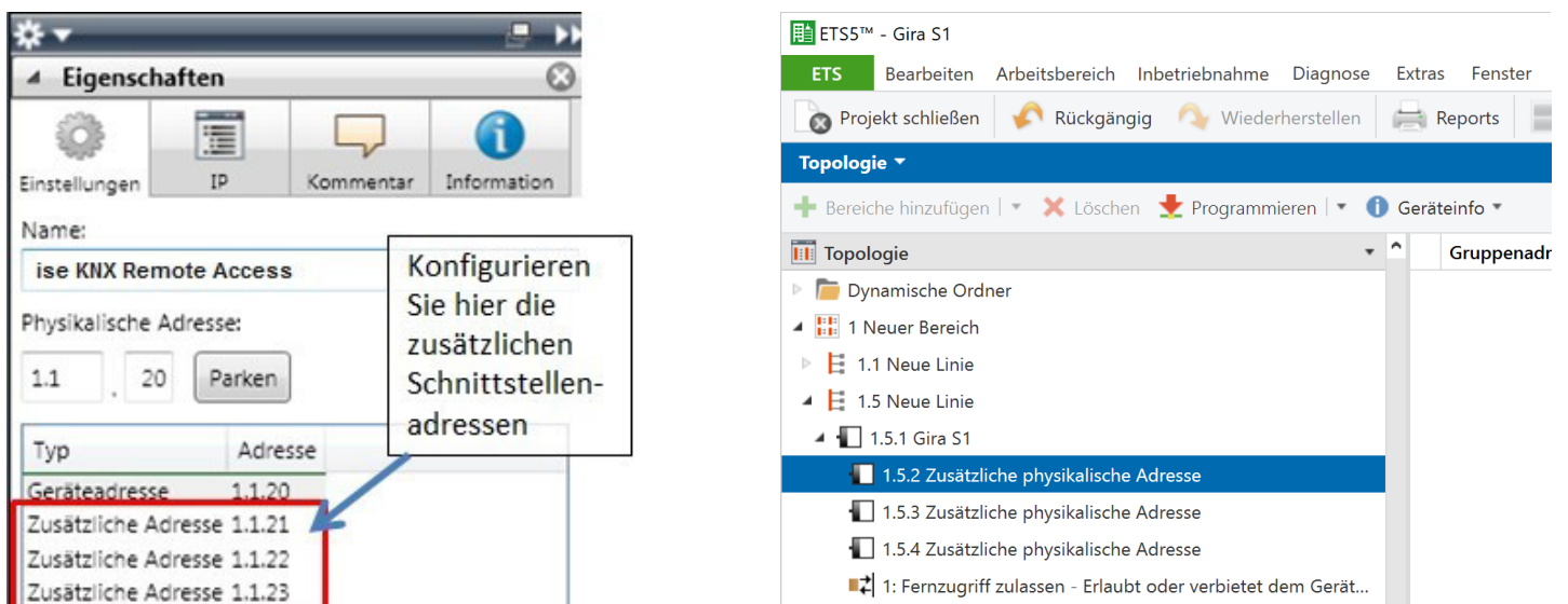
Bild 6: Zusätzliche physikalischen Adressen in der ETS4 (links) und der ETS5 (rechts)
