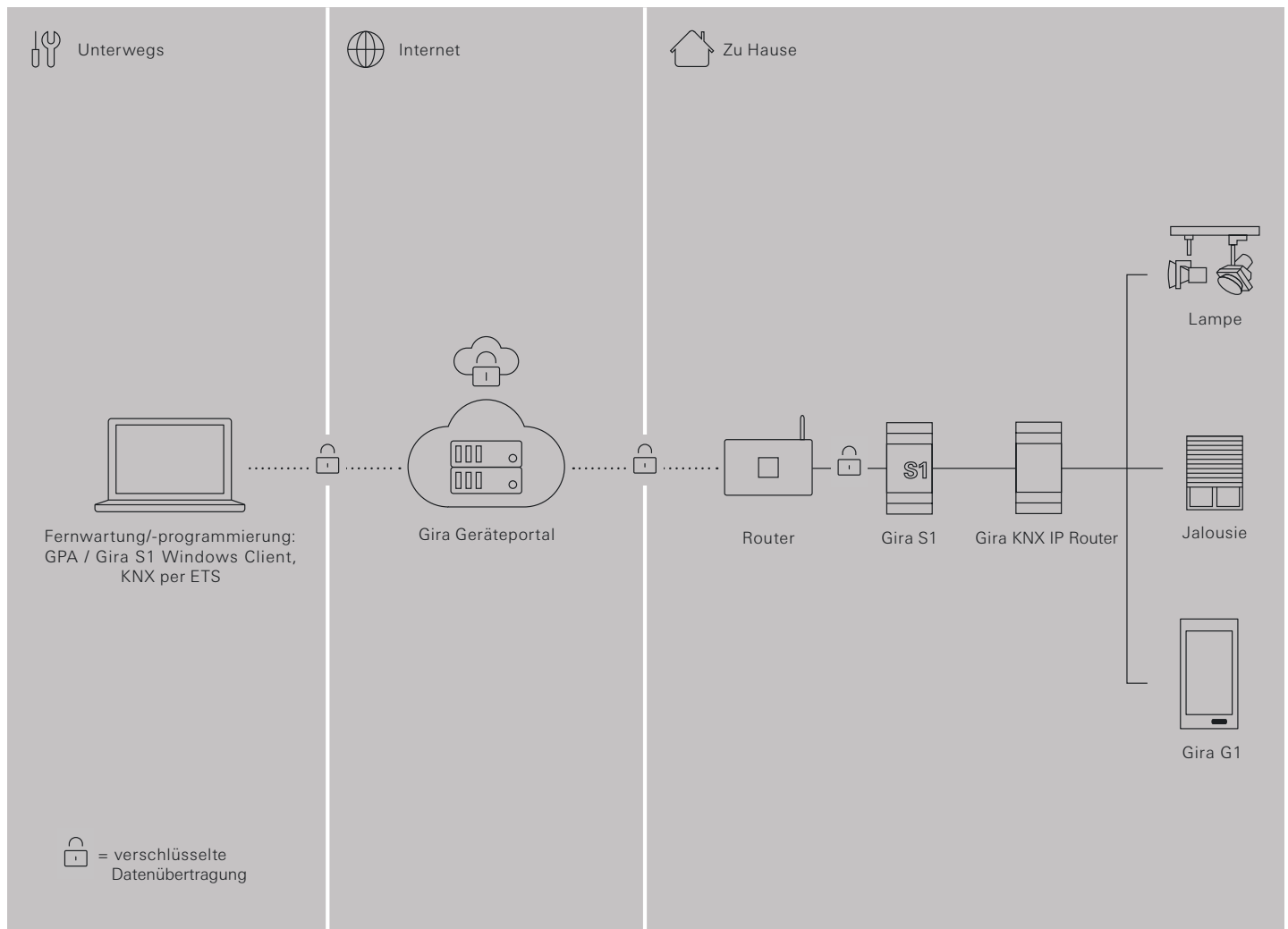
Bild 4: Sicherer Fernzugriff auf die KNX Installation mit dem Gira S1.
