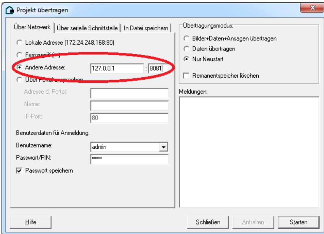
Bild 22: Projekt mit Experte über Fernzugriff übertragen.
