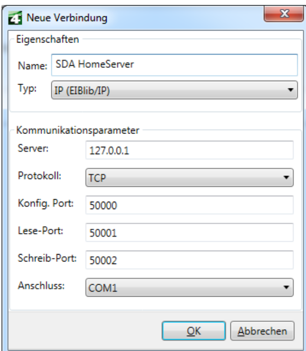
Bild 23: HomeServer mit Eiblib/IP über Fernzugriff für KNX Anbindung nutzen.
