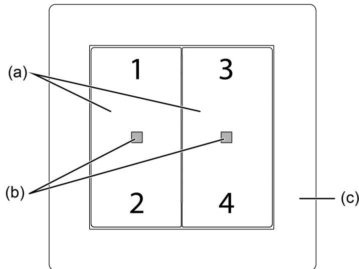
Bild 2: Geräteaufbau 2fach
