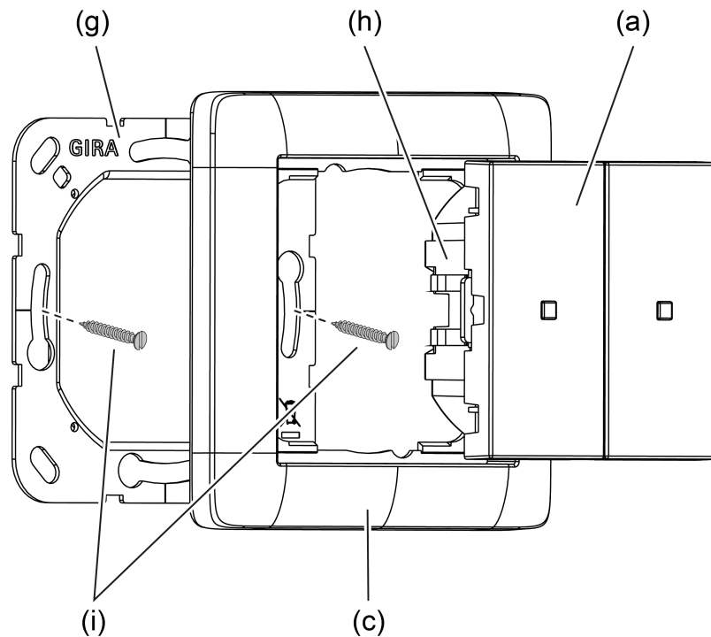
Bild 4: Gerät montieren
