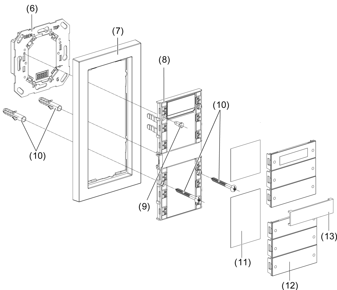
Bild 3: Gerätemontage eines Tastsensor 3 plus 6fach (doppelte Höhe)
