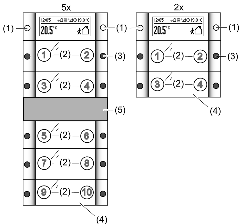
Bild 1: Geräteaufbau Tastensensoren 3 plus
