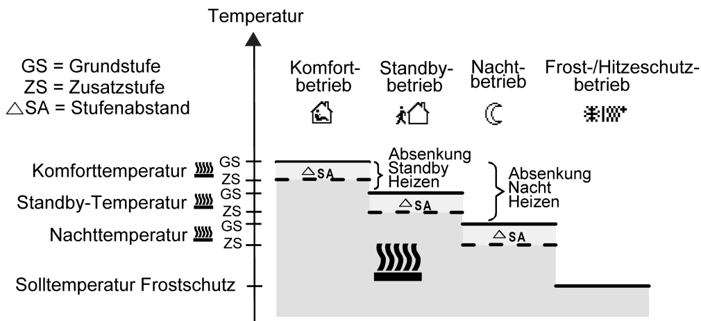
Bild 43: Solltemperaturen in der Betriebsart "Grund- und Zusatzheizen"
