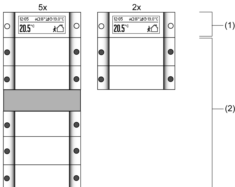
Bild 5: Anordnung der Bedienflächen auf der Gerätefront
