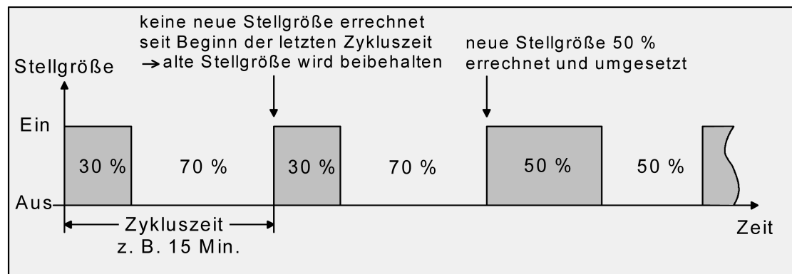
Bild 31: Schaltende PI-Regelung
