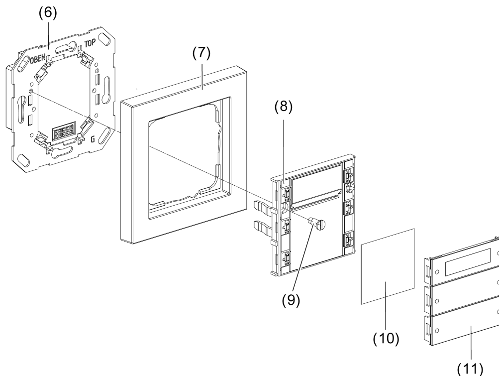
Bild 2: Gerätemontage eines Tastsensor 3 plus 2fach
