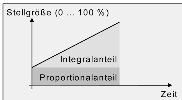
Bild 30: Stetige PI-Regelung
