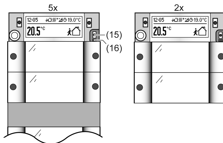
Bild 4: Anordnung der Programmier-LED und -Taste auf der Gerätefront
