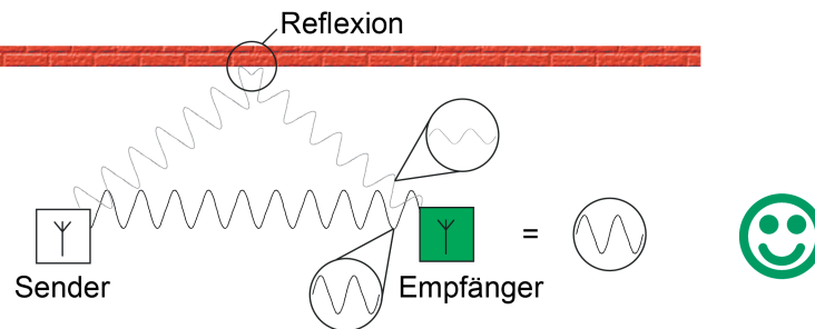
Bild 29: Interferenz beim Empfänger wirkungslos
