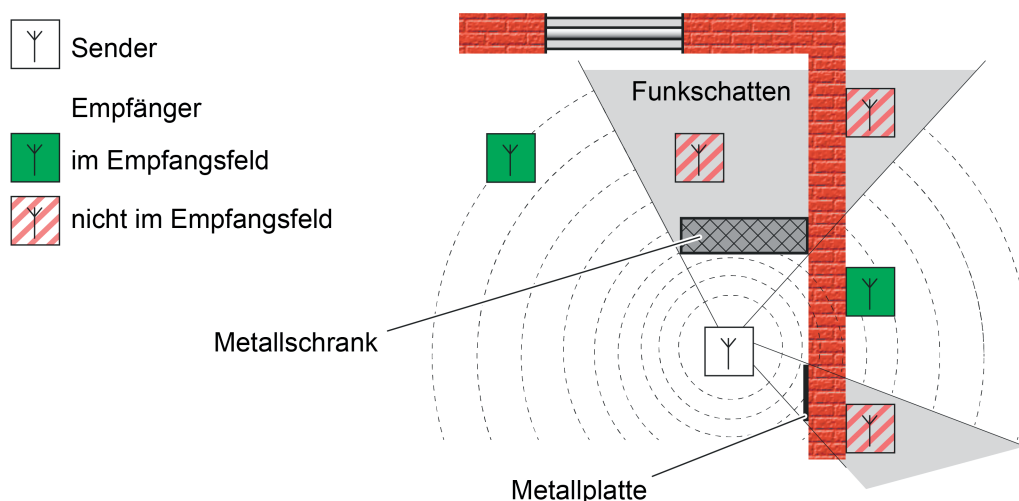
Bild 28: Funk Schatten in einem Gebäude durch Metallteile (idealisiert)
