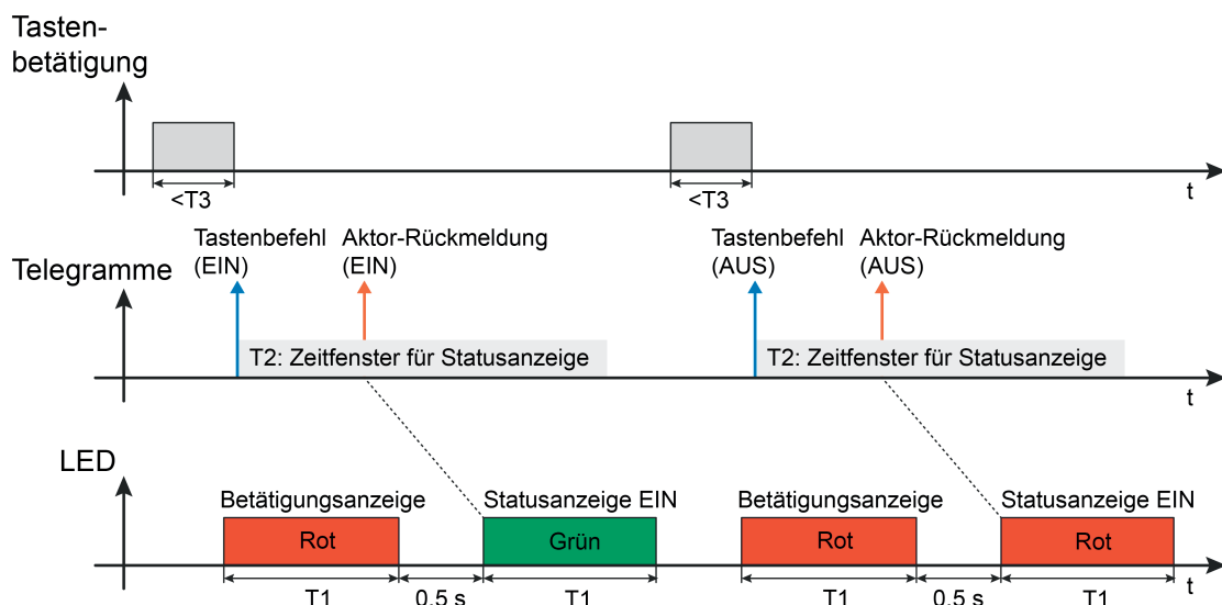
Bild 13: Beispiel einer Statusanzeige der Bedienfunktion "Dimmen" bei einem kurzen Tastendruck (mit Doppelstatus EIN und AUS)
