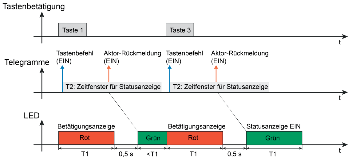
Bild 9: Beispiel einer 2-stufigen Betätigungs- und Statusanzeige Unterbrechung der Anzeigefunktion durch neue Tastenbetätigung
