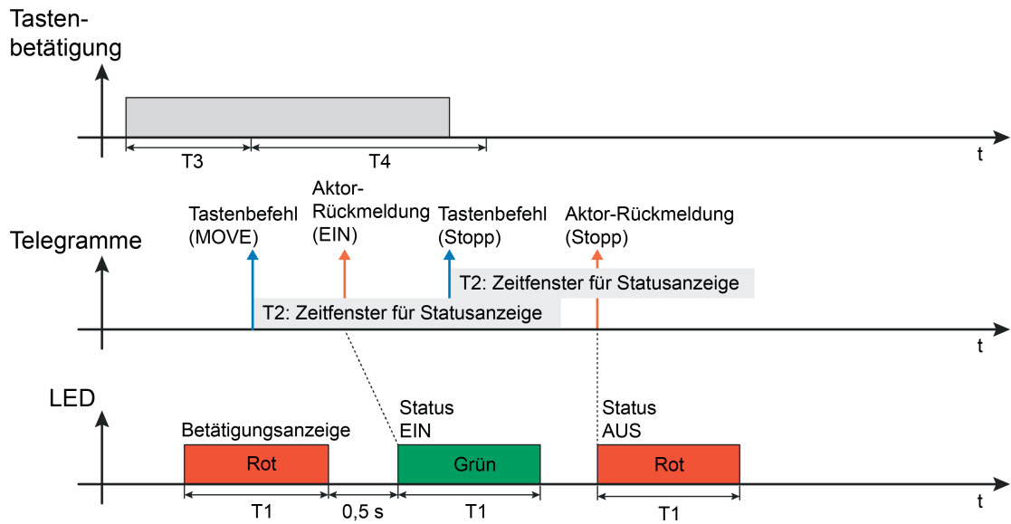
Bild 17: Beispiel einer Statusanzeige der Bedienfunktion "Jalousie" bei einem langen Tastendruck
