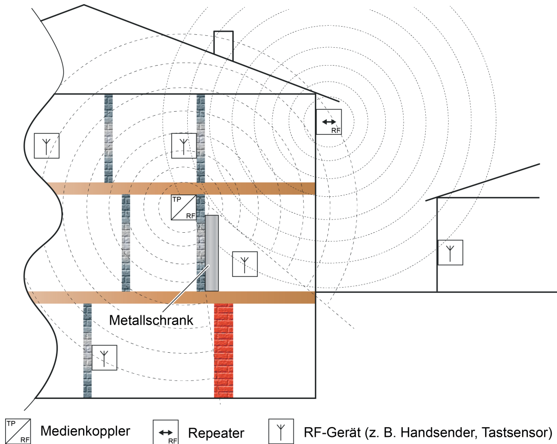
Bild 36: Verwendung eines Medienkopplers als Repeater zur Signalverstärkung und Beseitigung von Funkschatten für Innen- und Außenanwendungen
