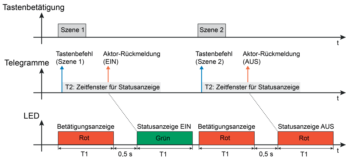
Bild 19: Beispiel einer Statusanzeige der Bedienfunktion "Szenennebenstelle" Szenennebenstelle ohne Speicherfunktion (mit Doppelstatus EIN und AUS)
