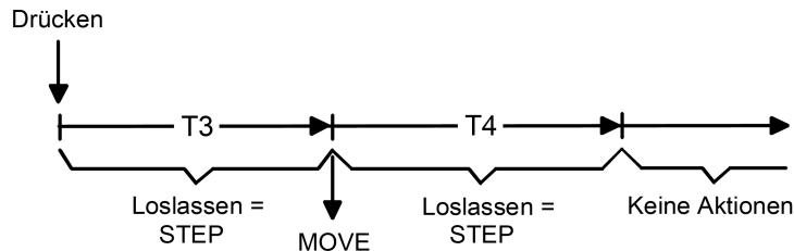
Bild 15: Bedienkonzept "Lang – Kurz oder Kurz"
