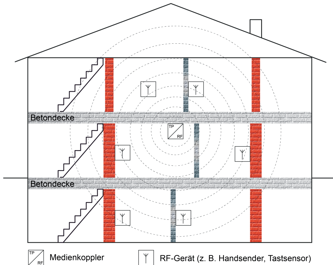
Bild 32: Gebäudestruktur mit einer KNX RF Linie (Beispiel)
