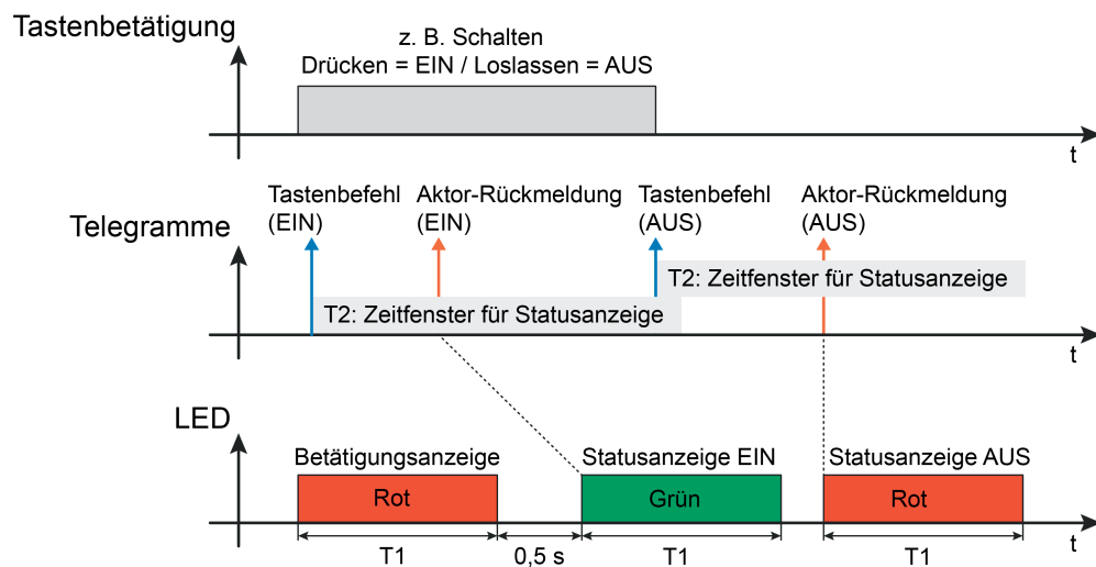
Bild 5: Beispiel einer 2-stufigen Betätigungs- und Statusanzeige mit Doppelstatus Neue Zeitfenster für Statusanzeige durch mehrere Bedientelegamente
