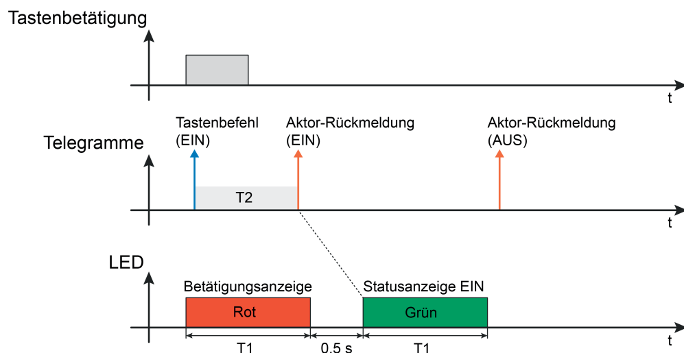
Bild 8: Beispiel einer 2-stufigen Betätigungs- und Statusanzeige mit Doppelstatus Empfang zweier Aktor-Statusmeldungen im Zeitfenster nicht zugelassen
