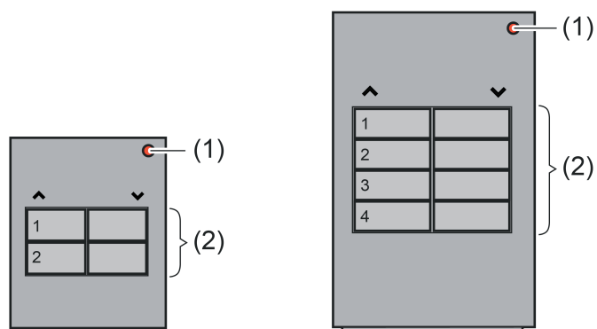
Bild 1: Geräteaufbau Handsender 2fach (links) und 4fach (rechts)
