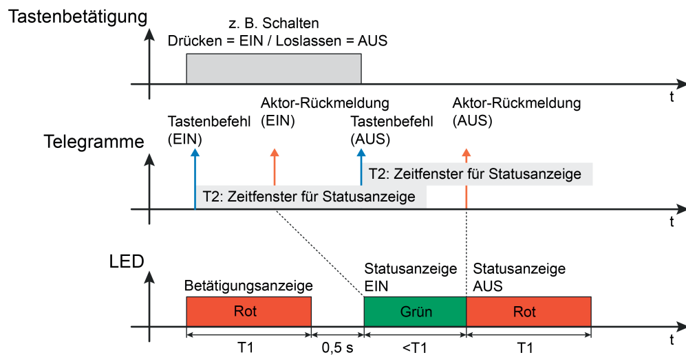
Bild 6: Beispiel einer 2-stufigen Betätigungs- und Statusanzeige mit Doppelstatus Unterbrechung der ersten Statusanzeige durch Aktorstatus im neuen Zeitfenster
