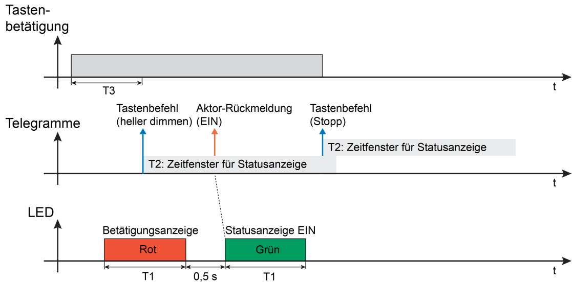
Bild 14: Beispiel einer Statusanzeige der Bedienfunktion "Dimmen" bei einem langen Tastendruck
