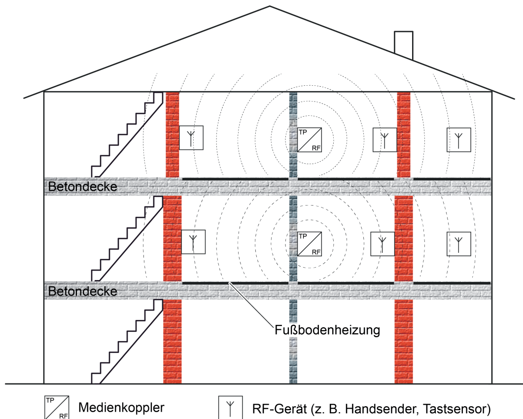
Bild 35: Gebäudestruktur mit zwei KNX RF Linien, die sich aufgrund der Gebäudebeschaffenheit nicht nachteilig beeinflussen (Beispiel)
