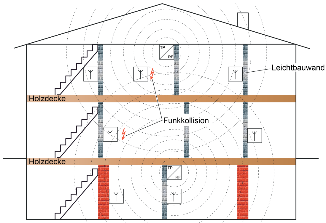
Bild 33: Gebäudestruktur mit zwei KNX RF Linien, ungünstige Beeinflussung (Beispiel)
