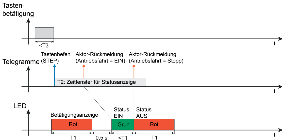
Bild 16: Beispiel einer Statusanzeige der Bedienfunktion "Jalousie" bei einem kurzen Tastendruck (mit Doppelstatus EIN und AUS)
