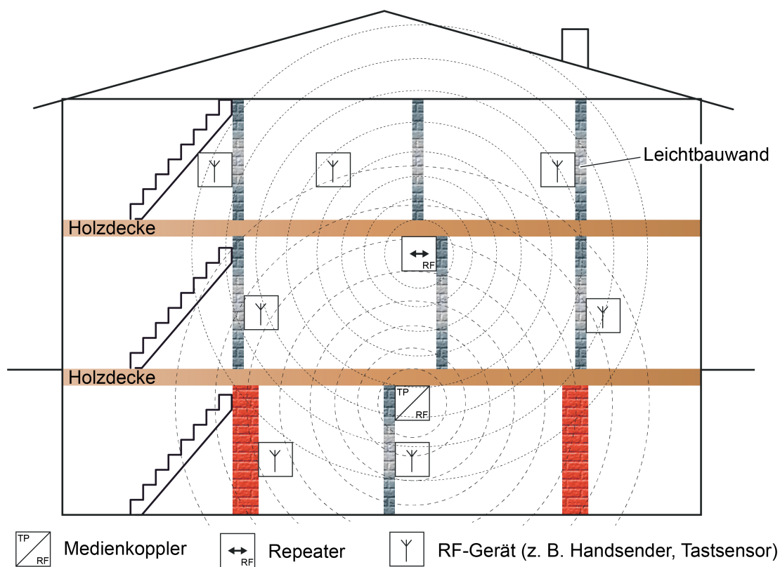
Bild 34: Gebäudestruktur mit einer KNX RF Linie und Repeater (Beispiel)
