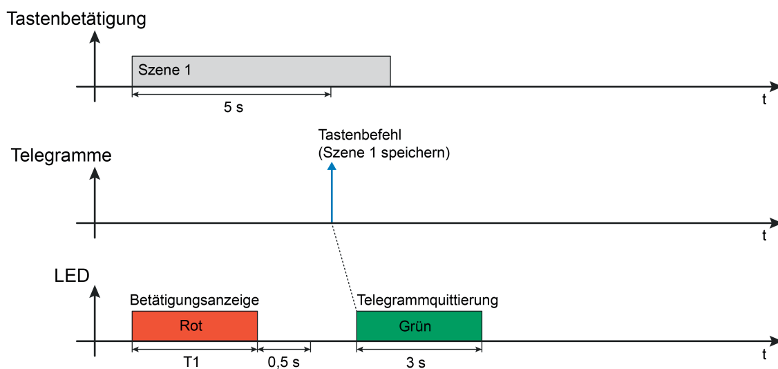
Bild 21: Beispiel einer LED-Anzeige der Bedienfunktion "Szenennebenstelle" Szenennebenstelle mit Speicherfunktion und Telegrammquittierung
