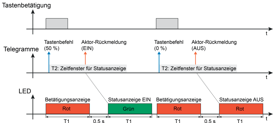
Bild 18: Beispiel einer Statusanzeige der Bedienfunktion "Wertgeber 1 Byte" mit Doppelstatus (EIN und AUS) Telegramm beim Drücken der Taste
