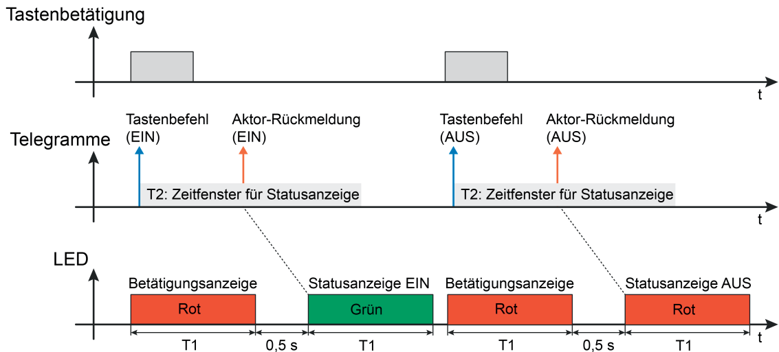
Bild 11: Beispiel einer Statusanzeige der Bedienfunktion "Schalten" mit Doppelstatus (EIN und AUS) Telegramm beim Drücken der Taste
