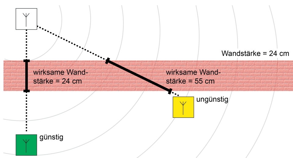
Bild 27: Dämpfung durch wirksame Wand- oder Deckenstärke
