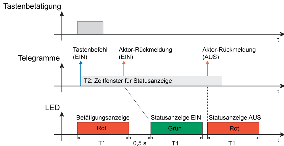
Bild 7: Beispiel einer 2-stufigen Betätigungs- und Statusanzeige mit Doppelstatus Empfang zweier Aktor-Statusmeldungen im Zeitfenster zugelassen
