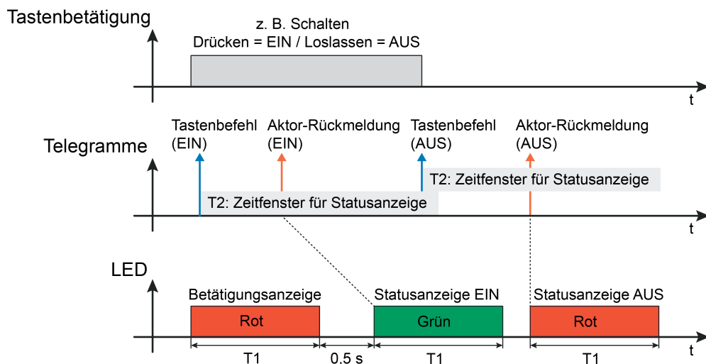
Bild 12: Beispiel einer Statusanzeige der Bedienfunktion "Schalten" mit Doppelstatus (EIN und AUS) Telegramm beim Drücken und Loslassen der Taste
