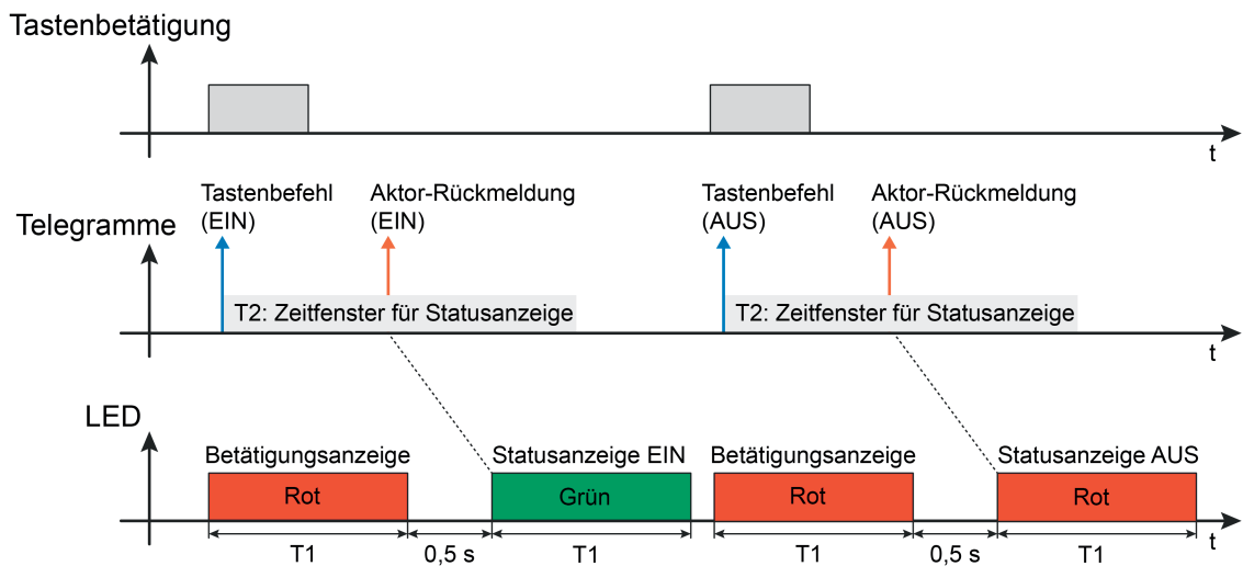
Bild 4: Beispiel einer 2-stufigen Betätigungs- und Statusanzeige mit Doppelstatus Statusanzeige Zustand "EIN" und "AUS" durch grüne und rote LED
