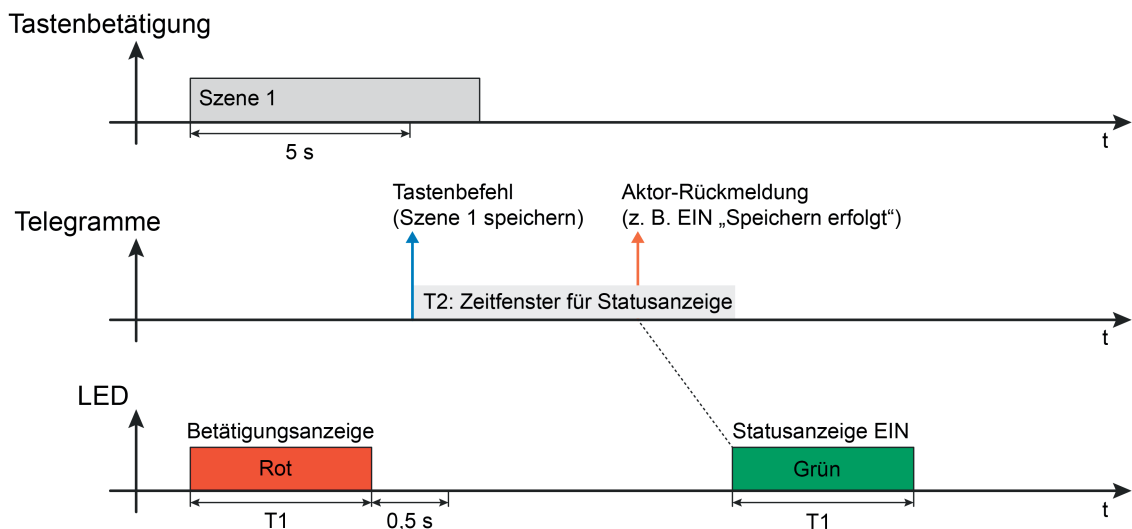
Bild 20: Beispiel einer Statusanzeige der Bedienfunktion "Szenennebenstelle" Szenennebenstelle mit Speicherfunktion und Statusanzeige (mit Einfachstatus EIN)
