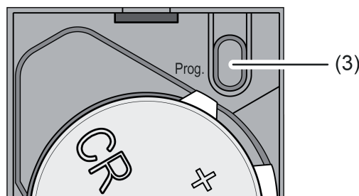
Bild 2: Programmiertaste im Batteriefach
