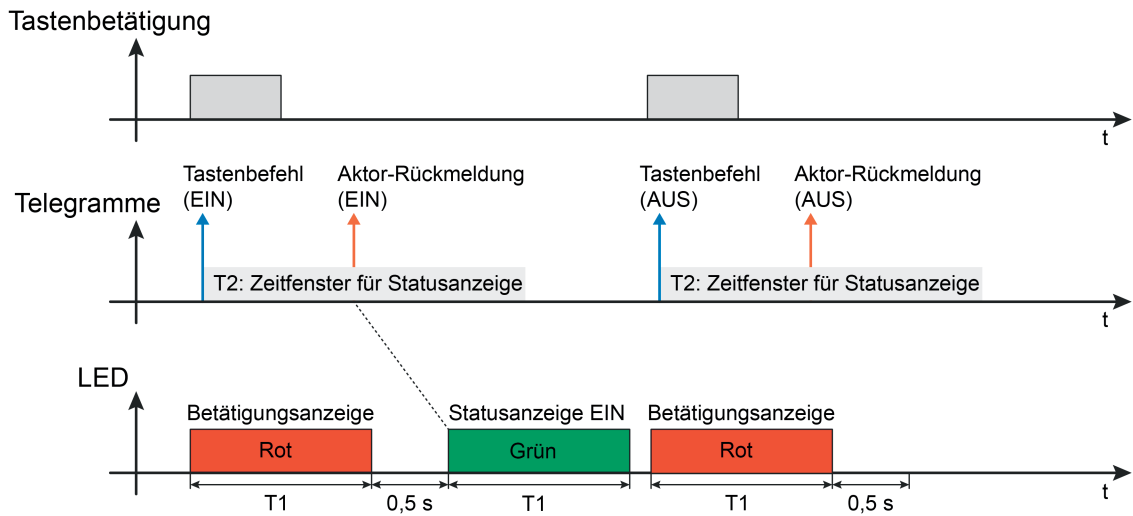
Bild 3: Beispiel einer 2-stufigen Betätigungs- und Statusanzeige mit Einfachstatus Statusanzeige Zustand "EIN" durch grüne LED
