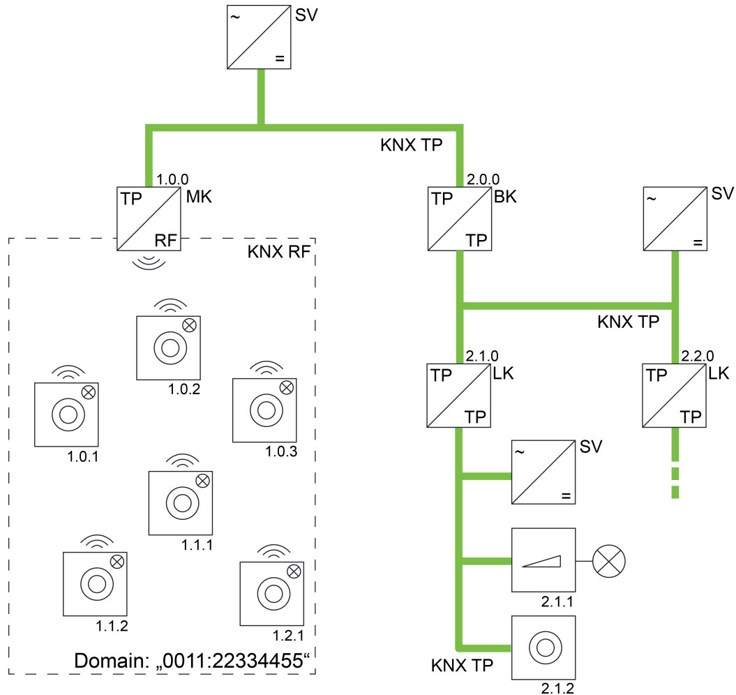
Bild 38: Beispiel einer möglichen KNX-Topologie mit RF- und TP-Linien Medienkoppler als Bereichskoppler
