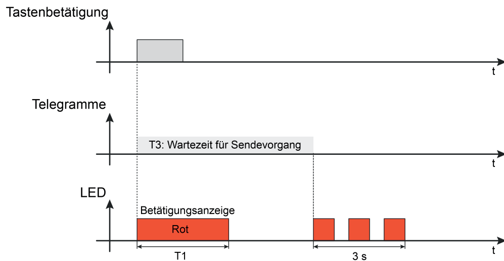
Bild 10: LED-Anzeige bei einem Übertragungsfehler
