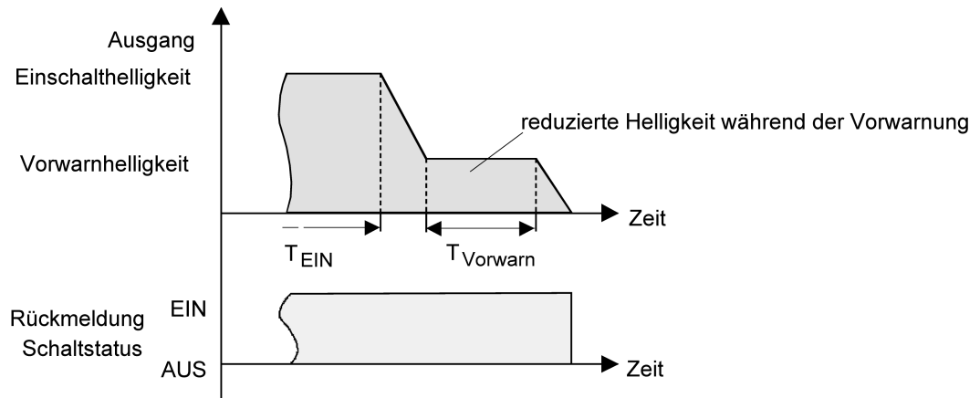
Bild 20: Die Vorwarnfunktion der Treppenhausfunktion mit Soft-AUS-Funktion (als Beispiel mit Minimalhelligkeit = 0 %)
