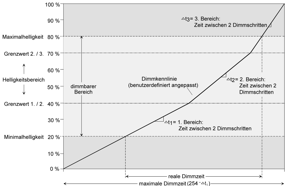
Bild 11: Benutzerdefinierte Dimmkennlinie als Beispiel mit Minimalhelligkeit und Maximalhelligkeit
