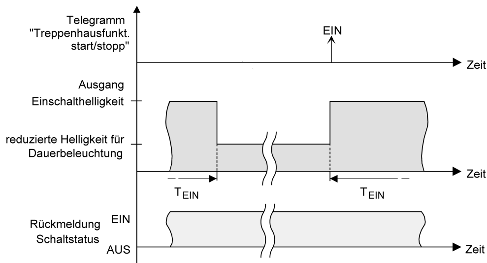
Bild 21: Die Dauerbeleuchtung der Treppenhausfunktion ohne Soft-Funktionen
