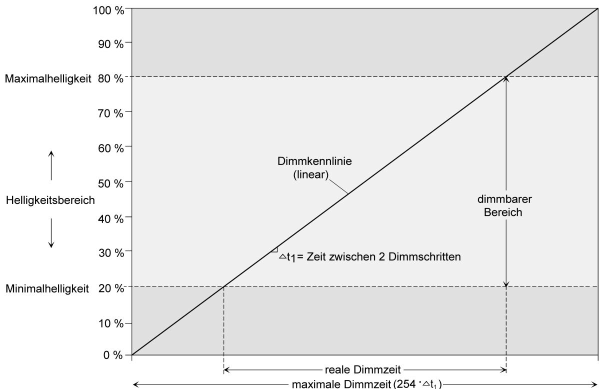
Bild 27: Lineare Dimmkennlinie als Beispiel mit Minimalhelligkeit > 0 % und Maximalhelligkeit
