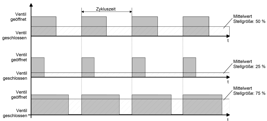
Bild 56: Resultierender Mittelwert durch variables Tastverhältnis bei einer Pulsweitenmodulation
