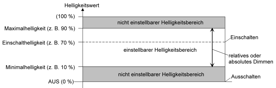
Bild 12: Beispiel eines Helligkeitsbereiches
