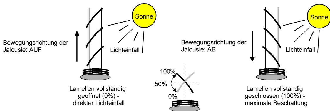
Bild 43: Typ 1 - Lamellenjalousien mit schräger Lamellenstellung in beide Fahrrichtungen
