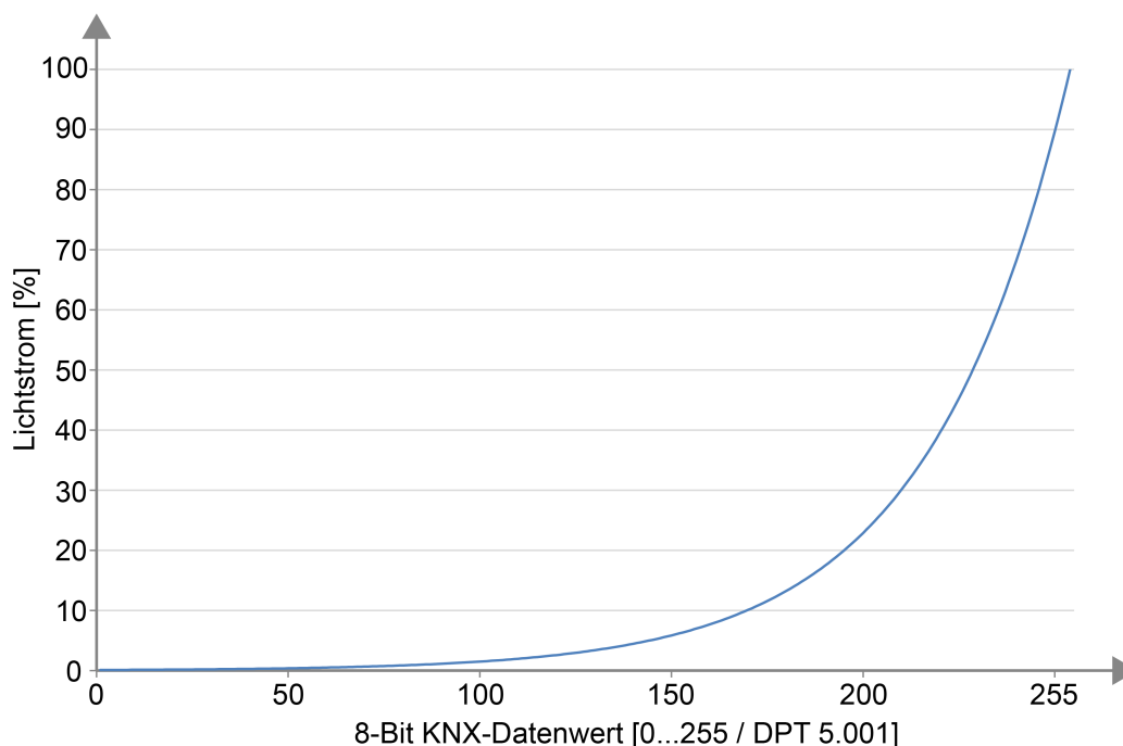
Bild 26: Logarithmische DALI-Dimmkennlinie (relativer Lichtstrom [%] abhängig vom 8-Bit KNX Datenwert [0...255])
