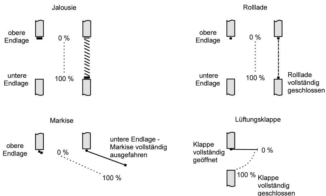
Bild 45: Positionsdefinition in Abhängigkeit der Antriebsart
