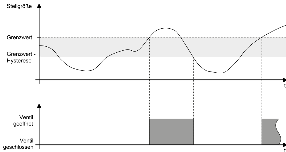
Bild 63: Beispiel einer Stellgrößenauswertung mit Grenzwert
