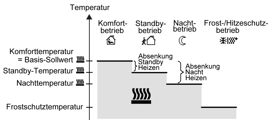
Bild 77: Solltemperaturen in der Betriebsart "Heizen"
