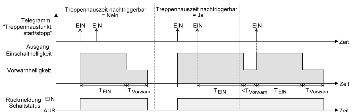
Bild 34: Einschaltverhalten der Treppenhausfunktion ohne Soft-Funktionen
