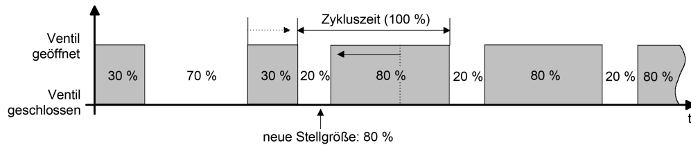
Bild 61: Beispiel einer Stellgrößenänderung 30 % -> 80 % während Schließphase des Ventils
