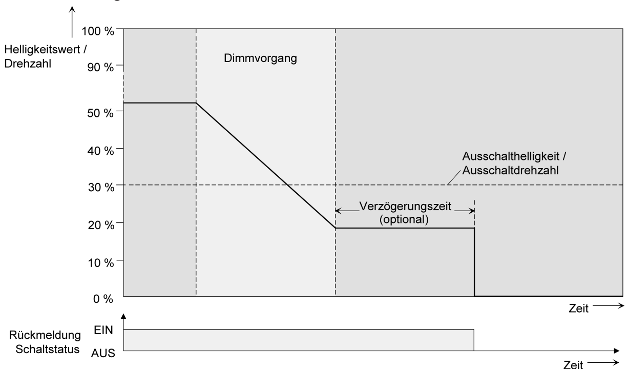
Bild 33: Dimm- und Schaltverhalten der automatischen Ausschaltfunktion
