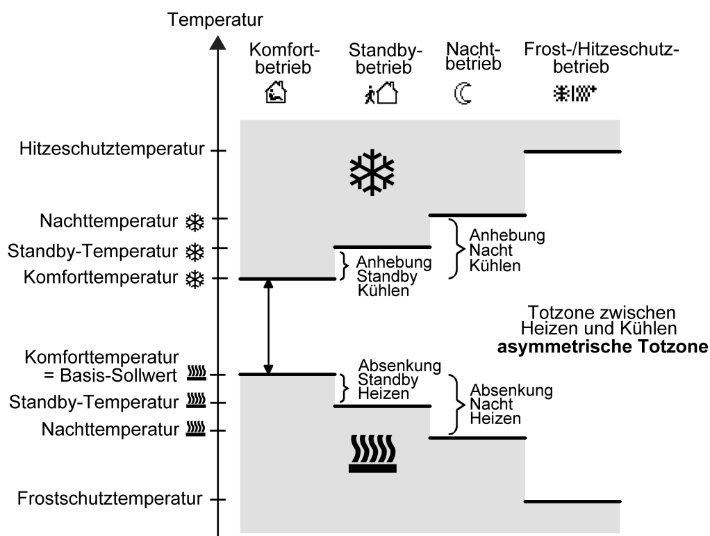
Bild 80: Solltemperaturen in der Betriebsart "Heizen und Kühlen" mit asymmetrischer Totzone
