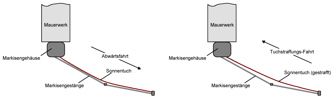
Bild 54: Tuchstraffung einer Markise
