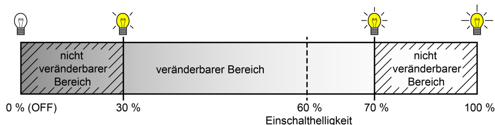
Bild 28: Beispiel eines Helligkeitsbereichs mit Einschalthelligkeit
