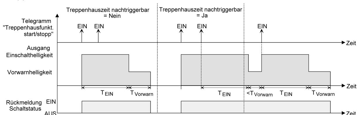
Bild 15: Einschaltverhalten der Treppenhausfunktion ohne Soft-Funktionen
