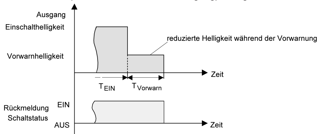
Bild 38: Die Vorwarnfunktion der Treppenhausfunktion ohne Soft-AUS-Funktion
