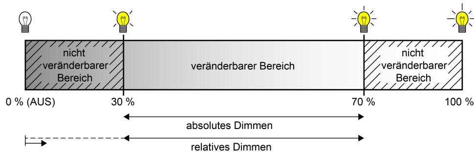
Bild 30: Beispiel eines dimmbaren Helligkeitsbereichs
