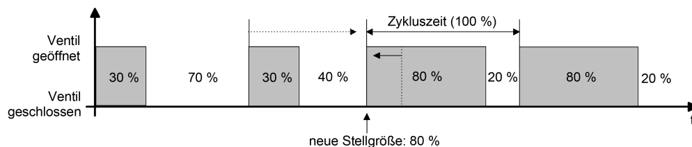
Bild 62: Beispiel einer Stellgrößenänderung 30 % -> 80 % während Öffnungsphase des Ventils (Öffnungsphase zu lang)
