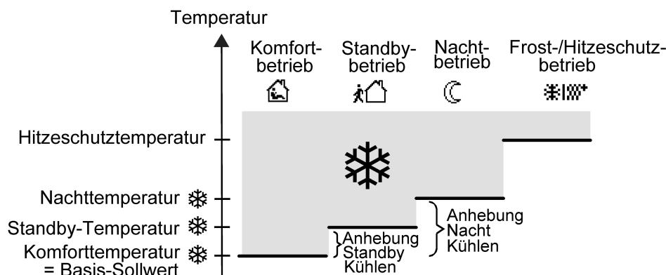
Bild 78: Solltemperaturen in der Betriebsart "Kühlen"
