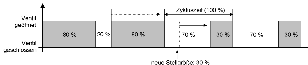
Bild 58: Beispiel einer Stellgrößenänderung 80 % -> 30 % während Schließphase des Ventils
