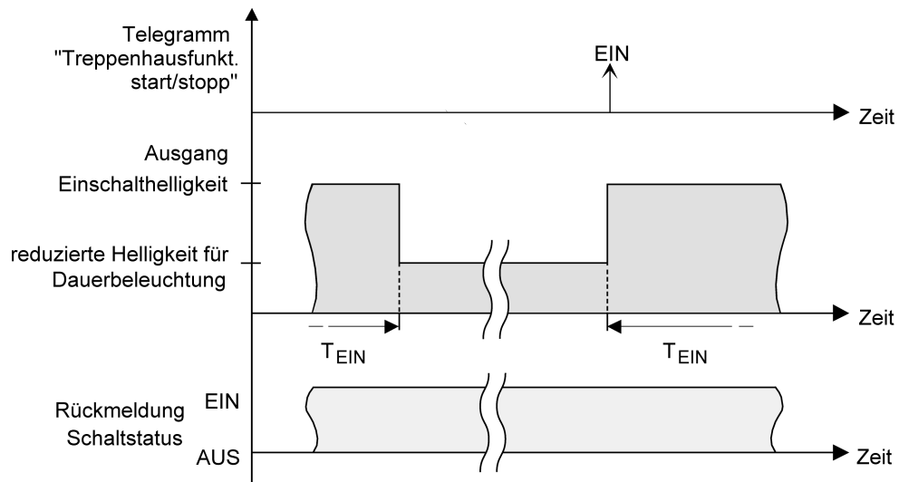
Bild 40: Die Dauerbeleuchtung der Treppenhausfunktion ohne Soft-Funktionen
