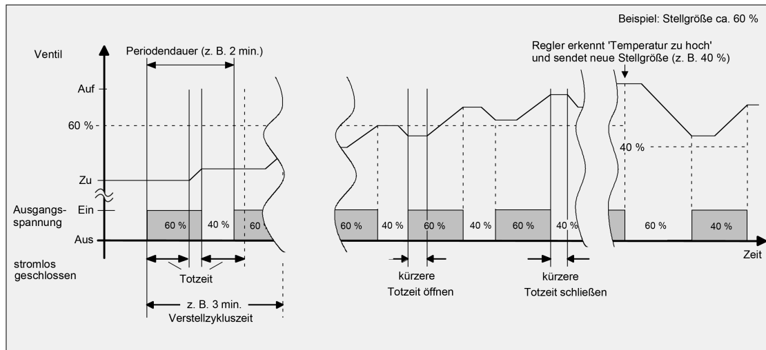
Bild 65: Idealisierter Verlauf des Ventilhubes exemplarisch dargestellt für eine Zykluszeit < Verstellzykluszeit
