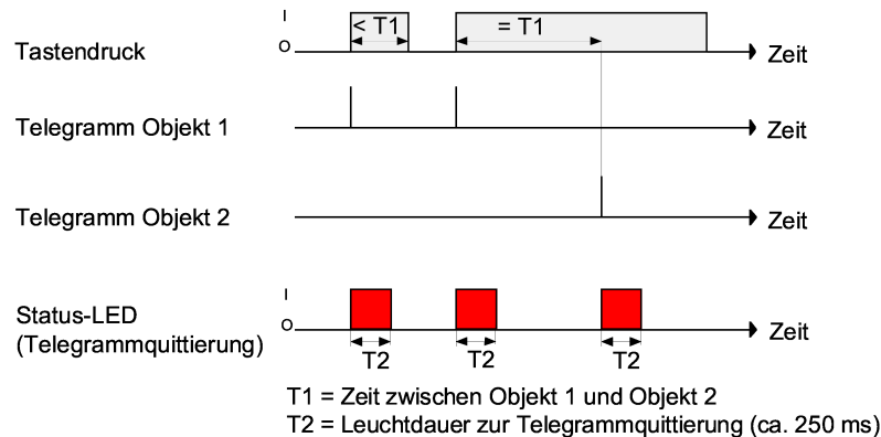
Bild 92: Beispiel zum Bedienkonzept "Kanal 1 und Kanal 2"
