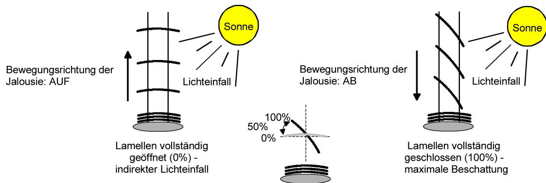
Bild 44: Typ 2 - Lamellenjalousien mit schräger und gerader Lamellenstellung
