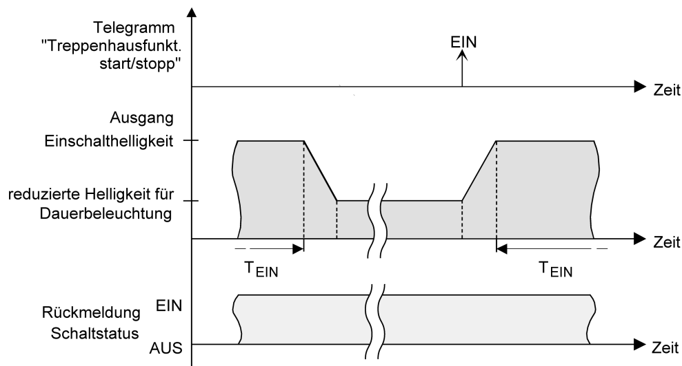
Bild 22: Die Dauerbeleuchtung der Treppenhausfunktion mit Soft-AUS-Funktion
