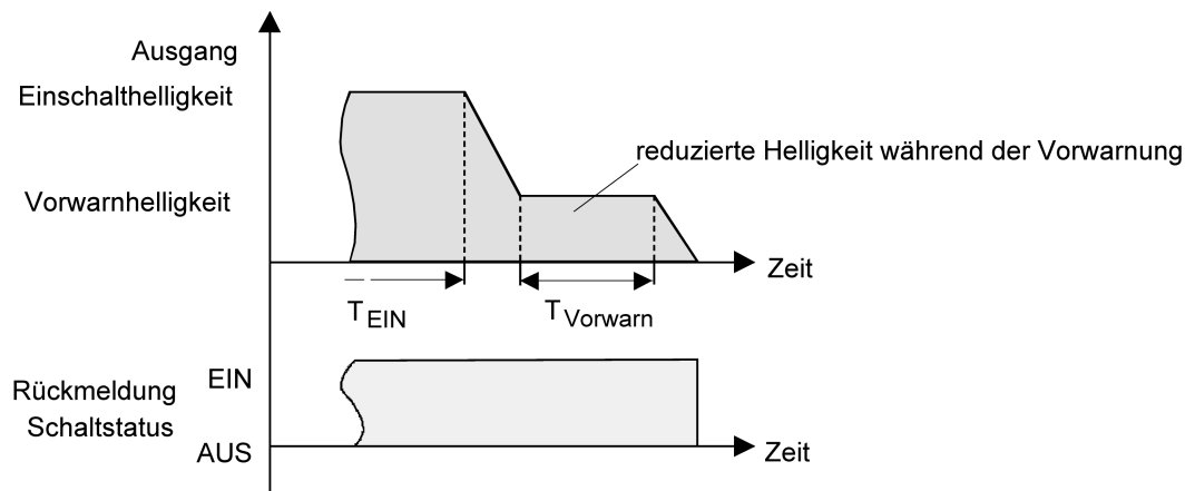
Bild 39: Die Vorwarnfunktion der Treppenhausfunktion mit Soft-AUS-Funktion (als Beispiel mit Minimalhelligkeit = 0 %)
