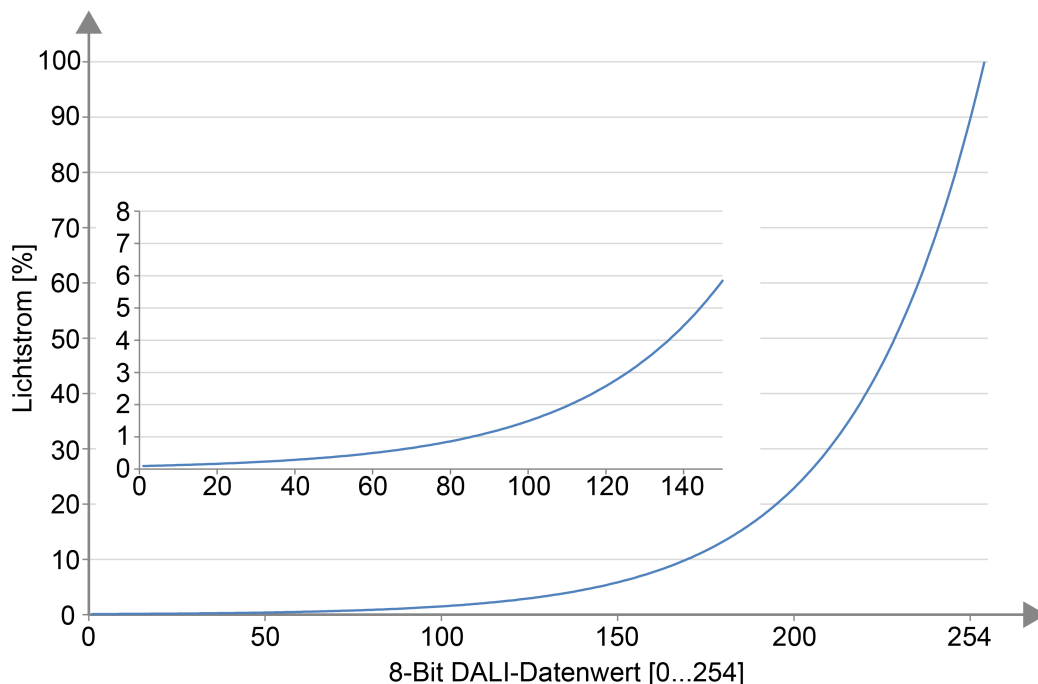
Bild 24: Logarithmische Dimmkurve in DALI-Betriebsgeräten (relativer Lichtstrom [%] abhängig vom 8-Bit DALI-Datenwert [0...254])
