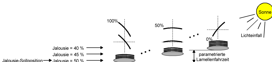
Bild 46: Beispiel für Lamellenpositionierung mit Auswirkung auf die Jalousieposition (Beispielhaft für Lamellentyp 1. Typ 2 sinngemäß gleich.)
