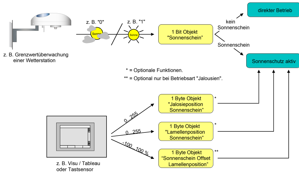
Bild 50: Prinzipschaltbild des Sonnenschutzes
