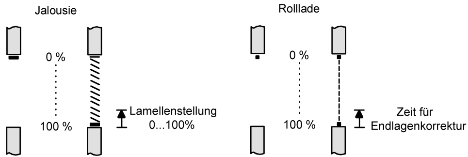
Bild 53: Endlagenkorrektur einer Jalousie oder Rolllade
