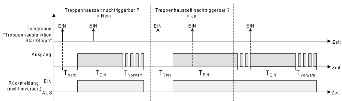
Bild 6: Einschaltverhalten der Treppenhausfunktion
