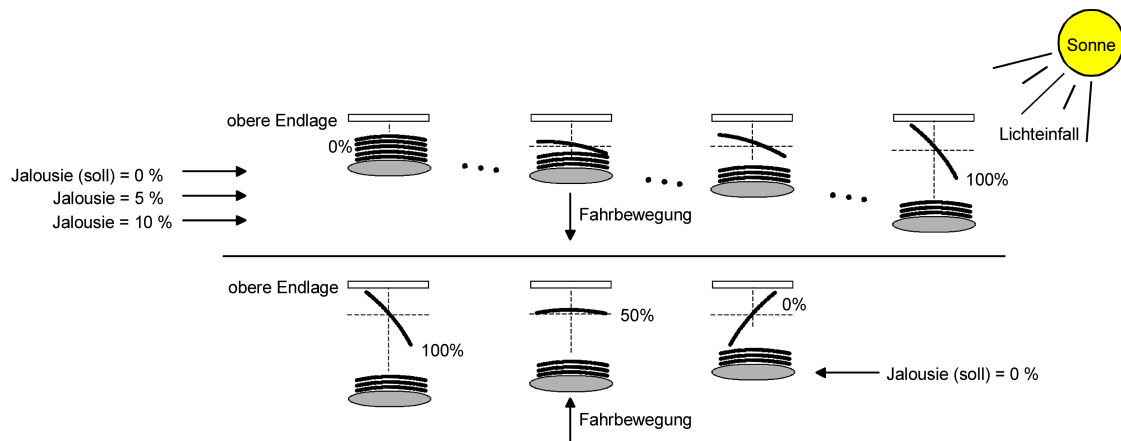
Bild 47: Beispiel für Lamellenpositionierung bei Jalousieposition in der oberen Endlage (Beispielhaft für Lamellentyp 1.)
