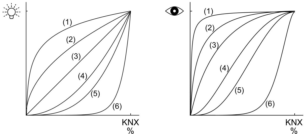
Bild 9: Dimmkennlinien im Wertebereich
