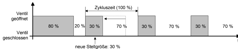
Bild 57: Beispiel einer Stellgrößenänderung 80 % -> 30 % während Öffnungsphase des Ventils
