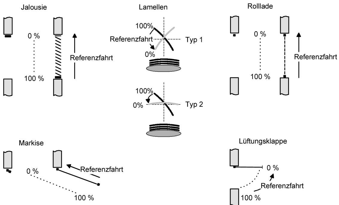
Bild 48: Referenzfahrt
