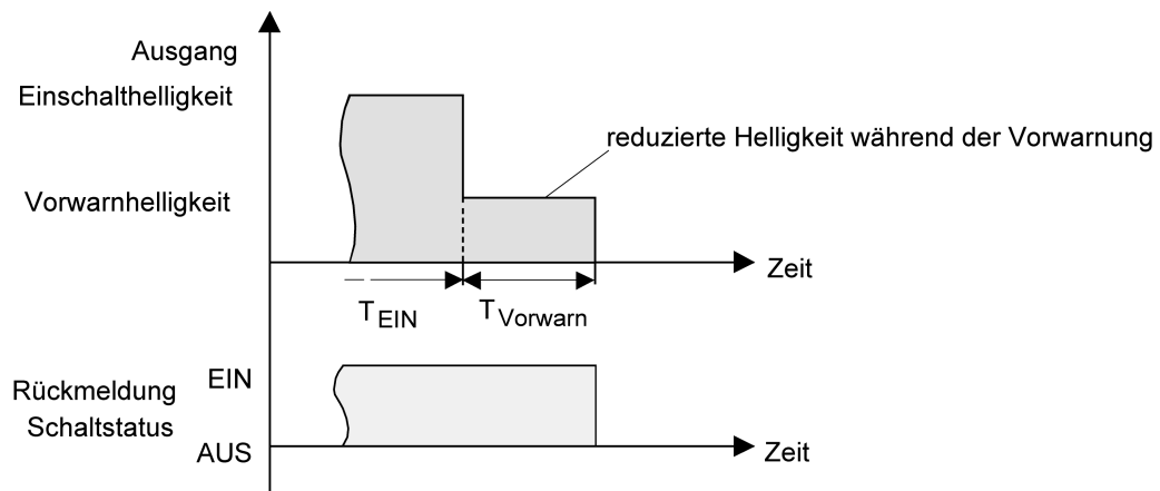
Bild 19: Die Vorwarnfunktion der Treppenhausfunktion ohne Soft-AUS-Funktion
