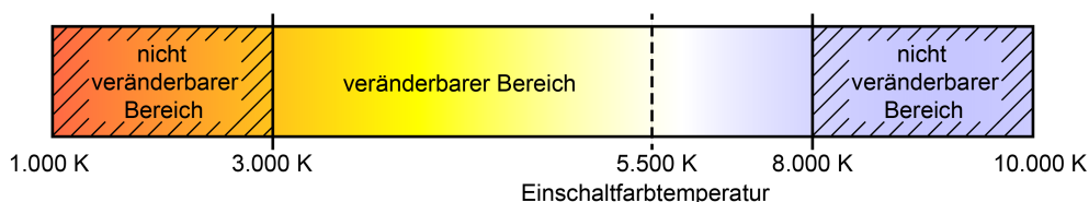
Bild 29: Beispiel eines konfigurierten Farbtemperaturbereichs mit Einschaltfarbtemperatur
