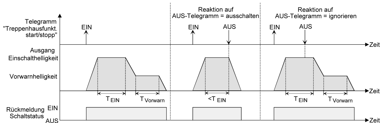
Bild 37: Ausschaltverhalten der Treppenhausfunktion mit Soft-Funktionen (als Beispiel mit Minimalhelligkeit = 0 %)
