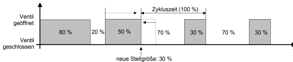
Bild 59: Beispiel einer Stellgrößenänderung 80 % -> 30 % während Öffnungsphase des Ventils (Öffnungsphase zu lang)
