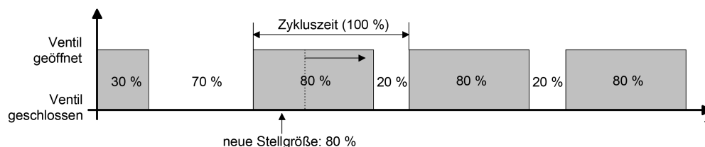
Bild 60: Beispiel einer Stellgrößenänderung 30 % -> 80 % während Öffnungsphase des Ventils
