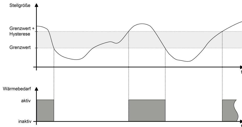
Bild 55: Wärmebedarfsinformation mit beispielhaftem Stellgrößenverlauf
