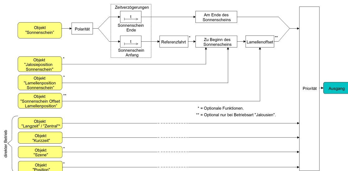
Bild 51: Funktionsschaltbild des Sonnenschutzes
