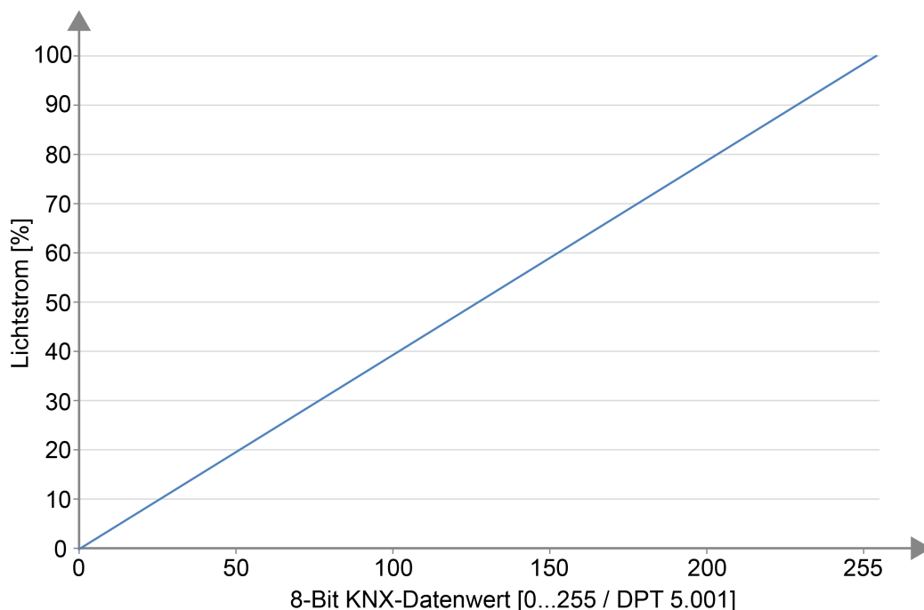
Bild 25: Lineare DALI-Dimmkennlinie (relativer Lichtstrom [%] abhängig vom 8-Bit KNX Datenwert [0...255])
