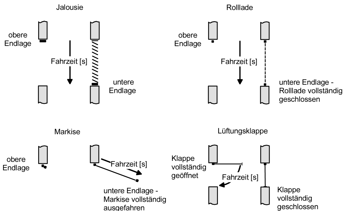
Bild 42: Ermittlung der Fahrzeit in Abhängigkeit der Antriebsart
