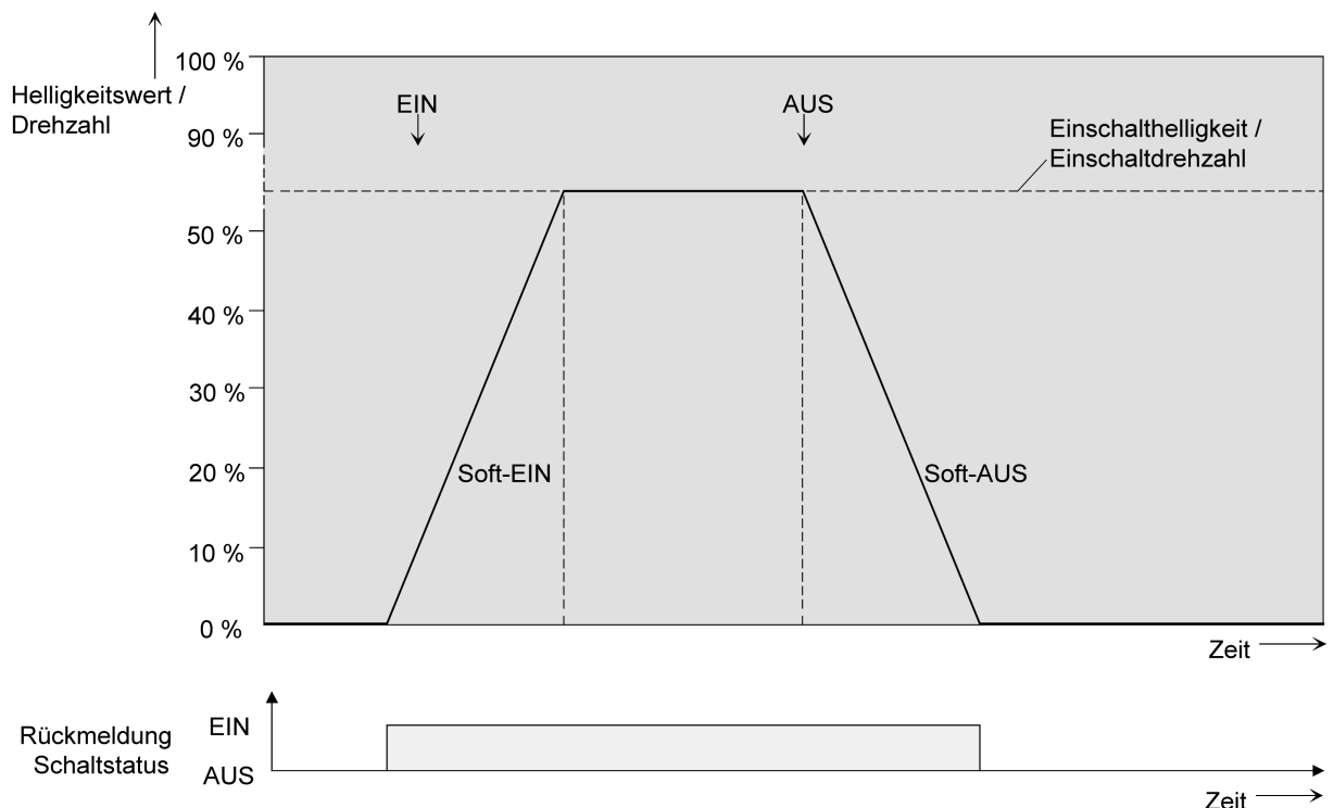
Bild 13: Dimmverhalten der Soft-EIN/AUS-Funktionen (als Beispiel)
