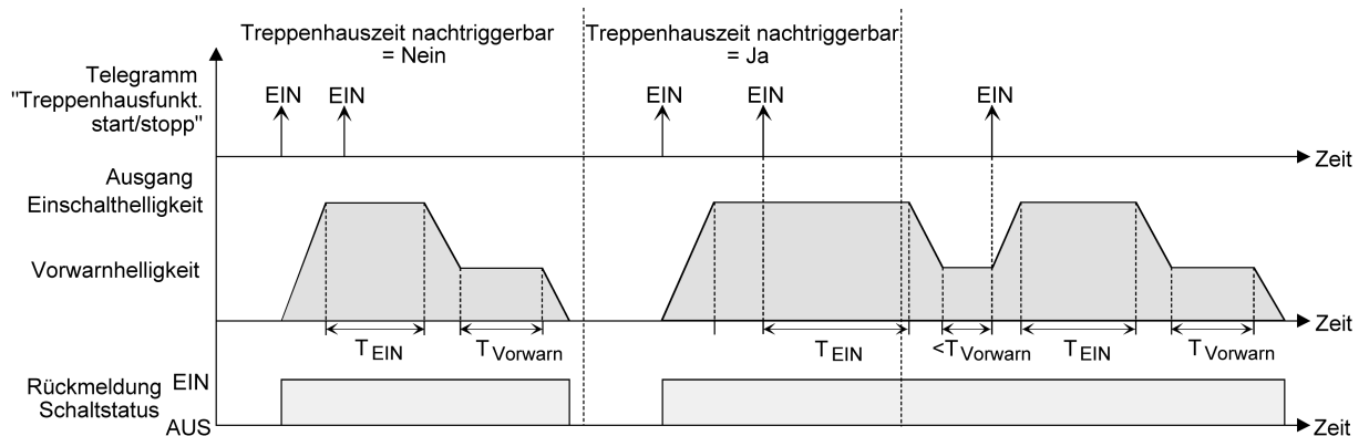
Bild 16: Einschaltverhalten der Treppenhausfunktion mit Soft-Funktionen (als Beispiel mit Minimalhelligkeit = 0 %)
