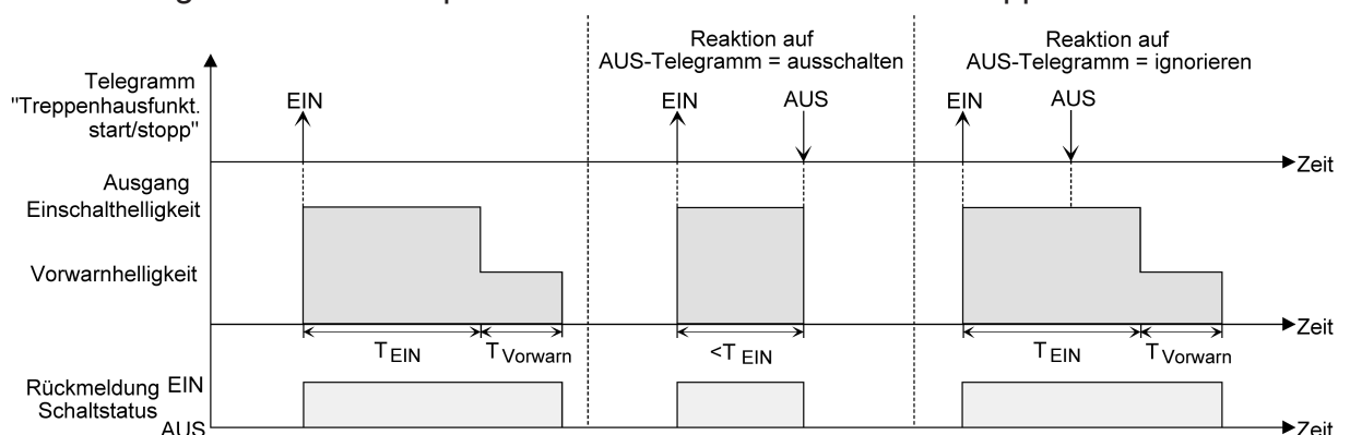
Bild 36: Ausschaltverhalten der Treppenhausfunktion ohne Soft-Funktionen
