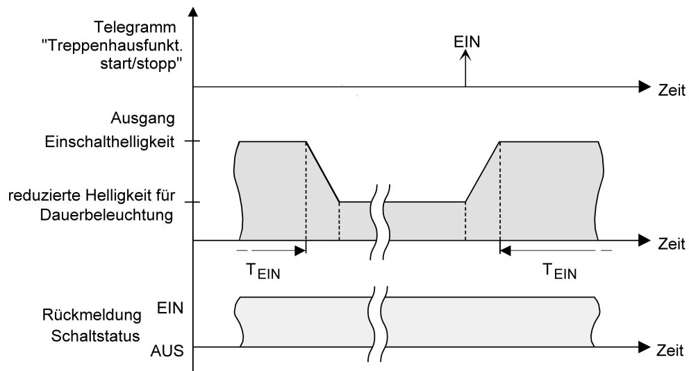
Bild 41: Die Dauerbeleuchtung der Treppenhausfunktion mit Soft-AUS-Funktion
