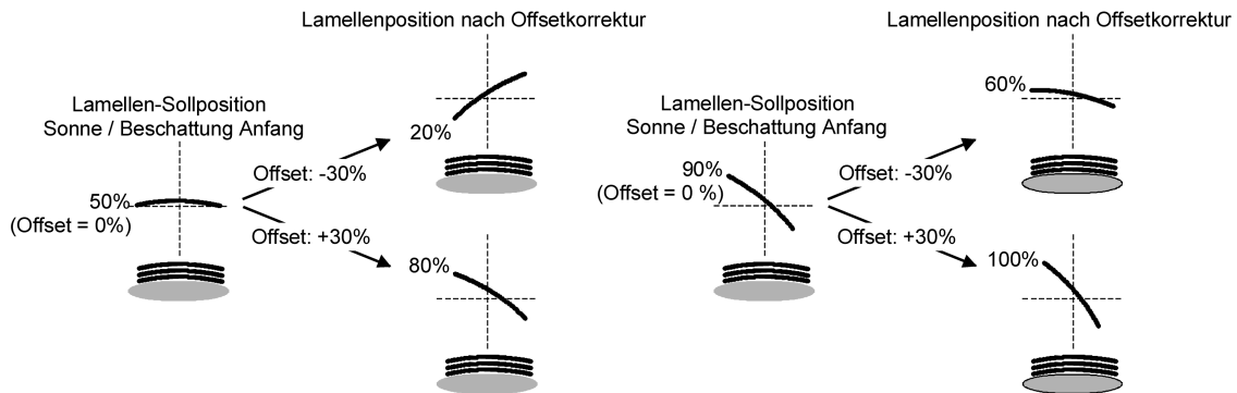
Bild 52: Funktionsweise des Lamellenoffsets als Beispiel (beispielhaft für Lamellentyp 1 / Lamellentyp 2 sinngemäß gleich)
