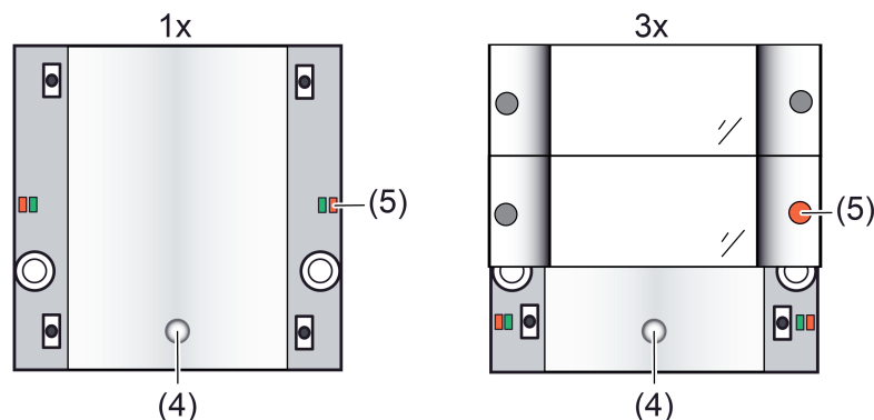
Bild 4: Programmier-Taste hinter der Wippenabdeckung (links: 1fach / rechts: 3fach)
