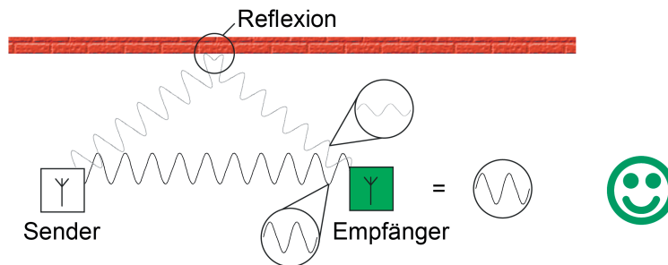
Bild 31: Interferenz beim Empfänger wirkungslos
