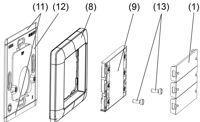
Bild 3: Klebmontage
