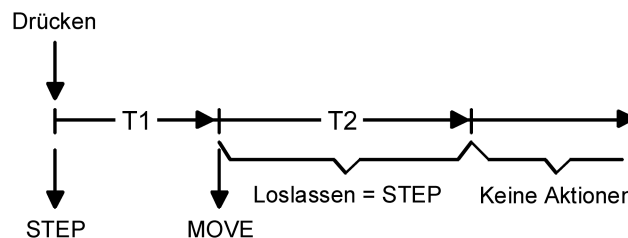
Bild 22: Bedienkonzept "Kurz-Lang-Kurz"
