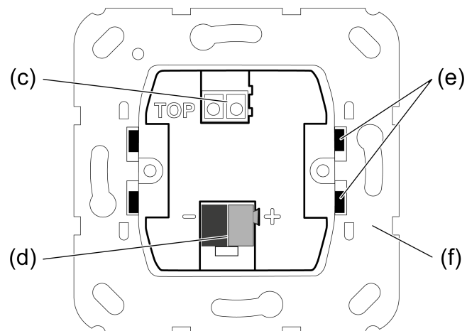
Bild 3: Geräteaufbau - Rückseite
