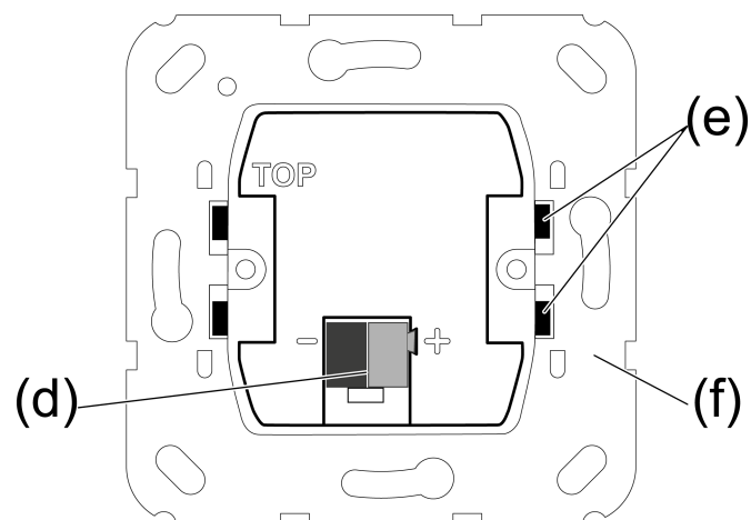
Bild 3: Geräteaufbau - Rückseite
