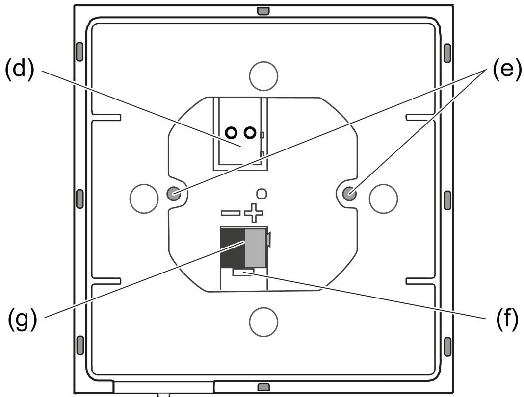
Bild 2: Geräteaufbau - Rückseite
