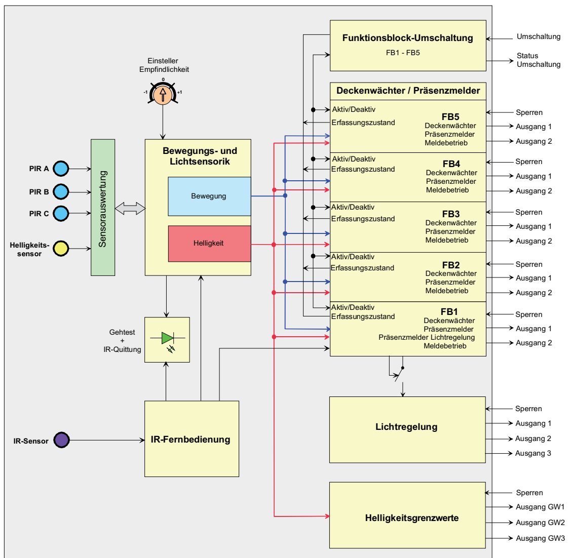
Bild 15: Blockschaltbild aller Funktionen des Geräts
