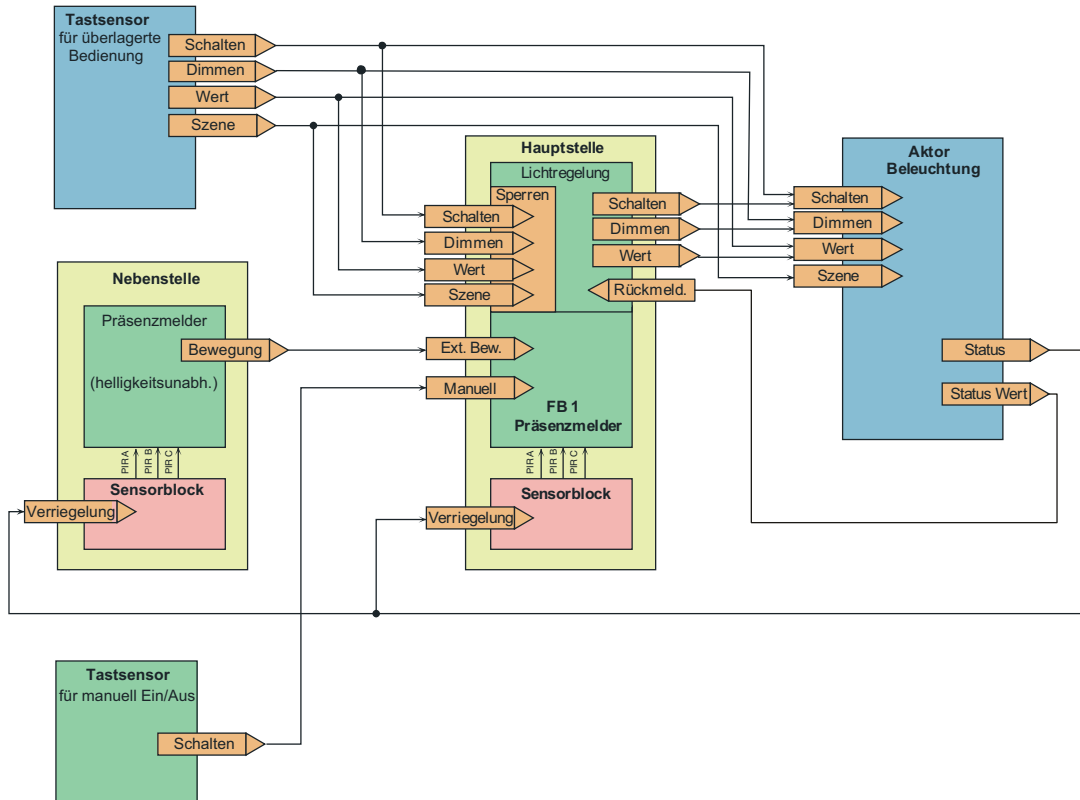
Bild 61: Applikationsbeispiel 1
