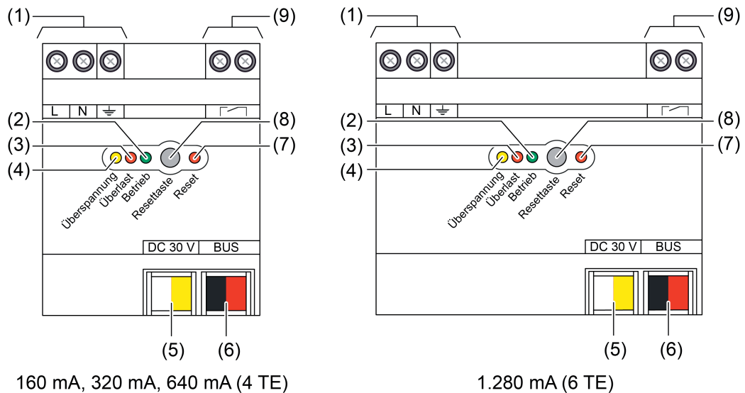
Bild 1: Geräteaufbau
