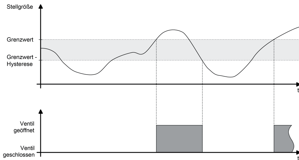
Bild 17: Beispiel einer Stellgrößenauswertung mit Grenzwert
