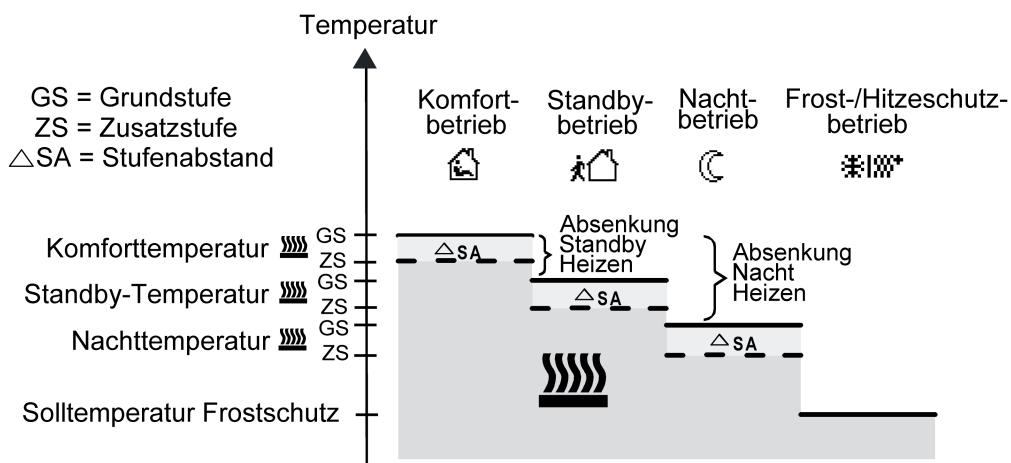
Bild 44: Solltemperaturen in der Betriebsart "Grund- und Zusatzheizen"
