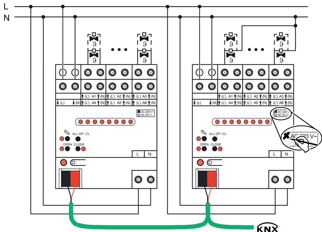
Bild 2: Anschluss für Stellantriebe AC 230 V (Anschlussbeispiele) links: Neutralleiter der Stellantriebe separat zum Aktor geführt / rechts: Gemeinsamer Neutralleiter für Stellantriebe
