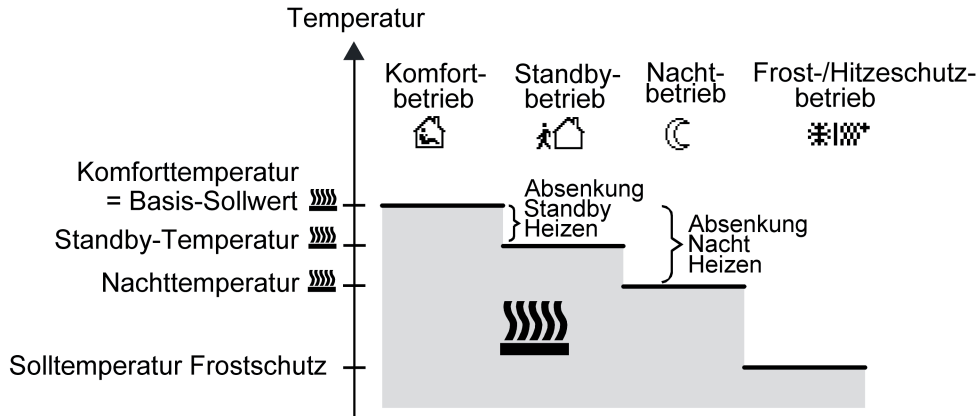
Bild 43: Solltemperaturen in der Betriebsart "Heizen"
