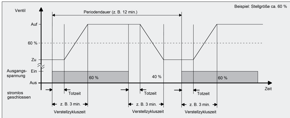
Bild 5: Idealisierter Verlauf des Ventilhubes exemplarisch dargestellt für eine Zykluszeit > 2 x Verstellzykluszeit
