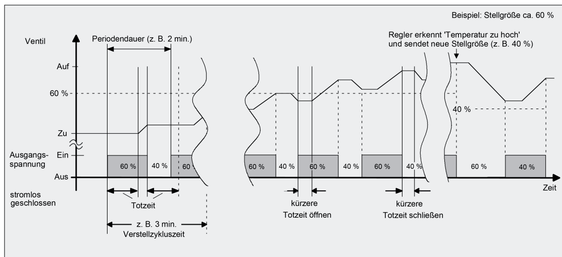
Bild 6: Idealisierter Verlauf des Ventilhubes exemplarisch dargestellt für eine Zykluszeit < Verstellzykluszeit
