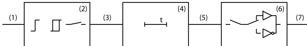
Bild 29: Blockdiagramm Ein- und Ausschaltverzögerung
