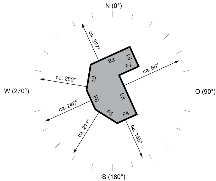
Bild 20: Fassadenausrichtung eines Gebäudes mit 8 Fassaden
