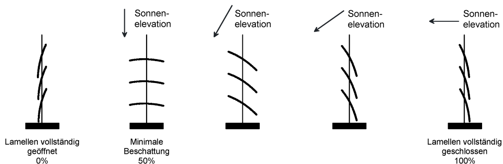
Bild 21: Lamellen werden abhängig vom Sonnenstand positioniert
