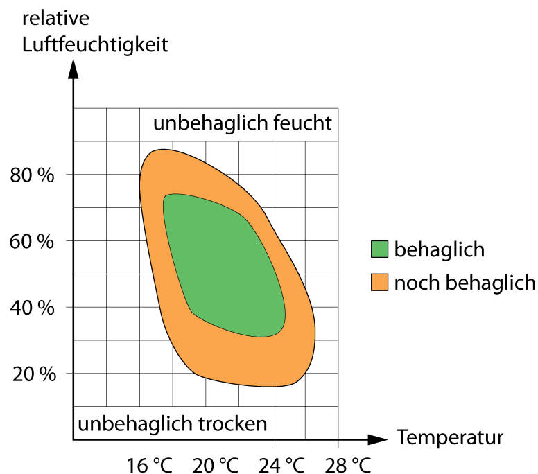
Bild 24: Behaglichkeitskurve
