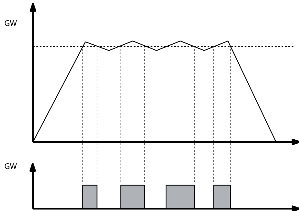
Bild 26: Schalthäufigkeit ohne Hysterese
