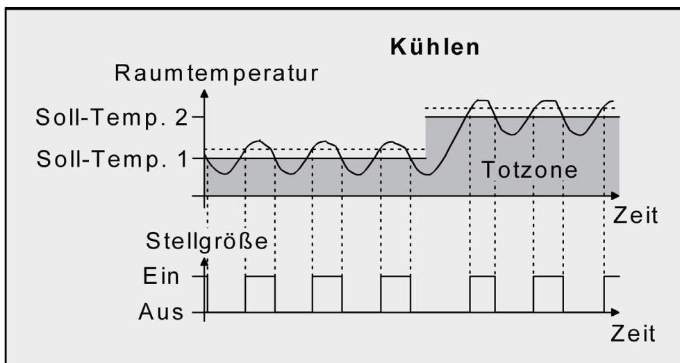
Bild 37: 2-Punkt-Regelung für Mischbetriebsart „Heizen und Kühlen“ bei aktivem Kühlbetrieb
