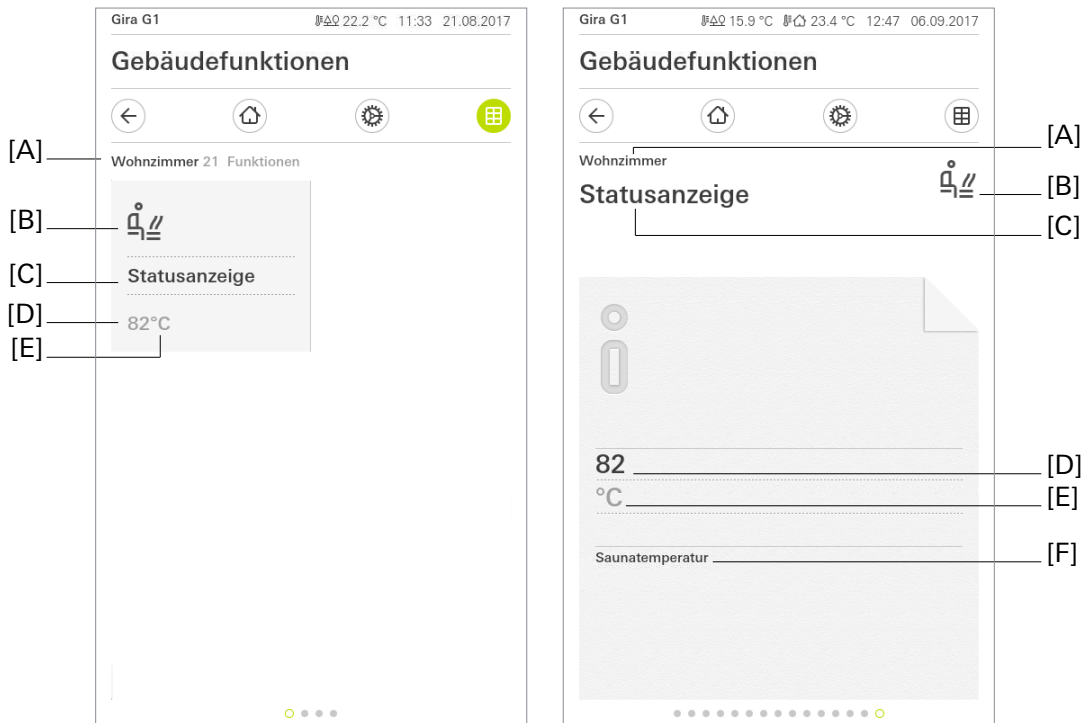
Bild 24: Beispiel für Bedien- und Anzeigeelement der Funktion „Statusanzeige“
