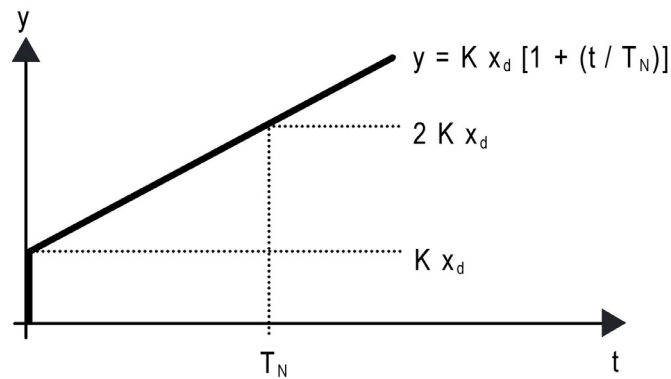
Bild 38: Funktion der Stellgröße einer PI-Regelung
