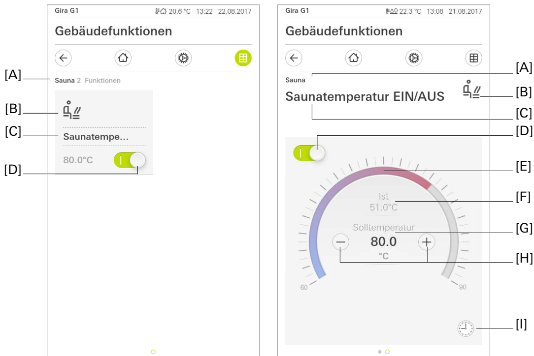
Bild 19: Beispiel für Bedien- und Anzeigeelement der Funktion „Saunatemperatur EIN/AUS“
