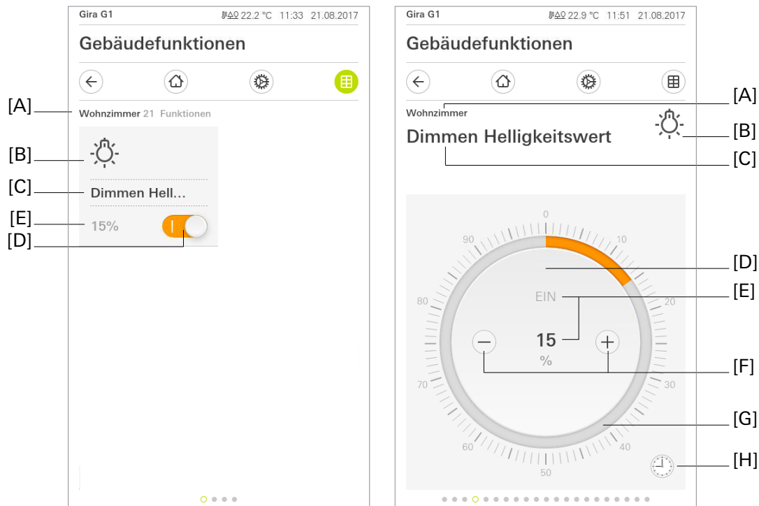
Bild 5: Beispiel für Bedien- und Anzeigeelement der Funktion „Dimmen Helligkeitswert“
