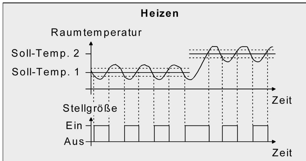
Bild 34: 2-Punkt-Regelung für Betriebsart „Heizen“
