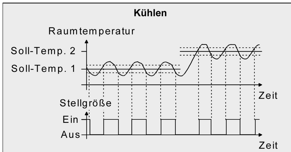
Bild 35: 2-Punkt-Regelung für Betriebsart „Kühlen“
