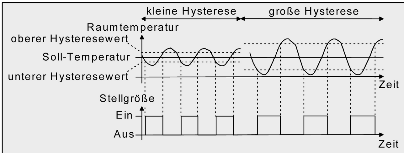
Bild 39: Auswirkungen der Hysterese auf das Schaltverhalten der Stellgröße einer 2-Punkt-Regelung
