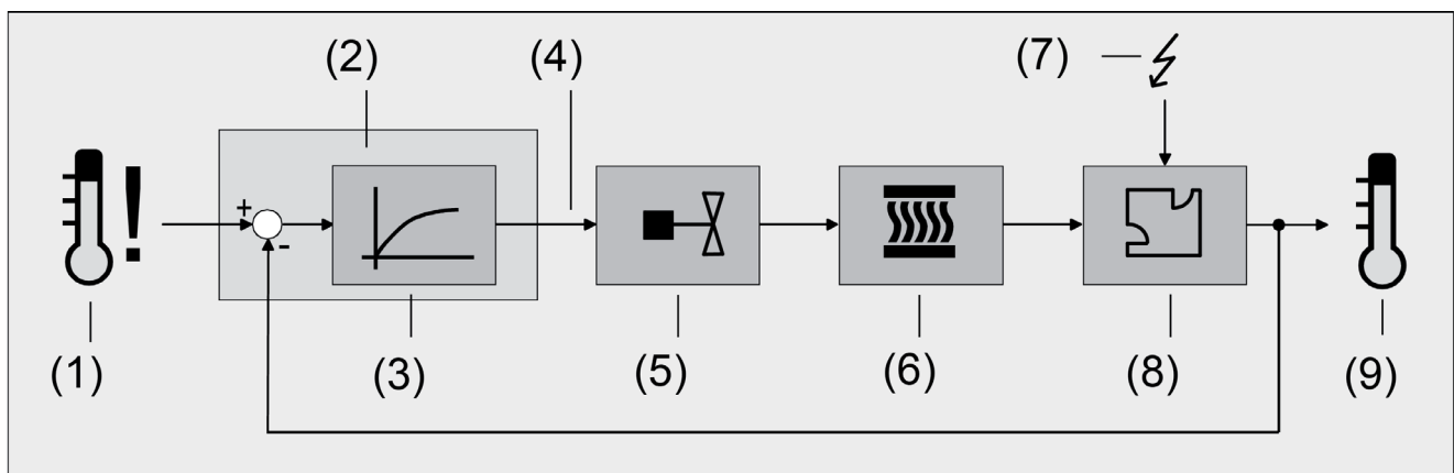
Bild 31: Regelstrecke einer Einzelraum-Temperaturregelung
