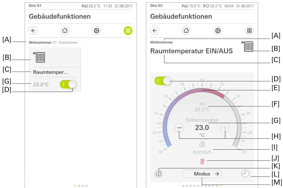
Bild 17: Beispiel für Bedien- und Anzeigeelement der Funktion „Raumtemperatur EIN/AUS“
