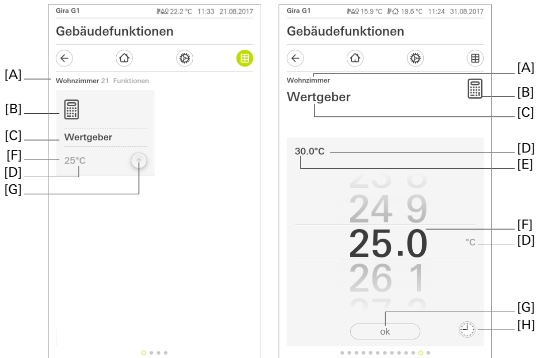
Bild 22: Beispiel für Bedien- und Anzeigeelement der Funktion „Wertgeber (Walze)“
