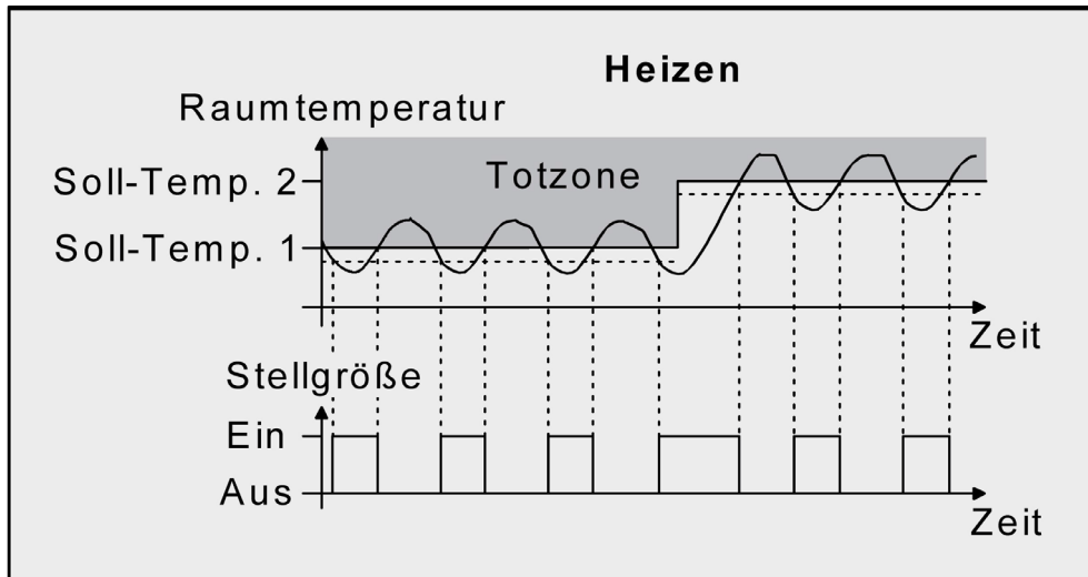
Bild 36: 2-Punkt-Regelung für Mischbetriebsart „Heizen und Kühlen“ bei aktivem Heizbetrieb
