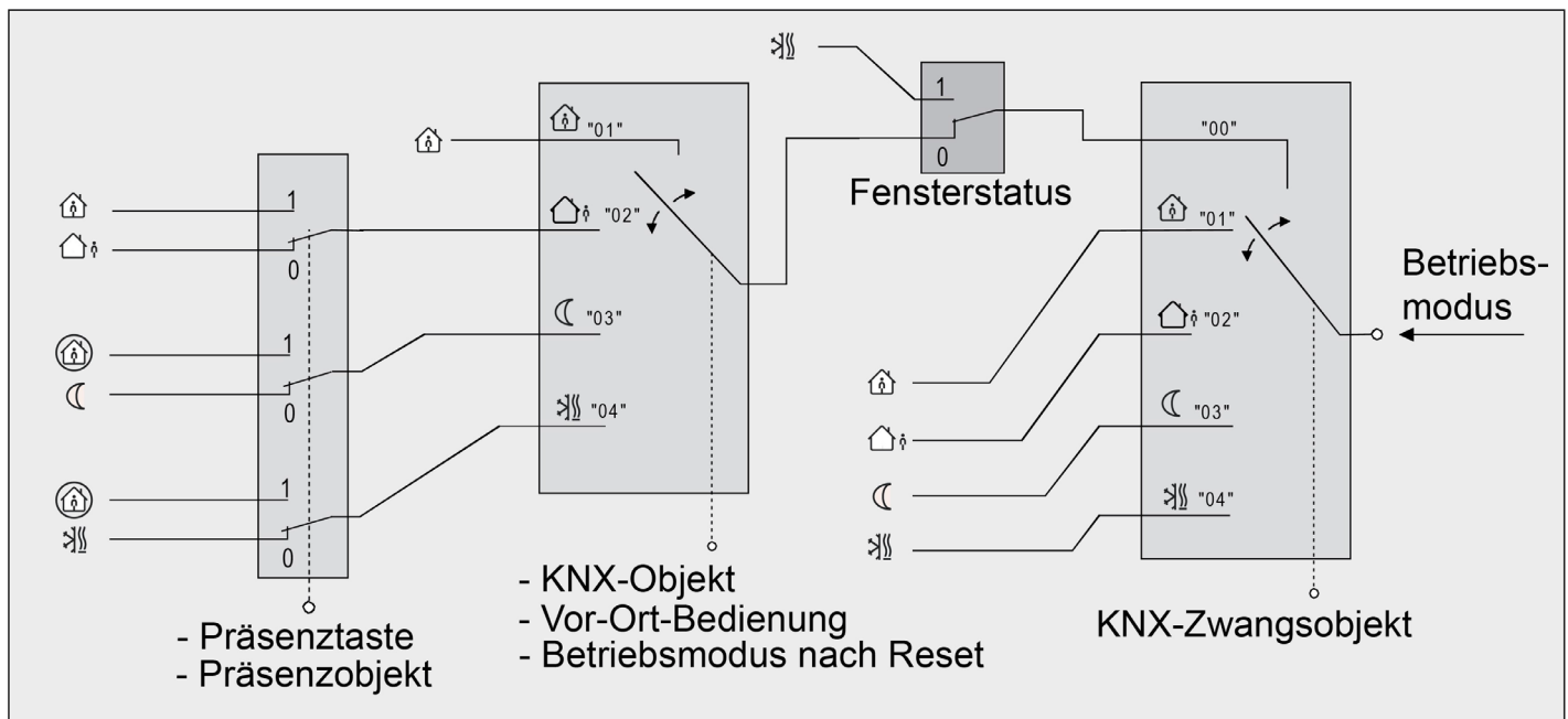
Bild 40: Betriebsmodusumschaltung durch KNX Objekt mit Präsenztaste
