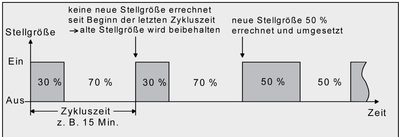
Bild 33: Schaltende PI-Regelung
