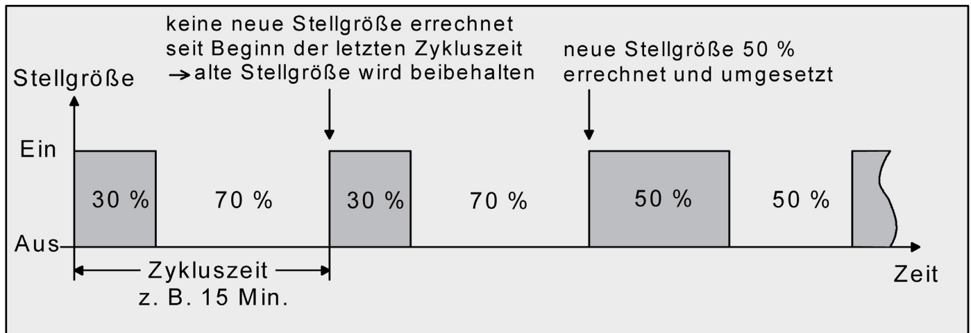
Bild 32: Schaltende PI-Regelung
