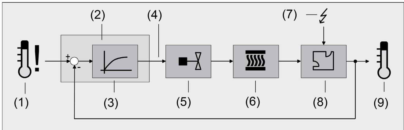
Bild 30: Regelstrecke einer Einzelraum-Temperaturregelung
