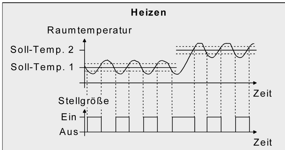
Bild 33: 2-Punkt-Regelung für Betriebsart „Heizen“
