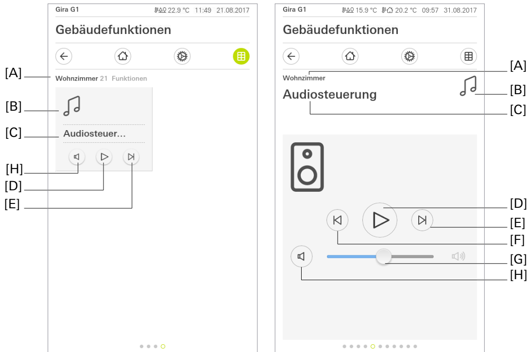
Bild 26: Beispiel für Bedien- und Anzeigeelement der Funktion „Audiosteuerung“
