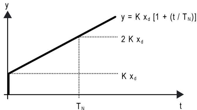
Bild 37: Funktion der Stellgröße einer PI-Regelung
