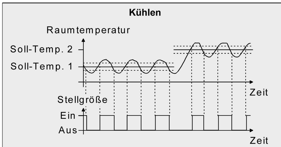
Bild 34: 2-Punkt-Regelung für Betriebsart „Kühlen“
