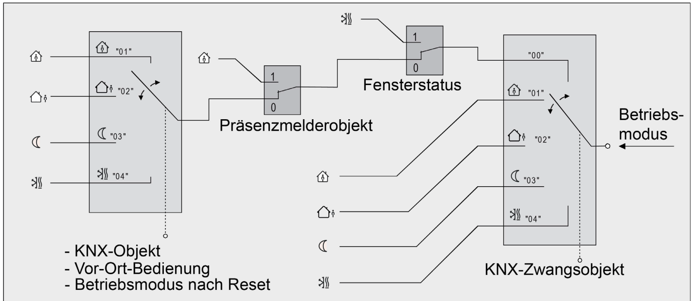
Bild 40: Betriebsmodusumschaltung durch KNX Objekt mit Präsenzmelder
