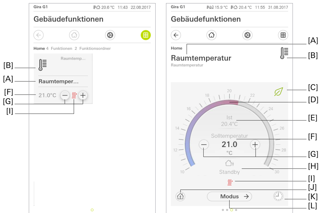
Bild 29: Beispiel für Bedien- und Anzeigeelement des Raumtemperaturreglers“
