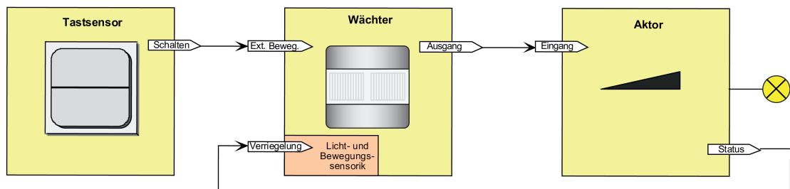
Bild 38: Applikationsbeispiel Einzelgerät mit externer Bewegungserfassung
