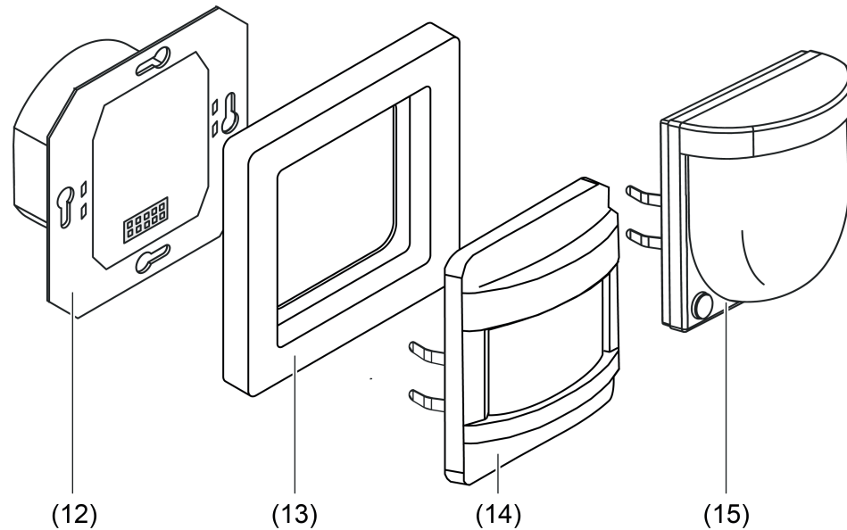
Bild 17: Montage
