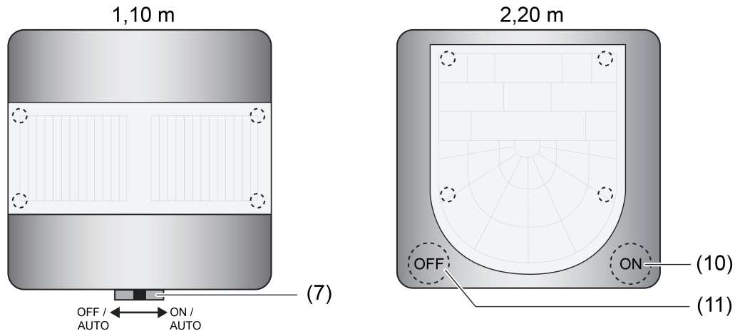
Bild 34: Anordnung der Bedienelemente zur Vor-Ort-Bedienung (Betriebsartenumschaltung)
