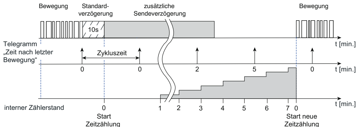
Bild 51: Messung der Zeitspanne nach letzter Bewegung
