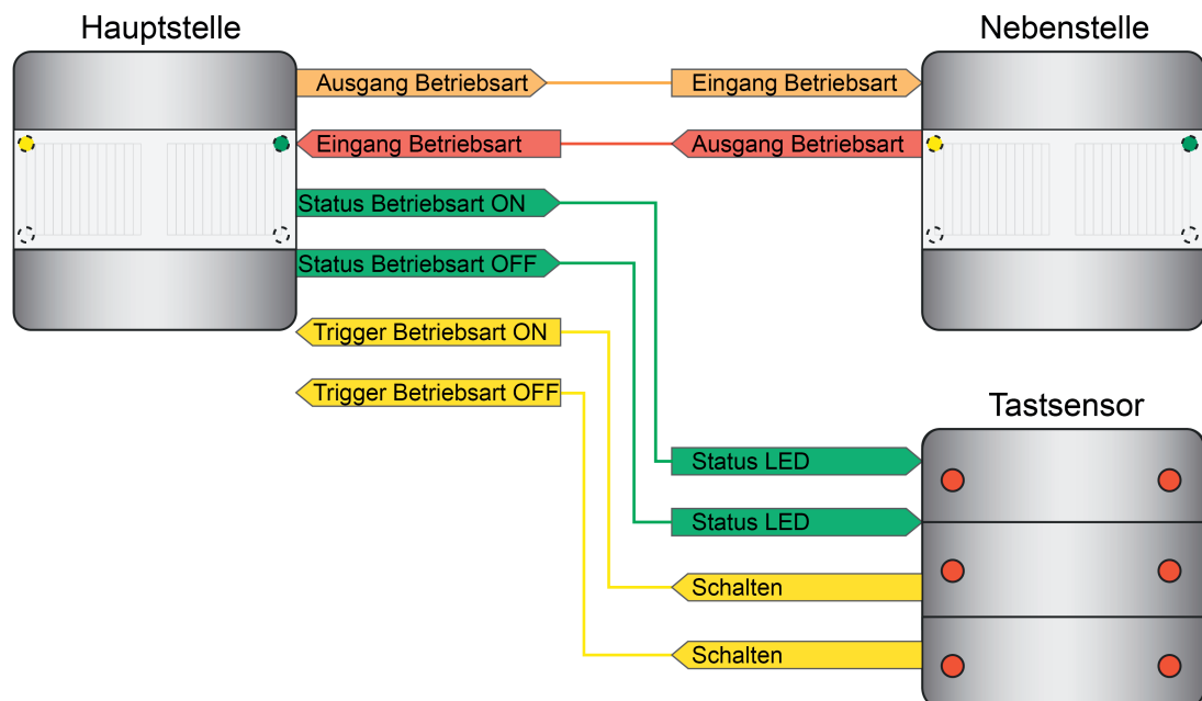
Bild 37: Beispiel zur Verknüpfung einer Hauptstelle mit einer Nebenstellen und einem Tastsensor zur Betriebsartenumschaltung und -anzeige
