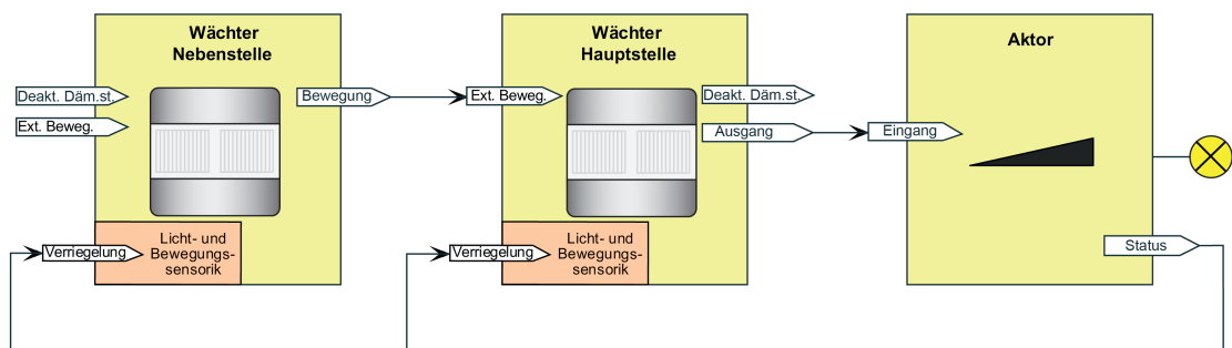
Bild 39: Applikationsbeispiel Haupt- und Nebenstelle ohne Dämmerungsstufenauswertung
