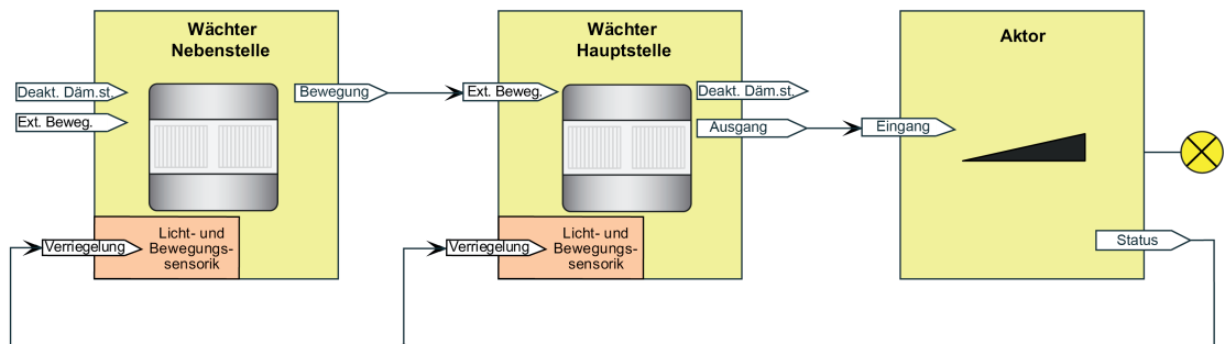
Bild 40: Applikationsbeispiel Haupt- und Nebenstelle mit Dämmerungsstufenauswertung in der Hauptstelle
