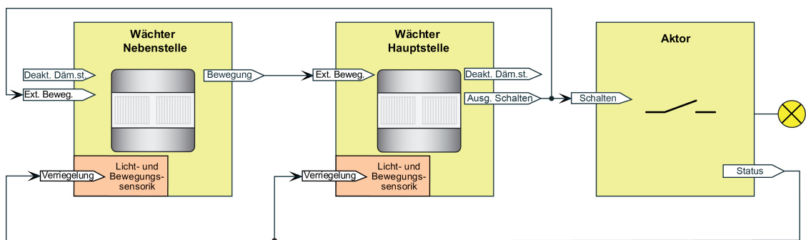
Bild 43: Applikationsbeispiel mit Dämmerungsstufenauswertung in der Hauptstelle und in den Nebenstellen für Ausgangsfunktion "Treppenhausfunktion"
