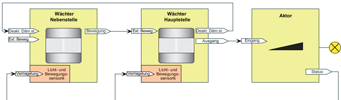
Bild 40: Applikationsbeispiel mit Dämmerungsstufenauswertung in der Hauptstelle und in den Nebenstellen Universal-Lösung für alle Datenformate
