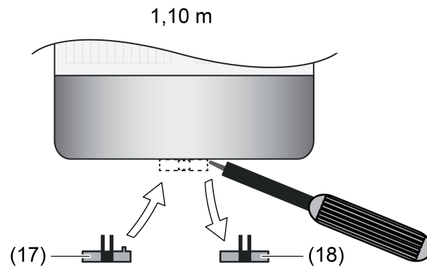
Bild 18: Arretierungsclip montieren
