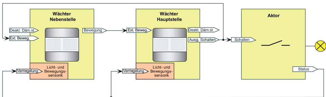
Bild 41: Applikationsbeispiel mit Dämmerungsstufenauswertung in der Hauptstelle und in den Nebenstellen für Ausgangsfunktion "Treppenhausfunktion"
