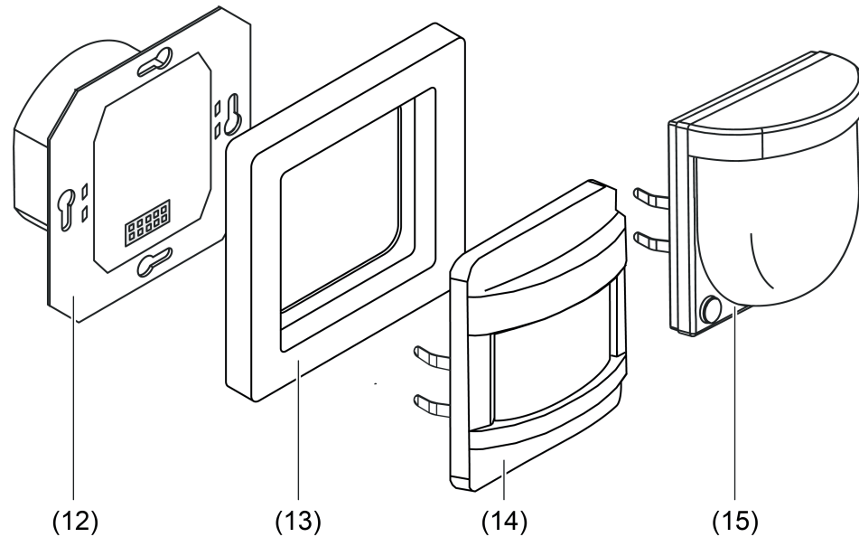
Bild 17: Montage
