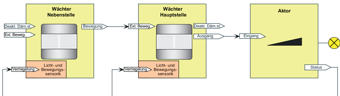
Bild 37: Applikationsbeispiel Haupt- und Nebenstelle ohne Dämmerungsstufenauswertung
