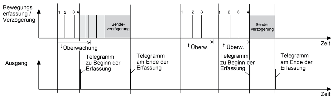
Bild 48: Bewegungsauswertung beim Melder
