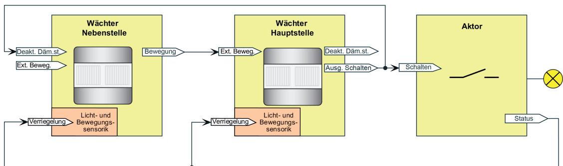
Bild 39: Applikationsbeispiel mit Dämmerungsstufenauswertung in der Hauptstelle und in den Nebenstellen für das Datenformat "Schalten"
