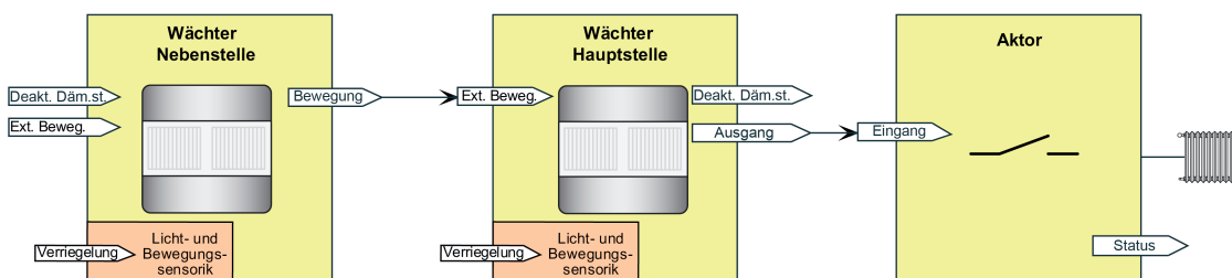
Bild 42: Applikationsbeispiel ohne Dämmerungsstufenauswertung in der Hauptstelle und in den Nebenstellen für Ausgangsfunktionen "Temperaturwertgeber" und "Betriebsmodus Raumtemperaturregler"
