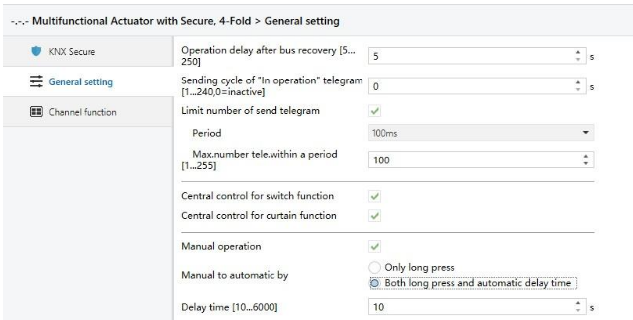
Fig. 4.2 Parameter window “General”
