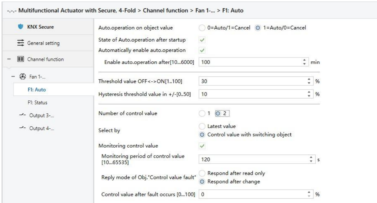
Fig. 4.8.1.1 Parameter window “Fx: Auto.”
