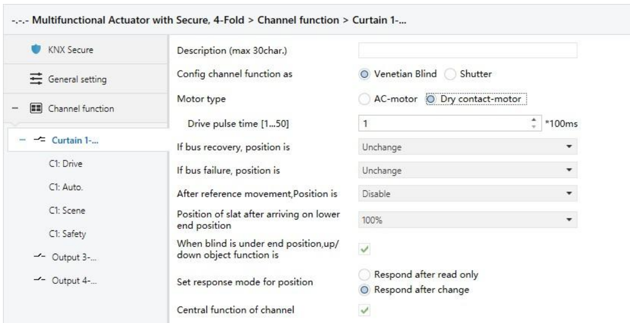
Fig. 4.6.1 Parameter window “Curtain X: Venetian Blind”
