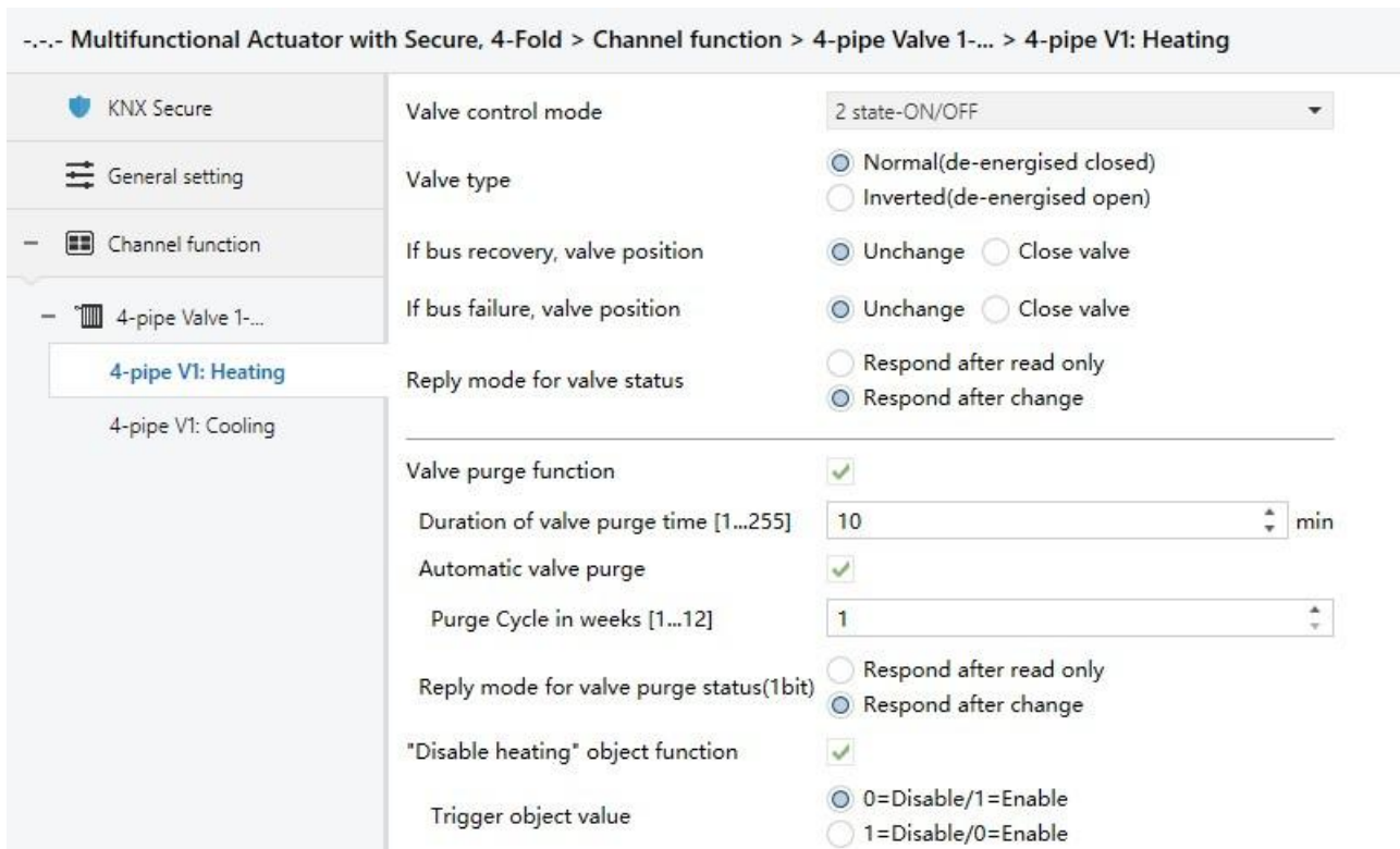
Fig. 4.9.1.1 Parameter window “2 state-ON/OFF”
