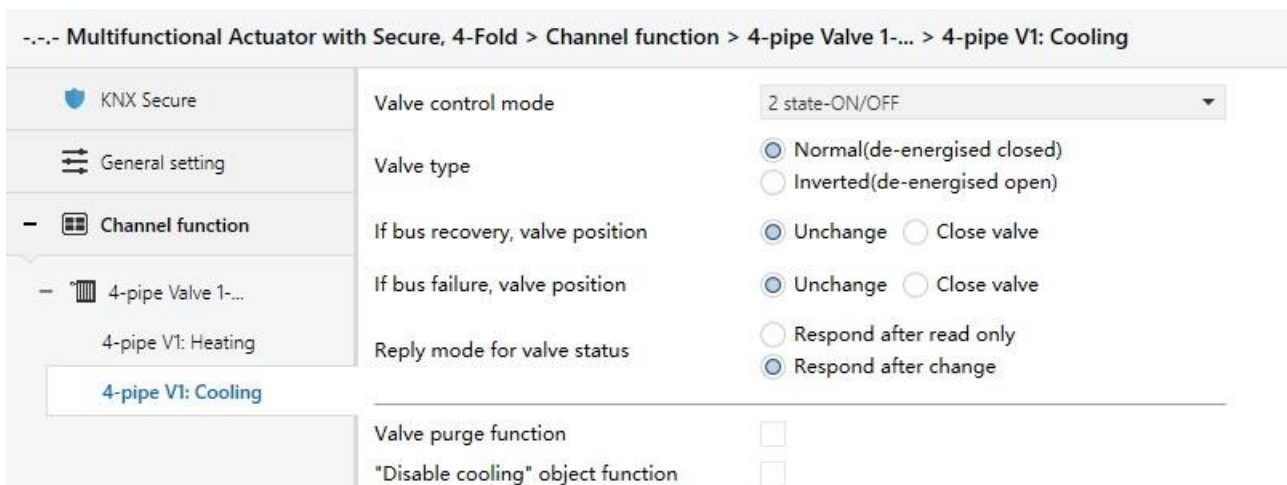
Fig. 4.9.1(2) Parameter window “Vx: Cooling”
