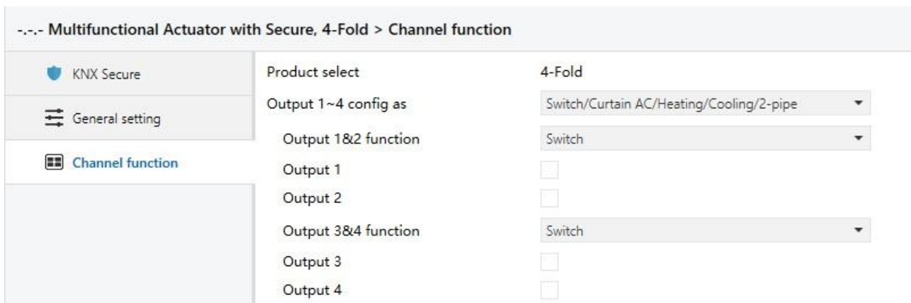
Fig. 4.3 Parameter window "Channel function"
