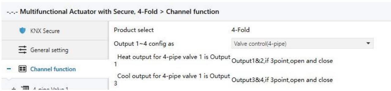
Fig. 4.9(1) Parameter window Channel function--valve type”
