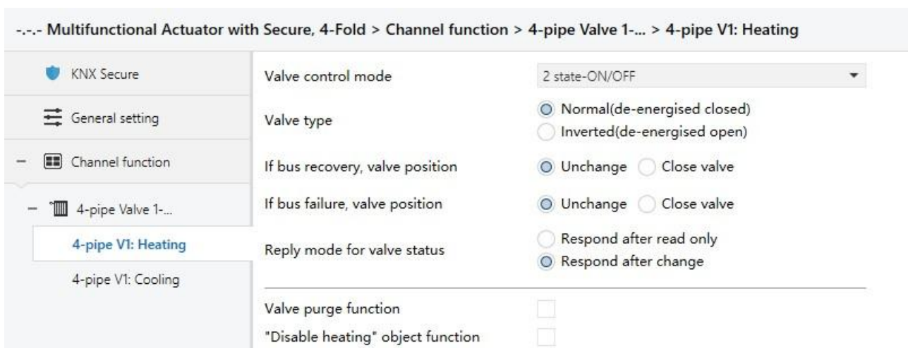
Fig. 4.9.1(1) Parameter window “Vx: Heating”
