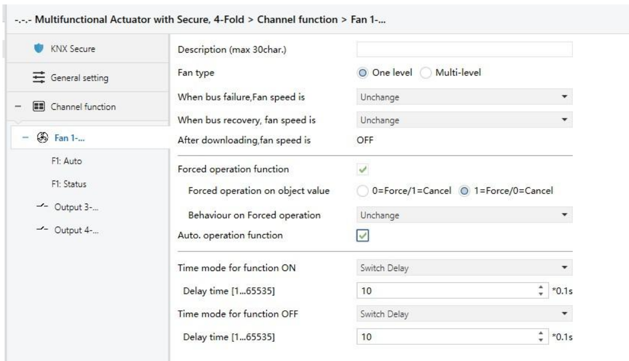
FIG. 4.8.1 Parameter window “Fan type -- One level”
