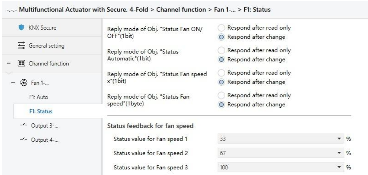
Fig. 4.8.2.2 Parameter window “Fx: Status”
