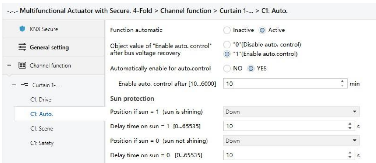
Fig. 4.6.1.2 Parameter window “Cx: Auto.”
