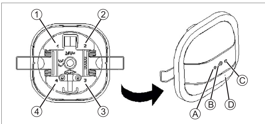
Abb. 1: Produktübersicht
