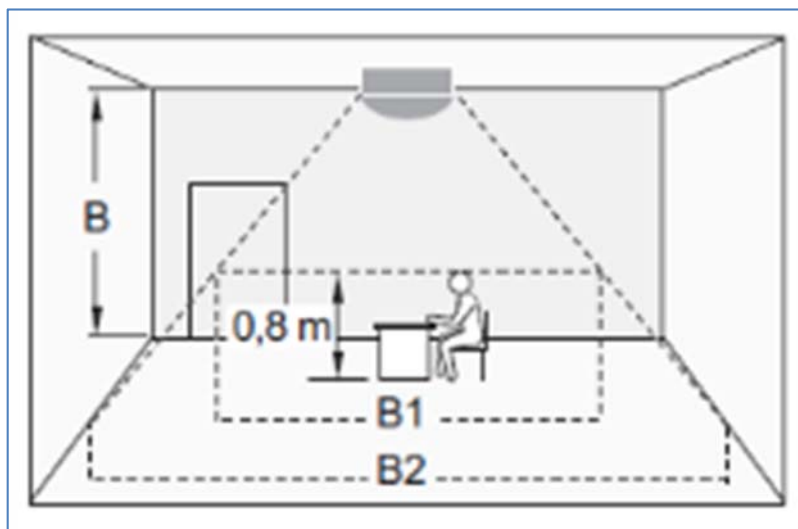
Abb. 11: Erfassungsbereiche Busch-Präsenzmelder Mini KNX / Busch-PräsenzmelderMini Premium KNX
