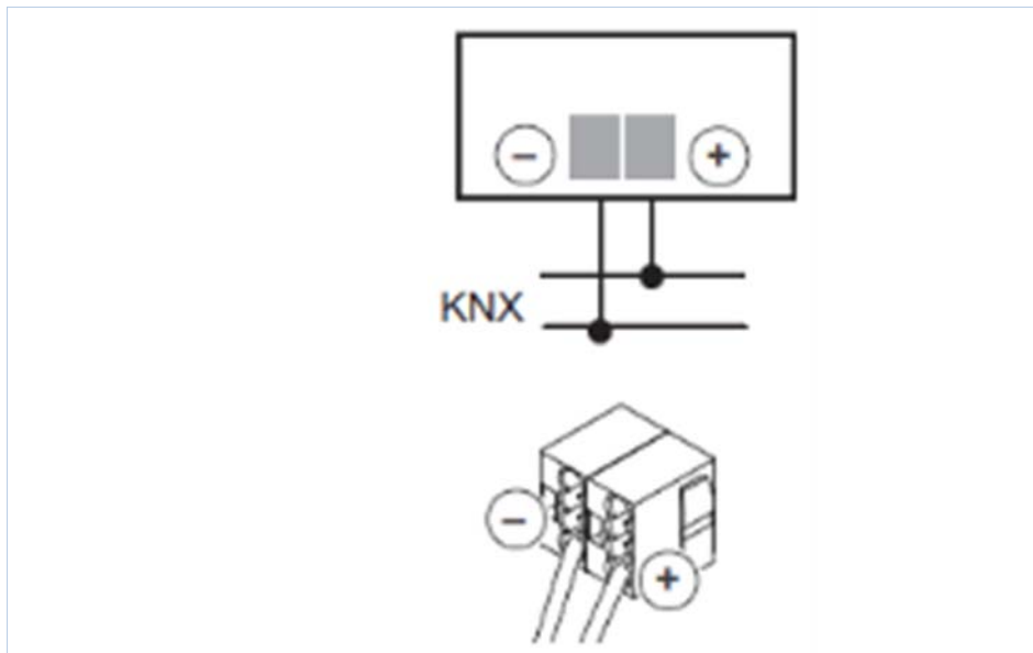
Abb. 10: Elektrischer Anschluss
