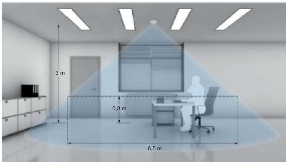
Abb. 5: Innerer Erfassungsbereich
