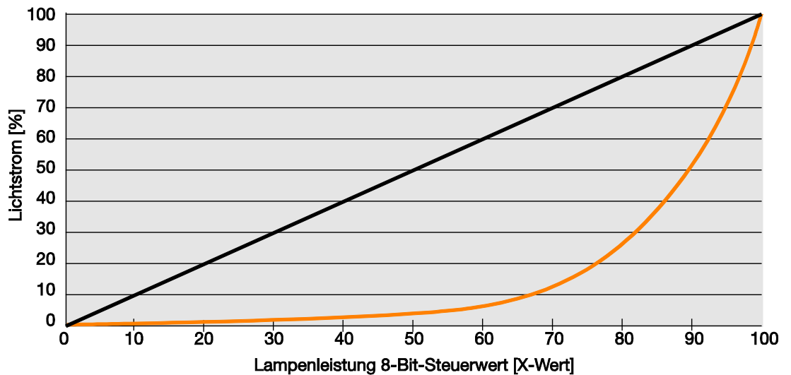
Unkompensierte DALI Kennlinie für Steuerwert [0...100 %]
