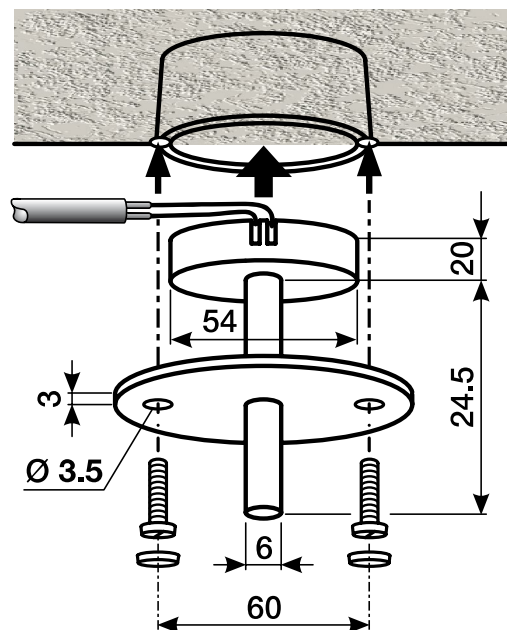
Maßbild 6197/71
