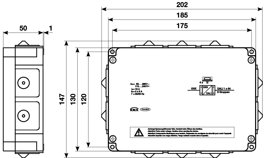
Maßbild 6174/40
