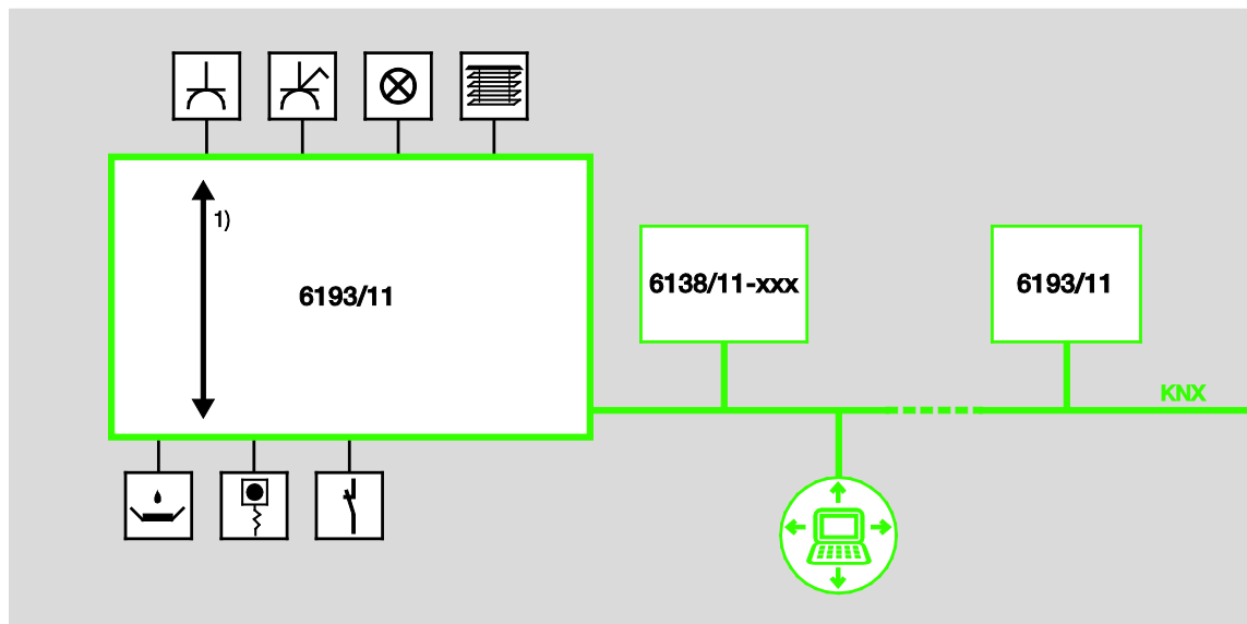
1 Interne Geräteverbindungen
