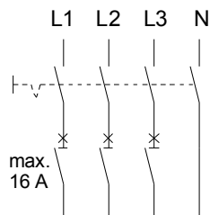
Leitungsschutz der einzelnen Phasen sowie Trennschalter zum Freischalten der Spannung
