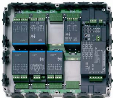
6174/10 (offen)
