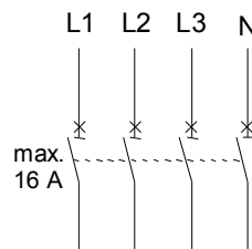
allpolig abschaltender Sicherungsautomat
