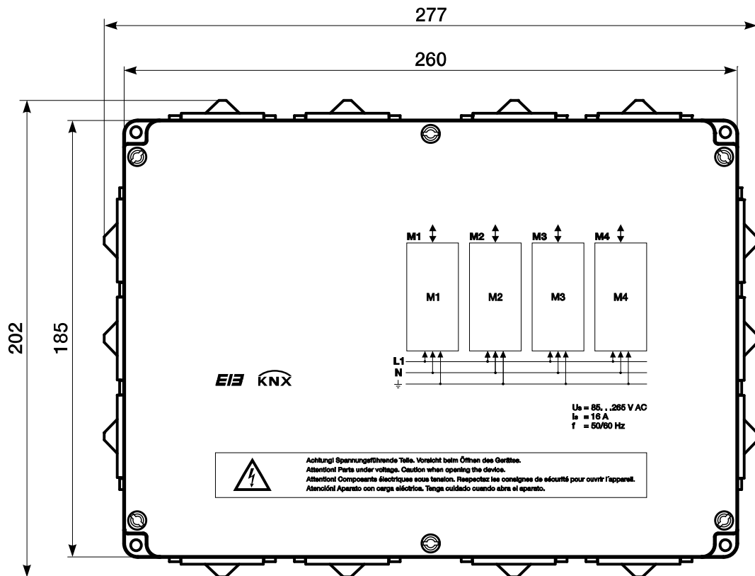
Maßbild 6174/09
