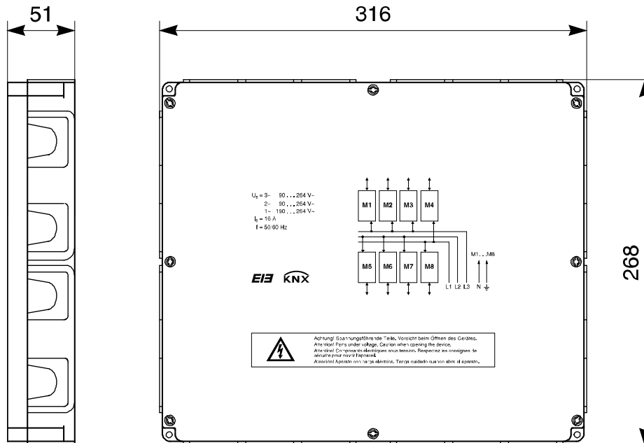
Maßbild 6174/10
