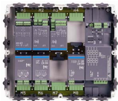
6174/10-101 (offen)
