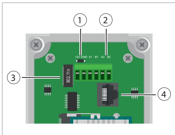
Abb. 20: Elektrischer Anschluss und Schnittstellen
