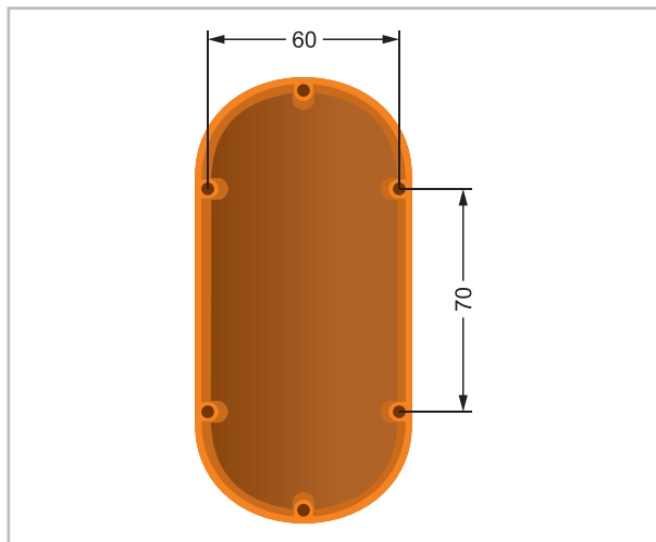
Abb. 27: Doppeldose
