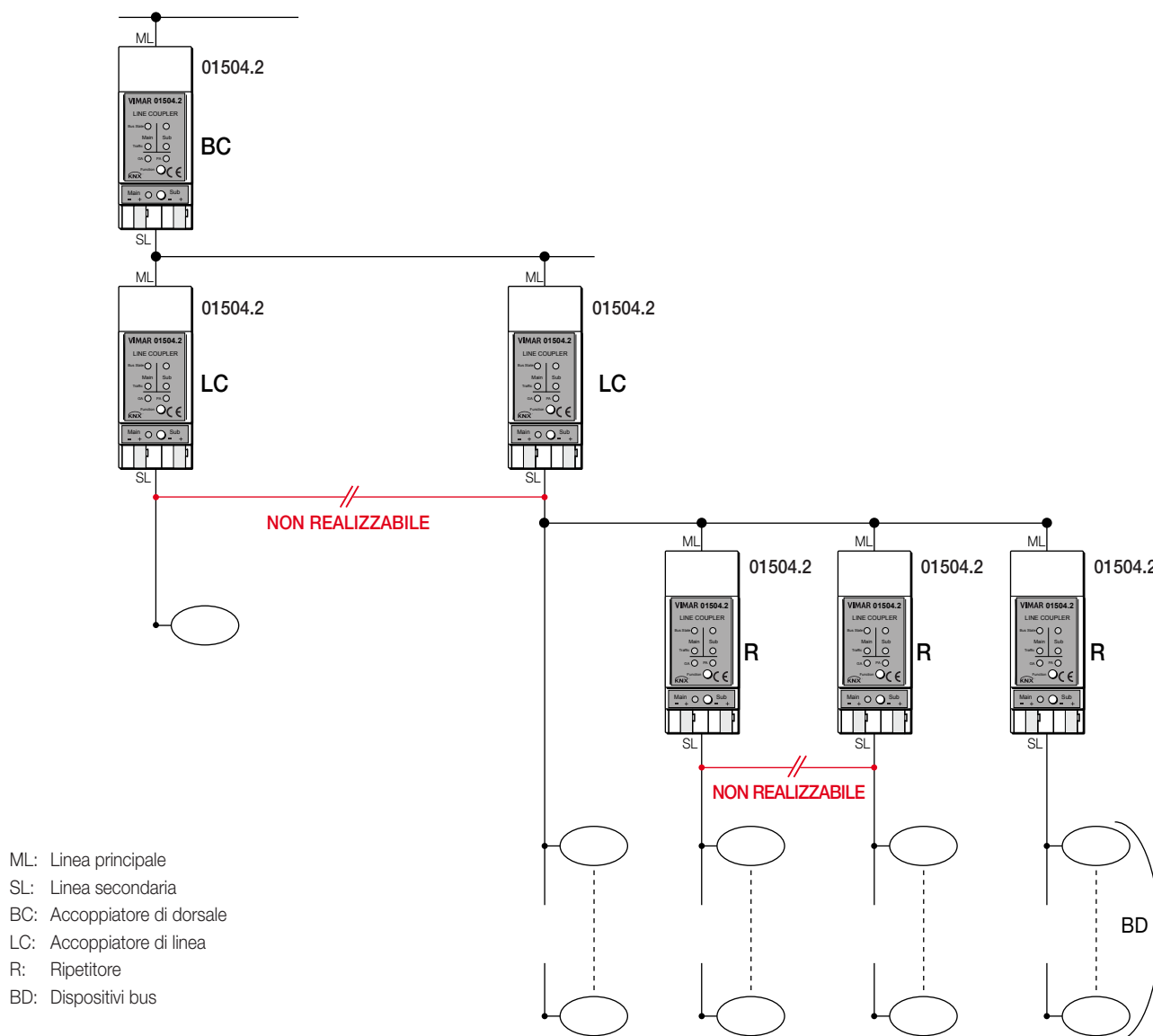
Fig. 1: Topologia
