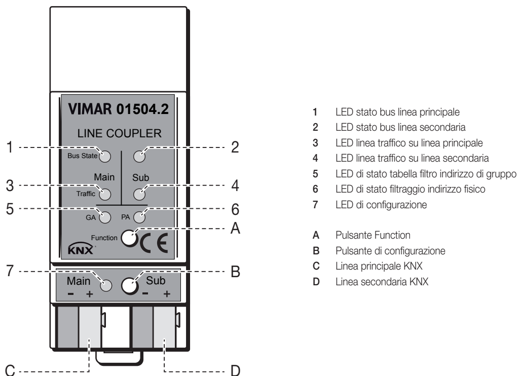
Fig. 2: Vista frontale
