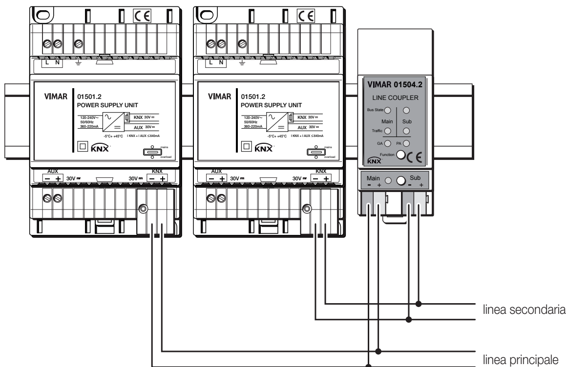
Fig. 3: Collegamento
