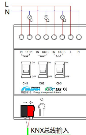
接线图
