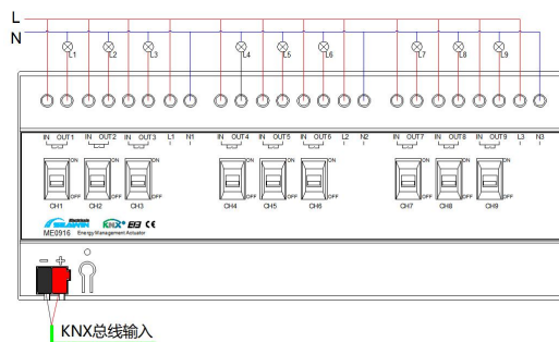
接线图
