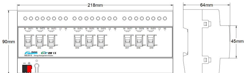
尺寸图
