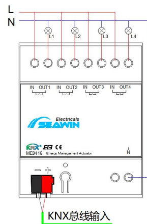
接线图
