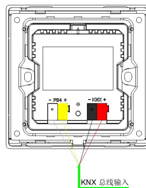
TC0203/TC0303 接线图
