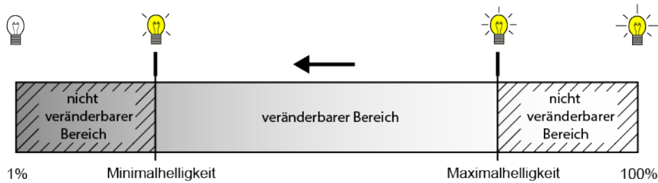
Bild 40: Helligkeitsdurchlauf Richtung "dunkler"
