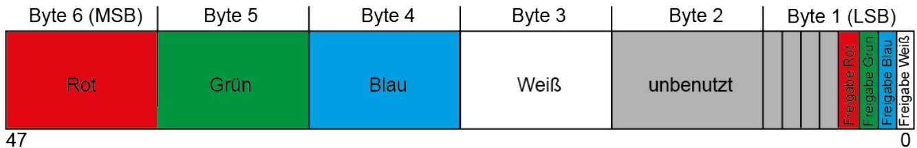
Bild 31: KNX Datentyp "RGBW kombiniert" (DPT 251.600)
