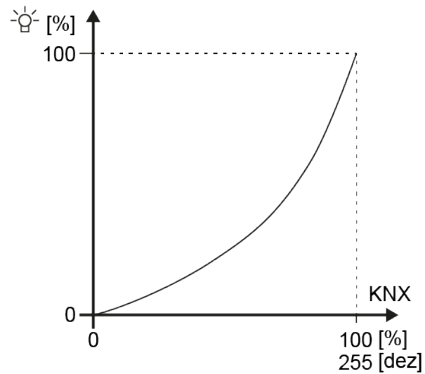
Bild 20: Kombinierte Dimmkennlinie am Ausgang eines Betriebsgeräts (relativer Lichtstrom [%] abhängig vom 8-Bit-KNX Datenwert [0...255])
