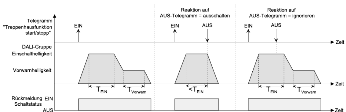
Bild 50: Ausschaltverhalten der Treppenhausfunktion mit Soft-Funktionen (als Beispiel mit Minimalhelligkeit = 0%)
