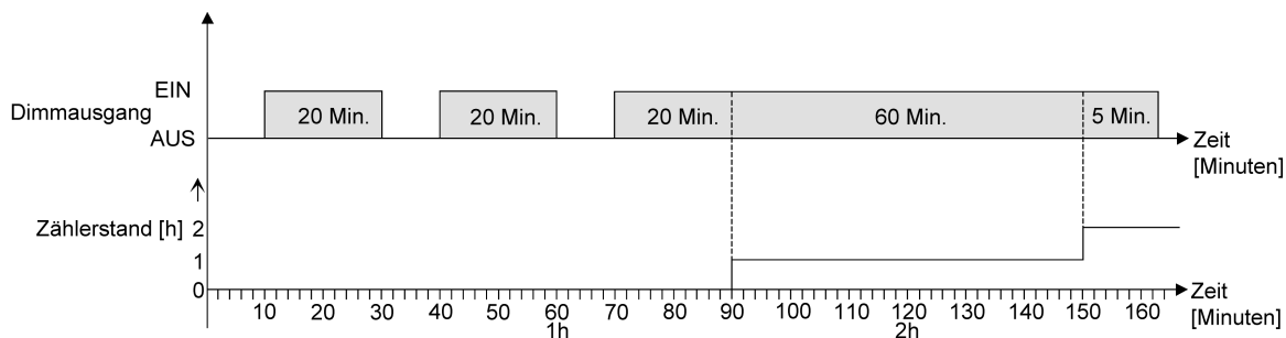
Bild 56: Funktionsweise des Betriebsstundenzählers (am Beispiel gezählter Stunden)
