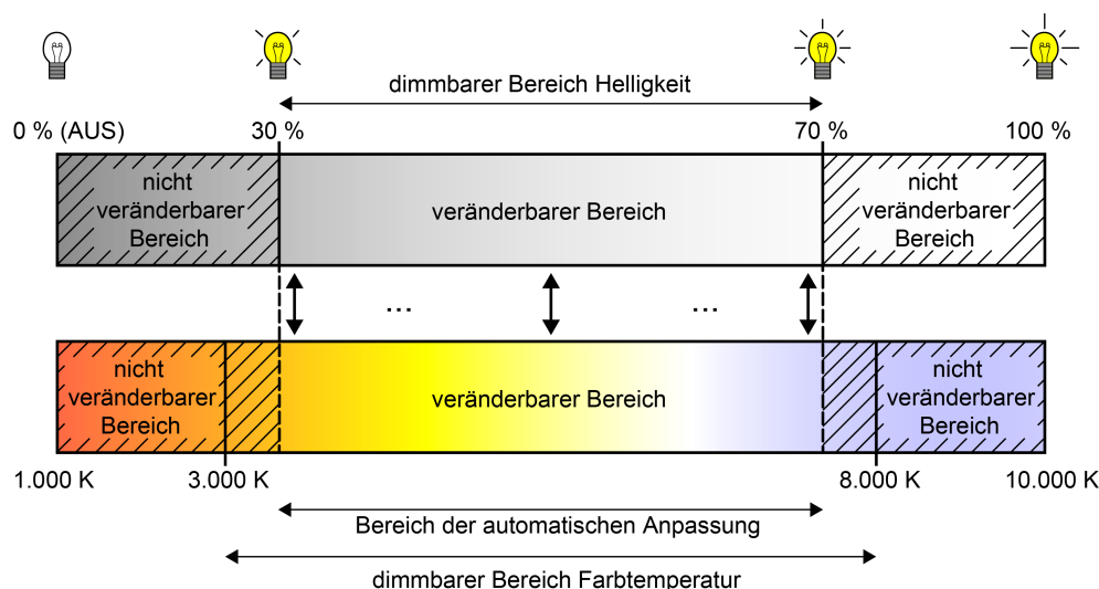
Bild 24: Automatische Anpassung der Farbtemperatur an die eingestellte Helligkeit Beispiel mit eingeschränktem Helligkeits- und Farbtemperaturbereich
