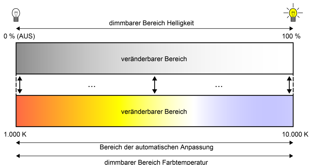
Bild 23: Automatische Anpassung der Farbtemperatur an die eingestellte Helligkeit Beispiel im maximalen Helligkeits- und Farbtemperaturbereich
