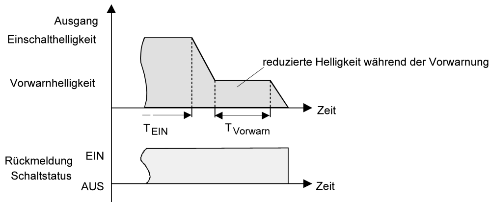
Bild 52: Die Vorwarnfunktion der Treppenhausfunktion mit Soft-AUS-Funktion (als Beispiel mit Minimalhelligkeit = 0%)
