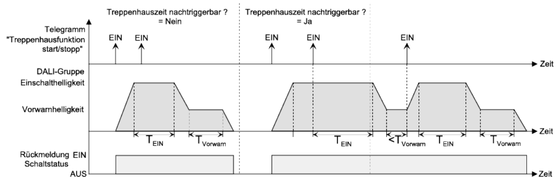
Bild 48: Einschaltverhalten der Treppenhausfunktion mit Soft-Funktionen (als Beispiel mit Minimalhelligkeit = 0%)
