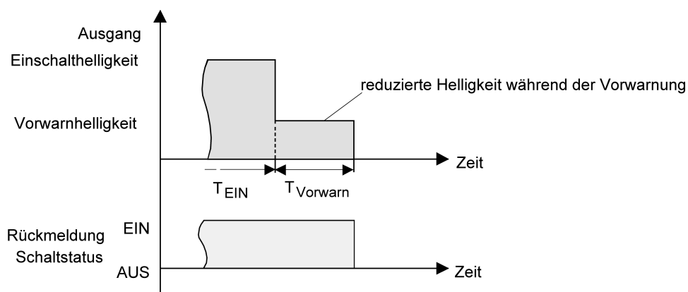
Bild 51: Die Vorwarnfunktion der Treppenhausfunktion ohne Soft-AUS-Funktion
