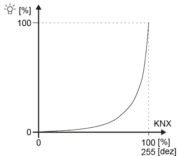
Bild 19: Logarithmische Dimmkennlinie am Ausgang eines Betriebsgeräts (relativer Lichtstrom [%] abhängig vom 8-Bit-KNX Datenwert [0...255])
