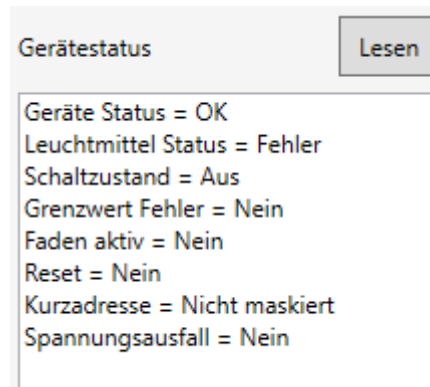
Bild 78: Beispiel für Gerätestatus
