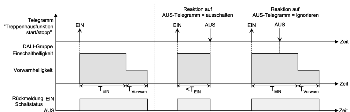
Bild 49: Ausschaltverhalten der Treppenhausfunktion ohne Soft-Funktionen
