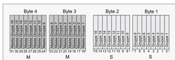
Bild 11: Struktur der Objekte der Sammelrückmeldung am Beispiel des Objekts für die Gruppen 1-16
