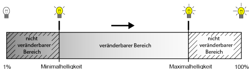
Bild 39: Helligkeitsdurchlauf Richtung "heller"
