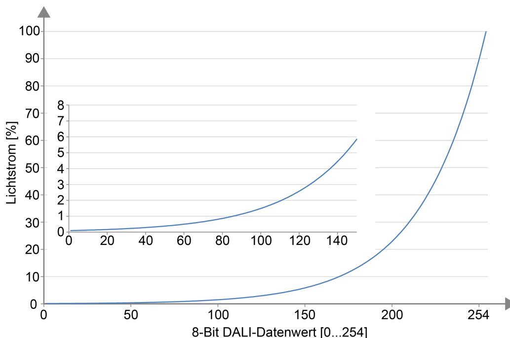
Bild 17: Logarithmische Dimmkurve in DALI-Betriebsgeräten (relativer Lichtstrom [%] abhängig vom 8-Bit-DALI-Datenwert [0...254])
