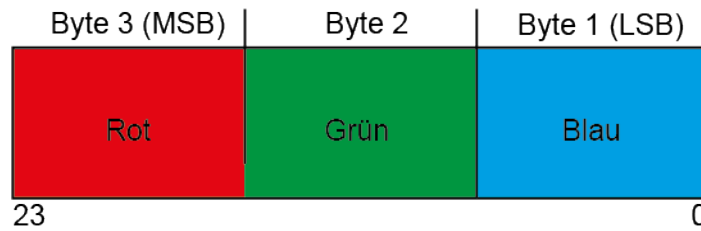
Bild 30: KNX Datentyp "RGB kombiniert" (DPT 232.600)
