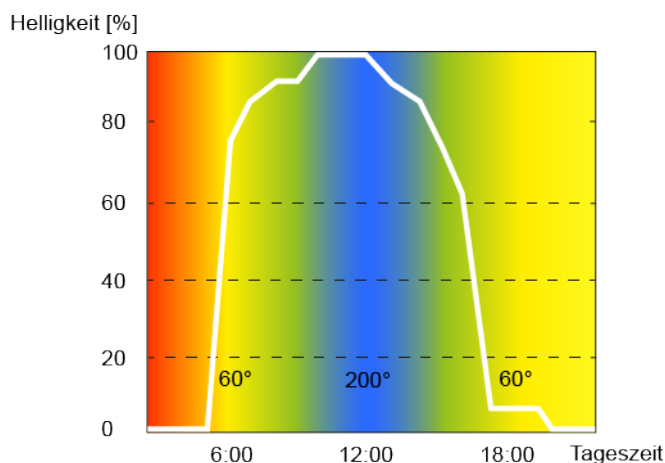
Bild 42: Beispielhafter Tagesfarbverlauf mit Farb- und Helligkeitsverstellung
