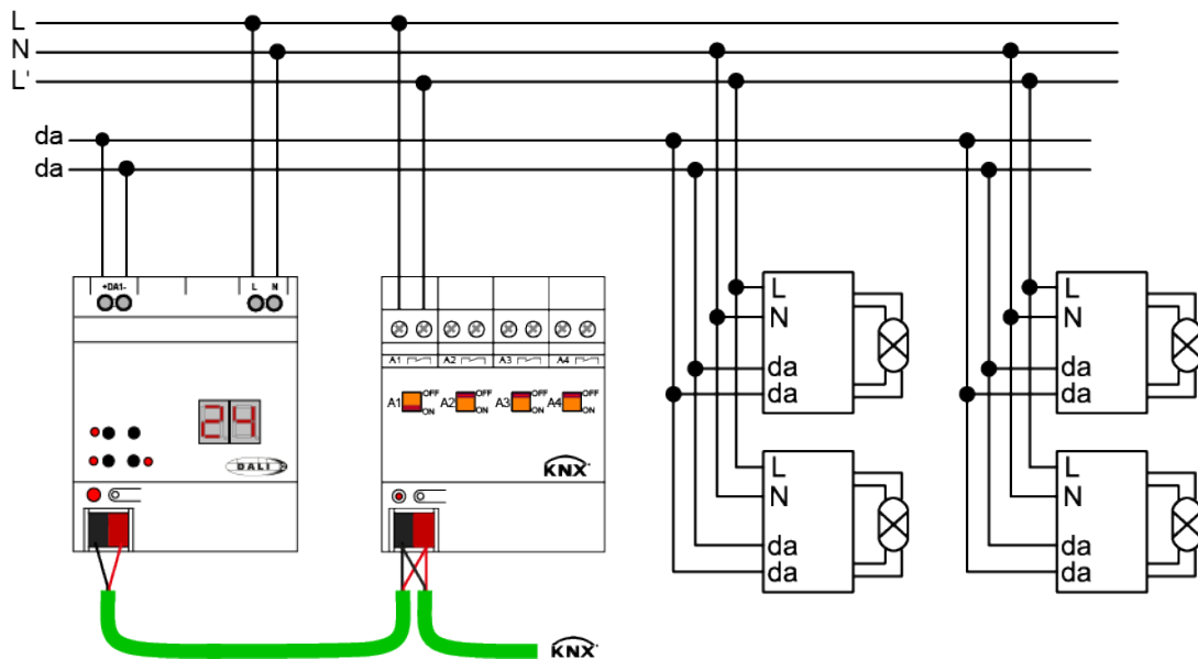
Bild 14: Beispiel eines Anschluss-Schemas zur Standby-Abschaltung durch einen KNX Schaltaktor
