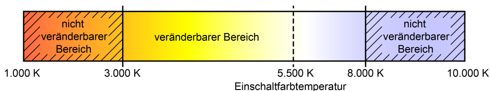
Bild 21: Beispiel eines konfigurierten Farbtemperaturbereichs mit Einschaltfarbtemperatur
