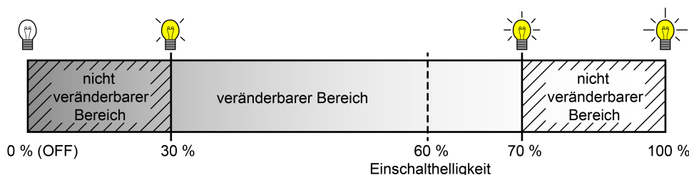
Bild 15: Beispiel eines Helligkeitsbereichs mit Einschalthelligkeit
