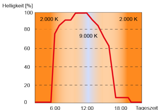
Bild 28: Beispielhafter Tagesfarbtemperaturverlauf "Gesundheit & Pflege"
