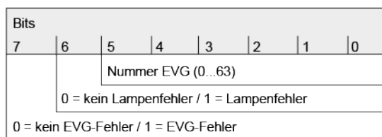
Bild 12: Telegrammaufbau 1-Byte-Fehlerstatus
