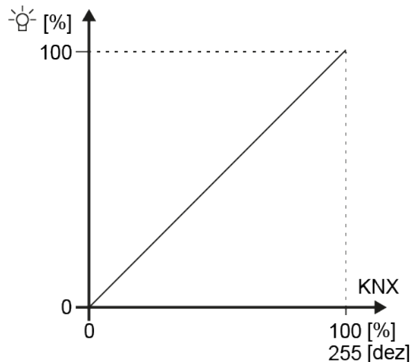
Bild 18: Lineare Dimmkennlinie am Ausgang eines Betriebsgeräts (relativer Lichtstrom [%] abhängig vom 8-Bit-KNX Datenwert [0...255])
