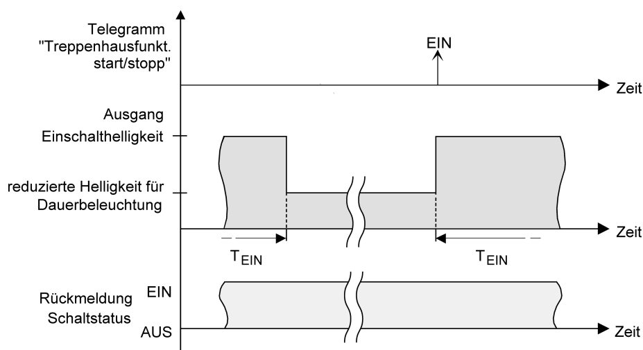
Bild 53: Die Dauerbeleuchtung der Treppenhausfunktion ohne Soft-Funktionen
