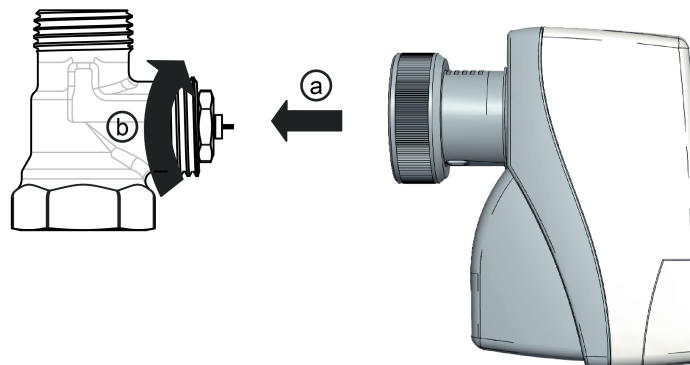
Bild 4: Gerät montieren
