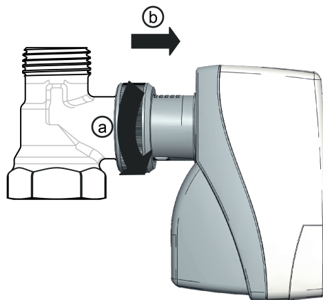
Bild 5: Gerät demontieren
