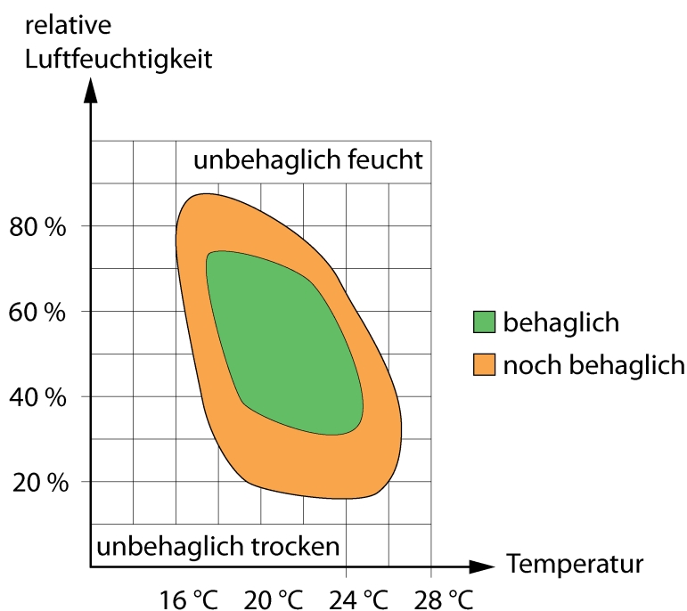
Bild 23: Behaglichkeitskurve
