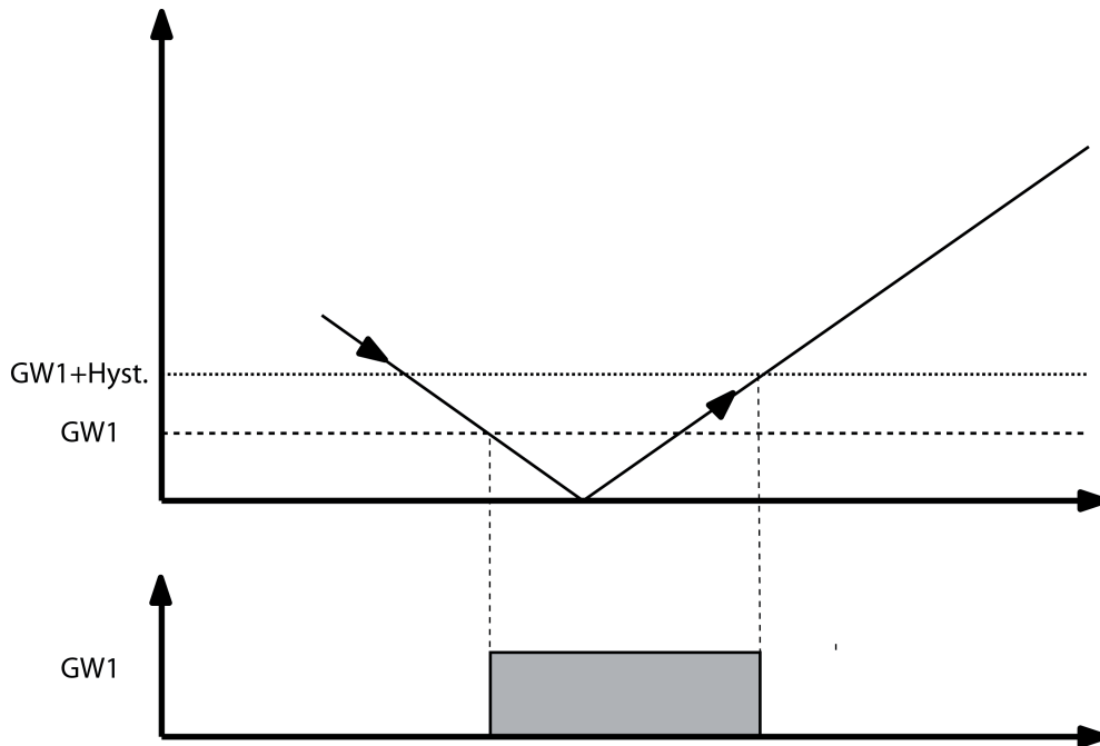
Bild 27: Aktivierung Grenzwert
