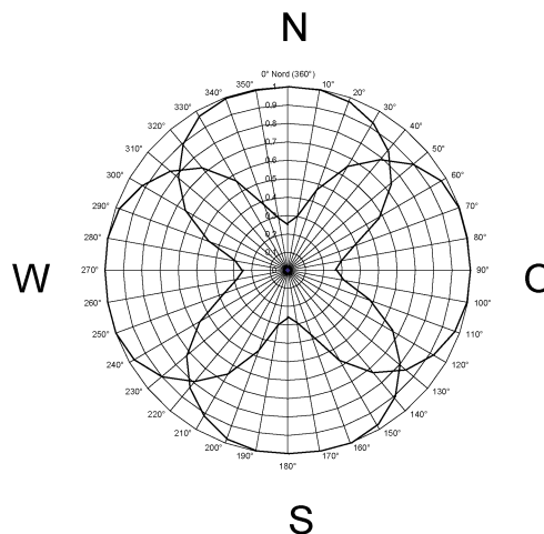
Bild 21: Kreisdiagramm Helligkeitserfassung
