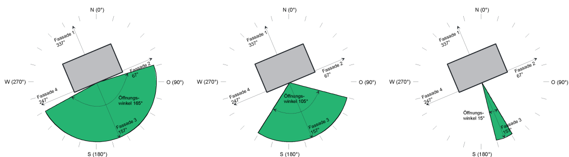
Bild 18: Fassadenausrichtung
