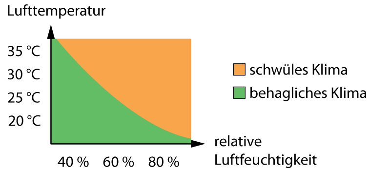
Bild 24: Schwüle - Kennlinie
