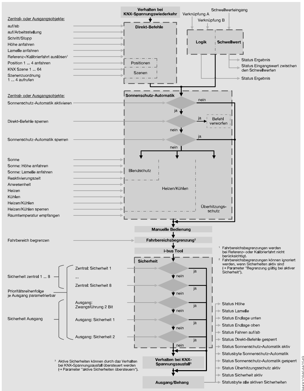
Abb. 5: Funktionsdiagramm JRA/S
