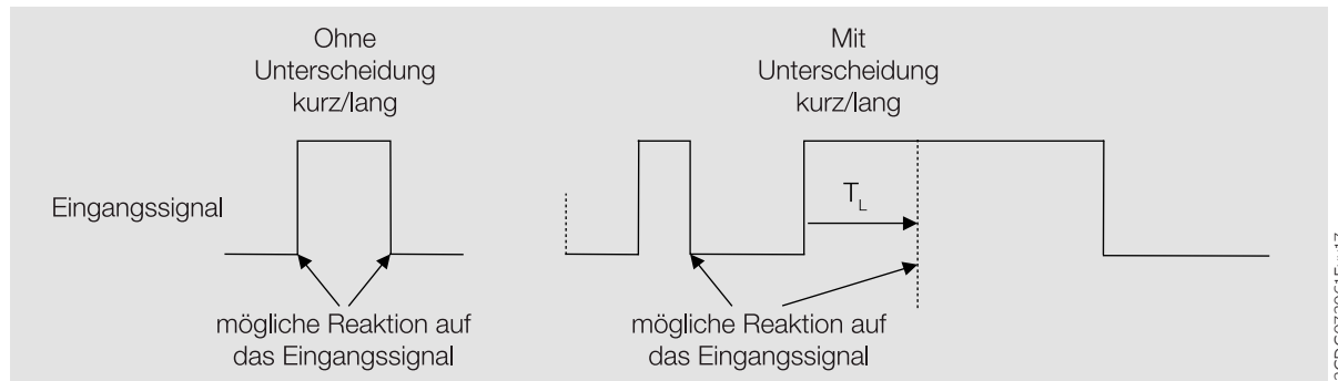
Abb. 5: Unterscheidung kurze/lange Betätigung
