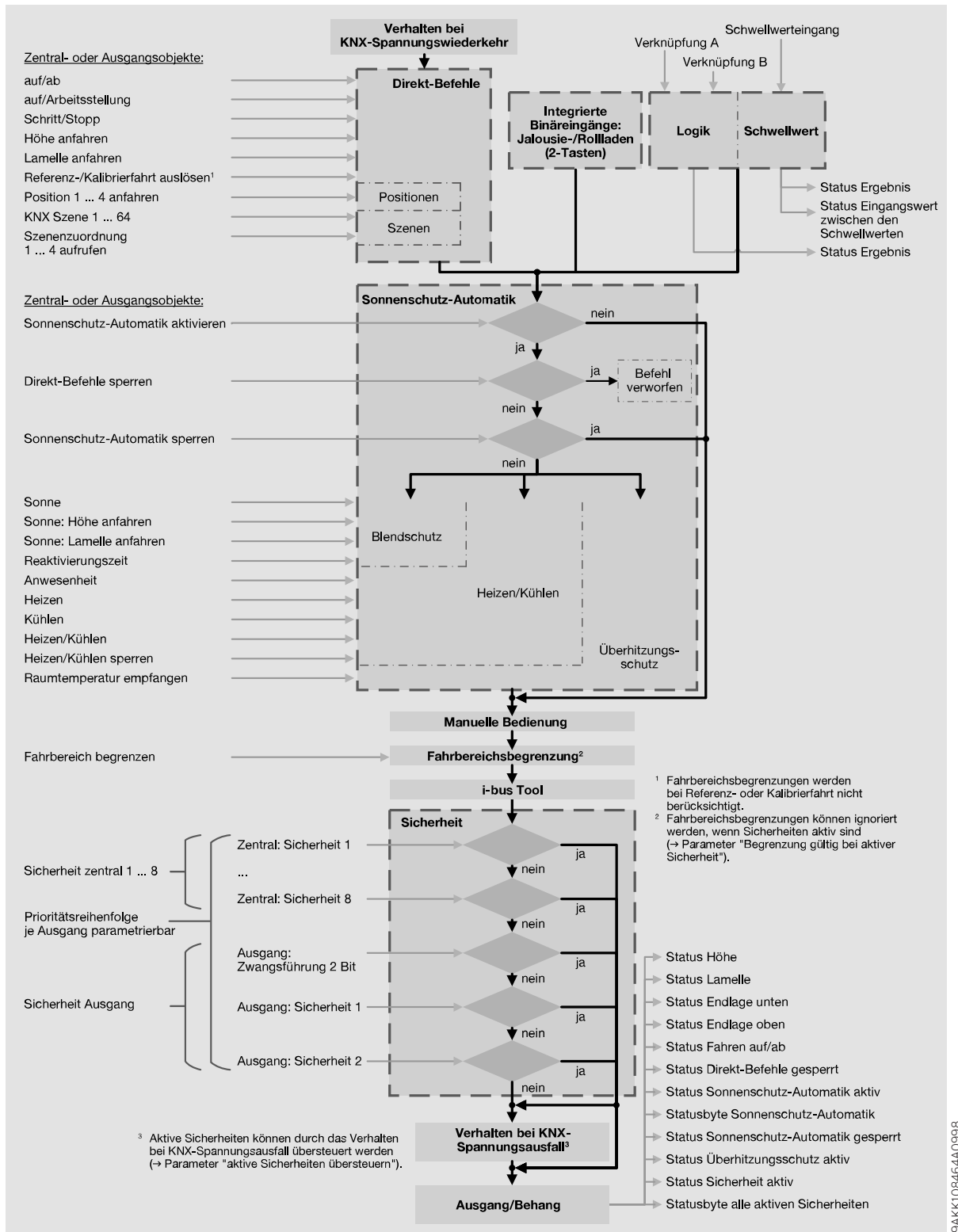
Abb. 4: Funktionsdiagramm JRA/S x.x.4.x, x.x.7.x
