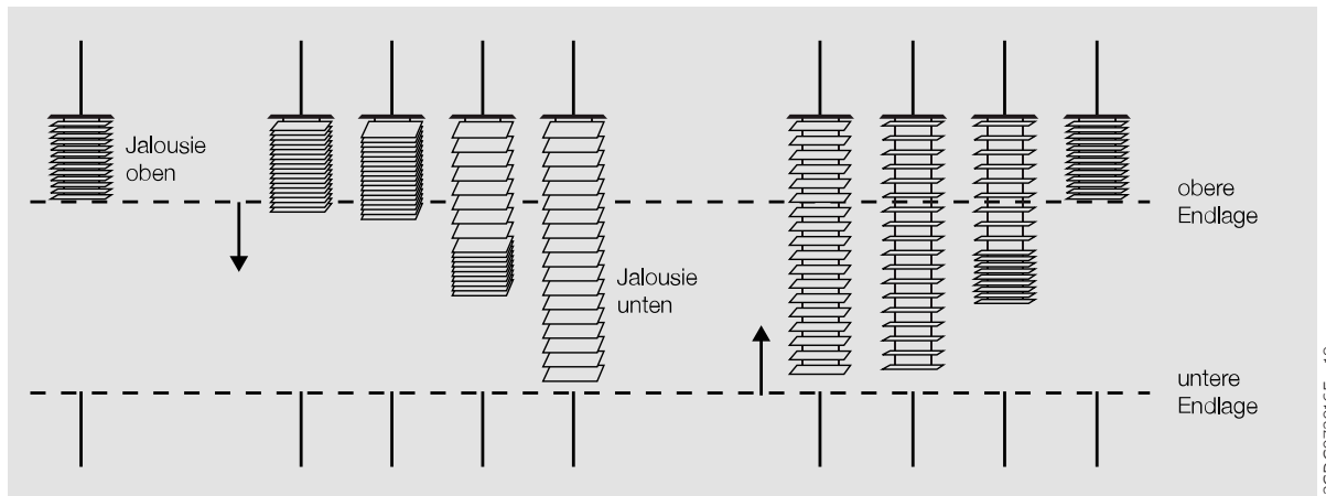
Abb. 26: Behangsteuerung mit Lamellenverstellung
