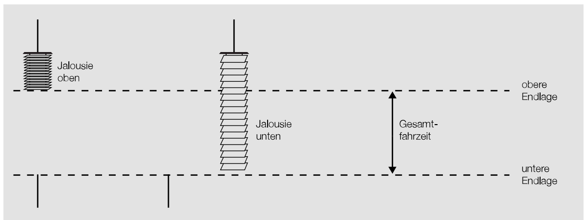
Abb. 25: Funktionsdiagramm Fahrzeiten
