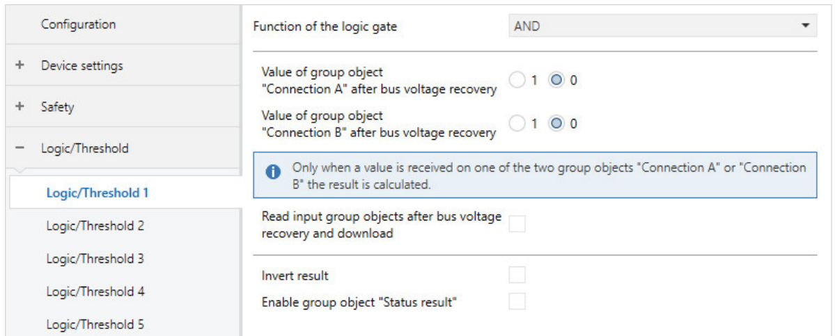
Fig. 25: Parameter window Logic/Threshold 1
