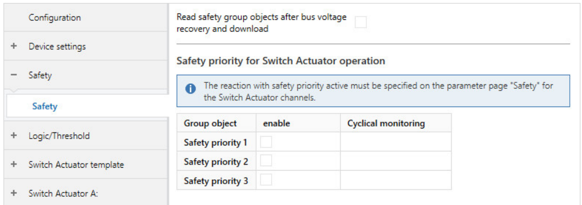
Fig. 24: Parameter window Safety
