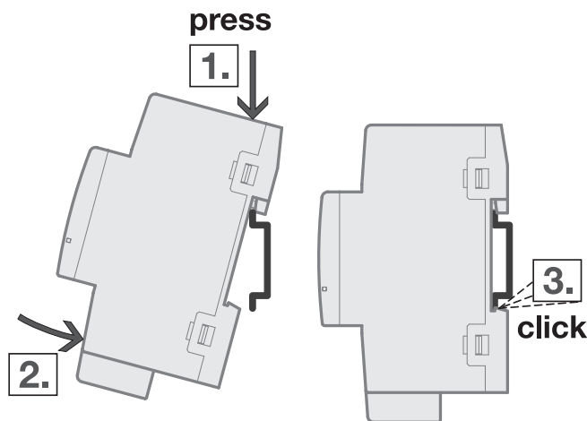
Abb. 21: Montage auf der Tragschiene
