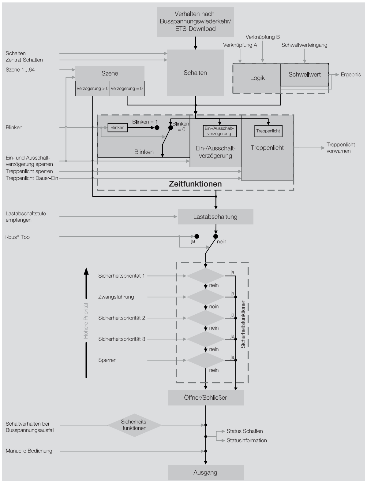
Abb. 13: Funktionsschaltbild Schaltaktor
