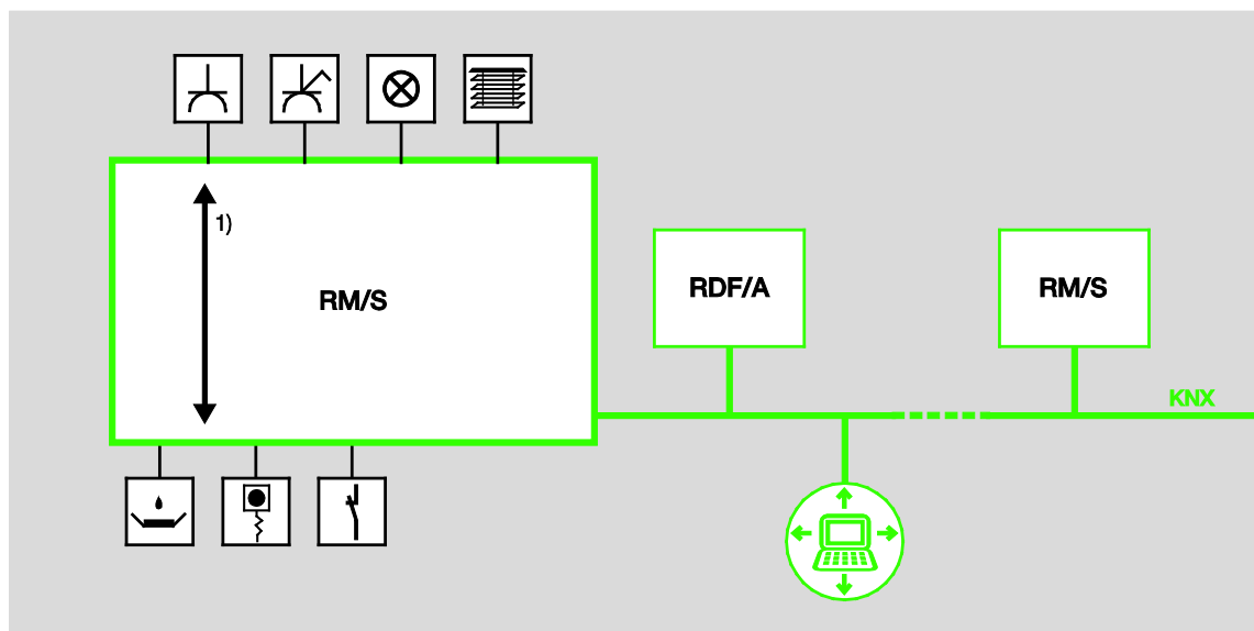
1 Interne Geräteverbindungen
