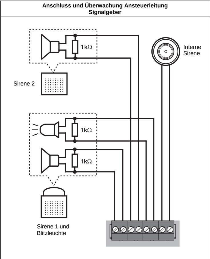
Anschlussbild Signalgeber
