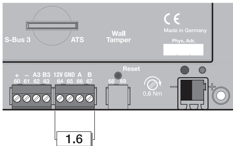
Anschlussbild ATS-Bus
