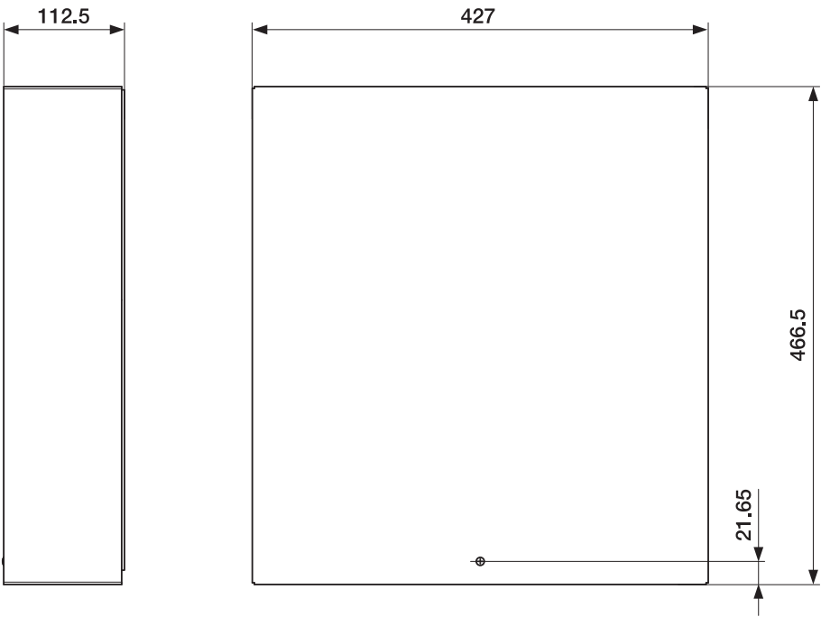
Maßbild Gehäuseoberteil
