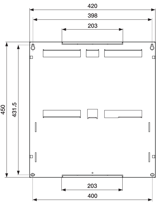
Maßbild Gehäuseunterteil
