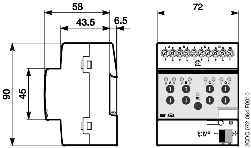
Maßbild JRA/S 4.24.5.1
