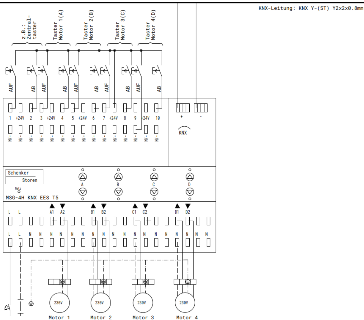
Abbildung 4: Anschlussschema MSG-4H KNX EES T5
