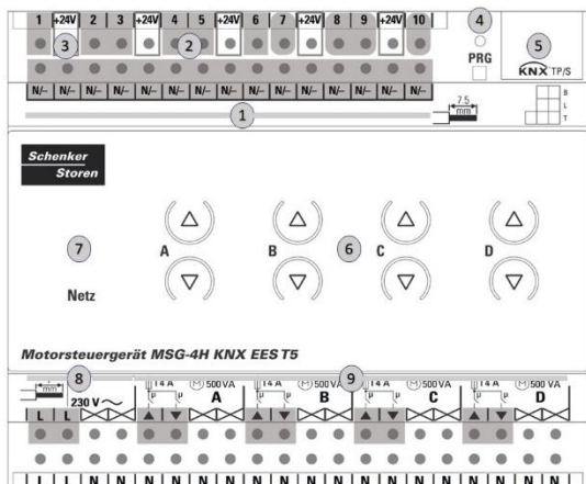
Abbildung 2:Aufbau
