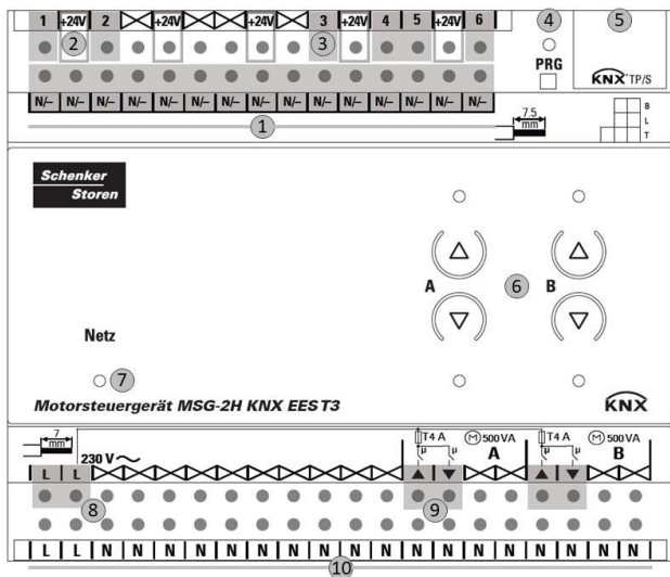
Abbildung 2:Aufbau
