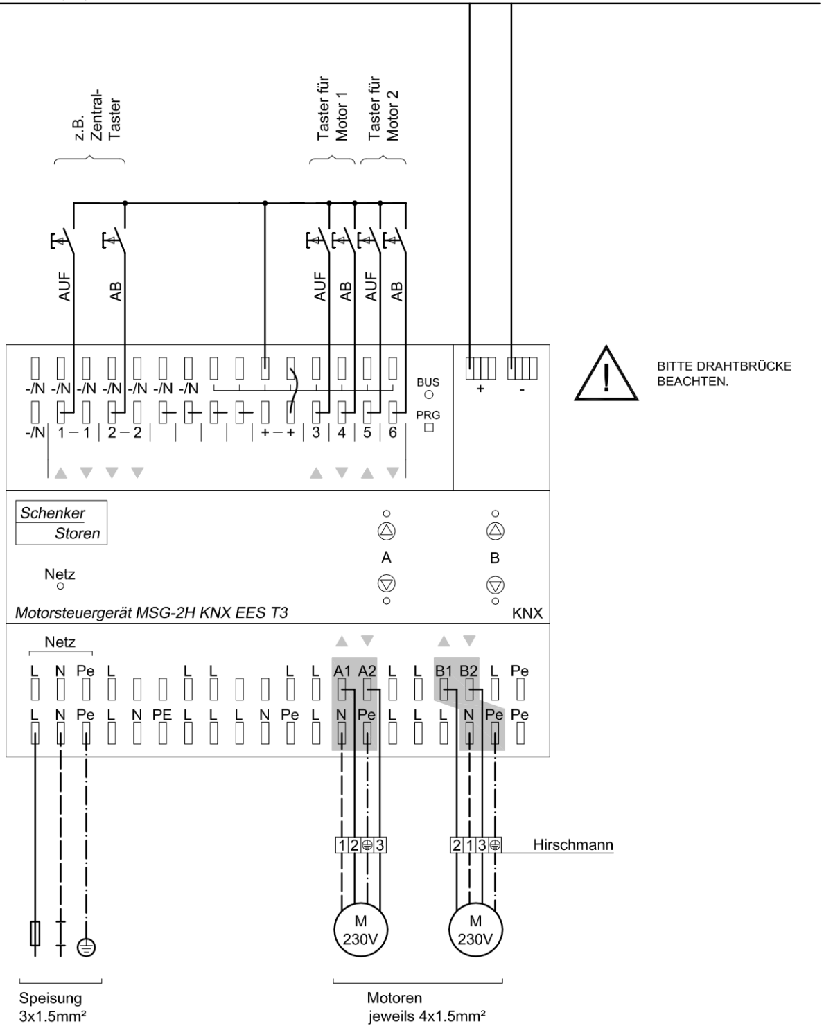
Abbildung 4: Anschlussschema MSG-2H KNX EES T3
