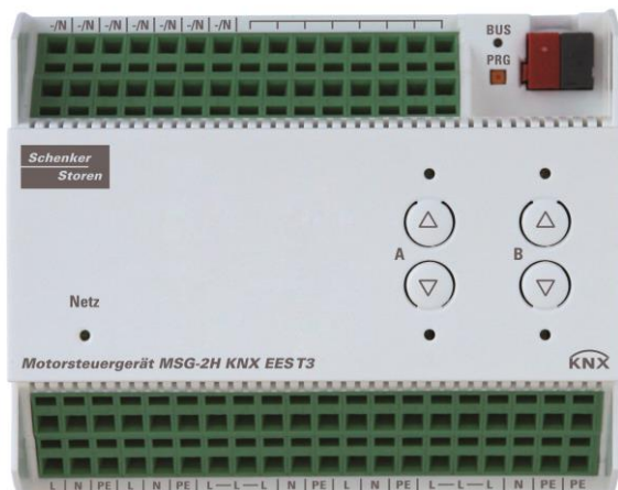
Abbildung 1: KNX - Aktor MSG-2H KNX EES T3
