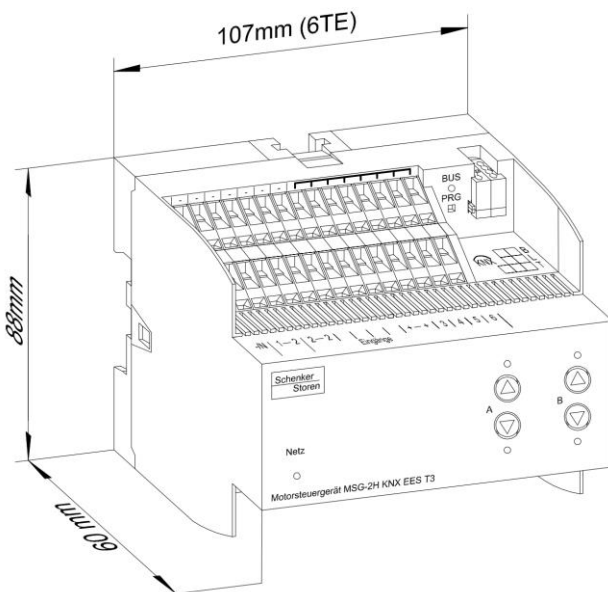
Abbildung 3: Einbaugröße MSG-2H KNX EES T3
