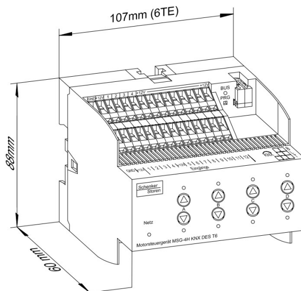
Abbildung 3: Einbaugröße MSG-4H KNX DES T6
