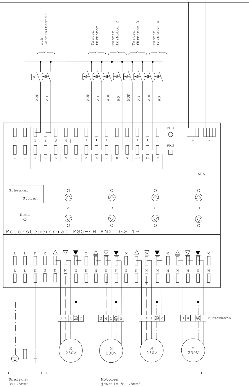
Abbildung 4: Anschlussschema MSG-4H KNX DES T6
