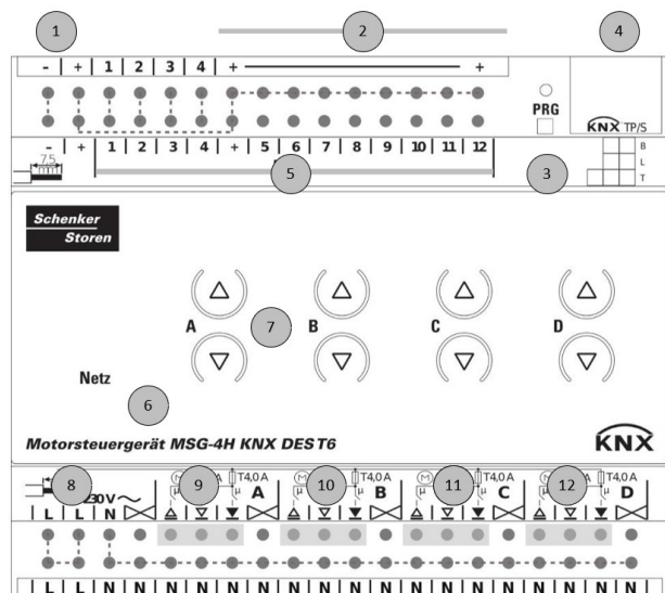
Abbildung 2: Aufbau MSG-4H KNX DES T6
