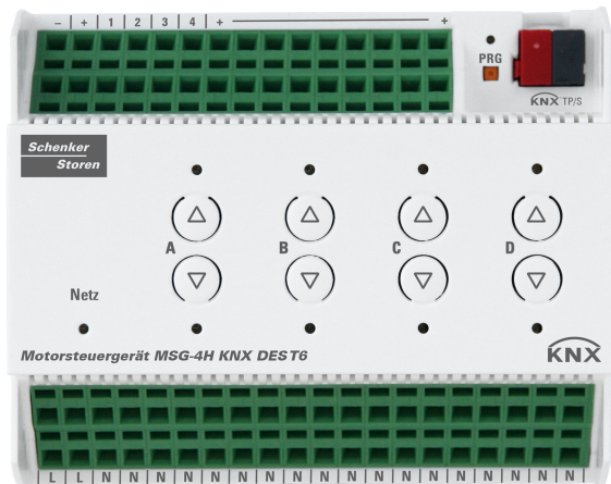
Abbildung 1: KNX - Aktor MSG-4H KNX DES T6
