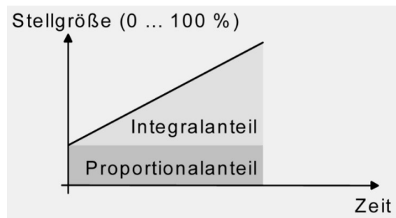
Abbildung 31: PI-Regler
