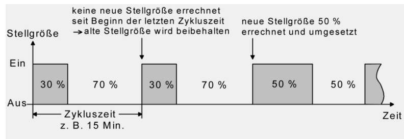
Abbildung 32: PI mit PWM Ausgang
