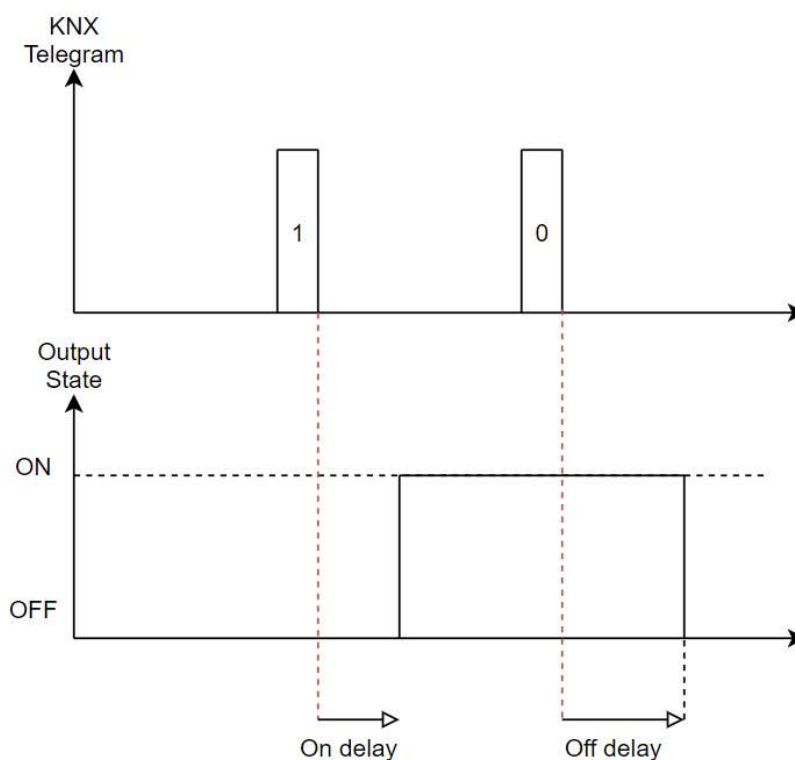
Figure 7 On&amp;Off delay
